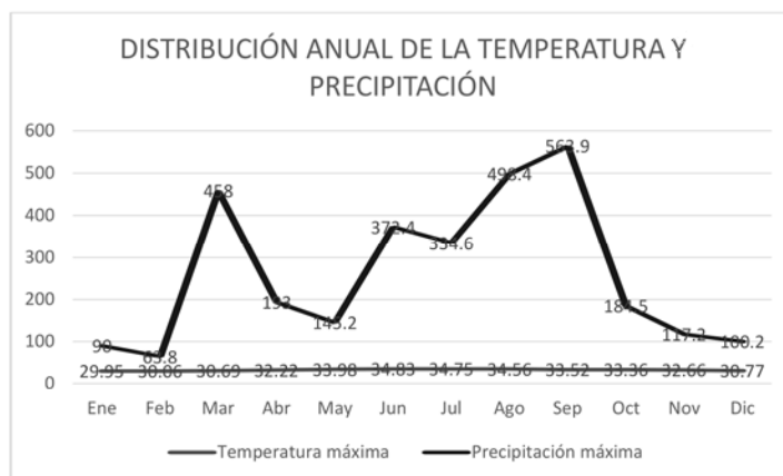
Fig. IV.32 Distribución anual de la temperatura y precipitación mensual en el área del proyecto.
