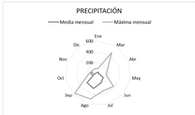
Fig. IV.31 Precipitación mensual en el área del proyecto
