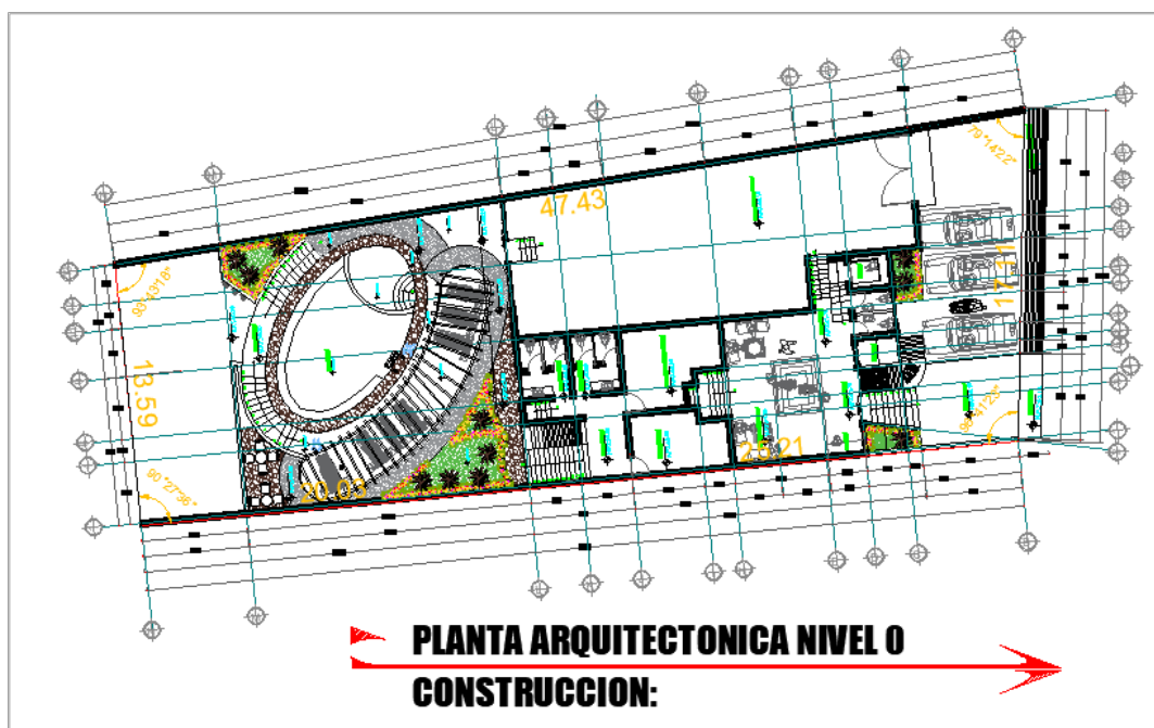
Imagen II.2 Detalle de planta arquitectónica del nivel 0 o planta baja
