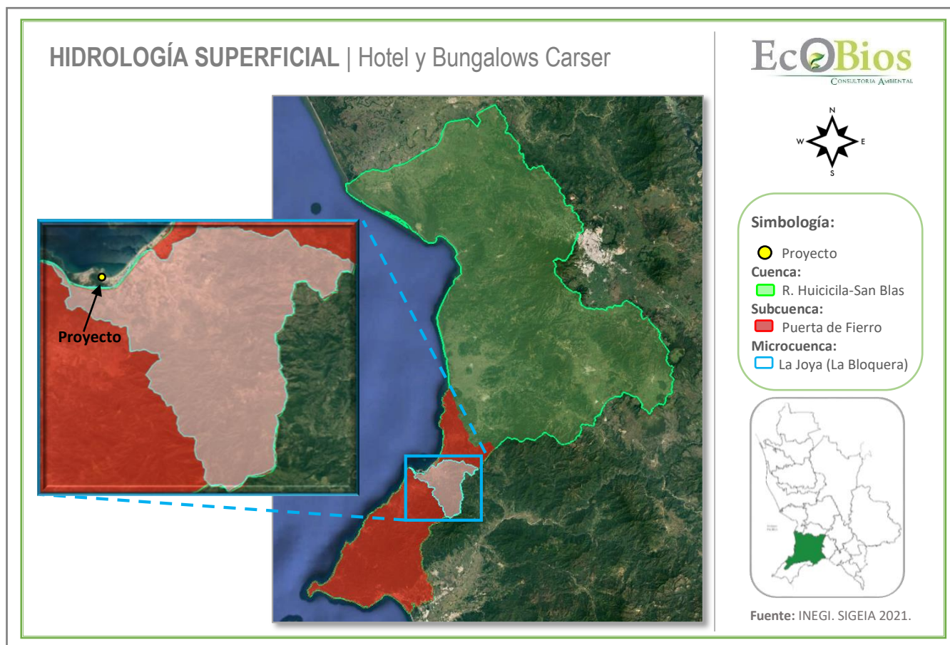
Figura IV.13 Hidrología superficial
