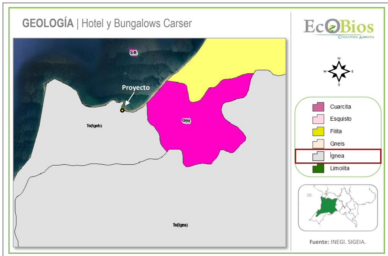
Figura IV.8 Geología del área del proyecto
