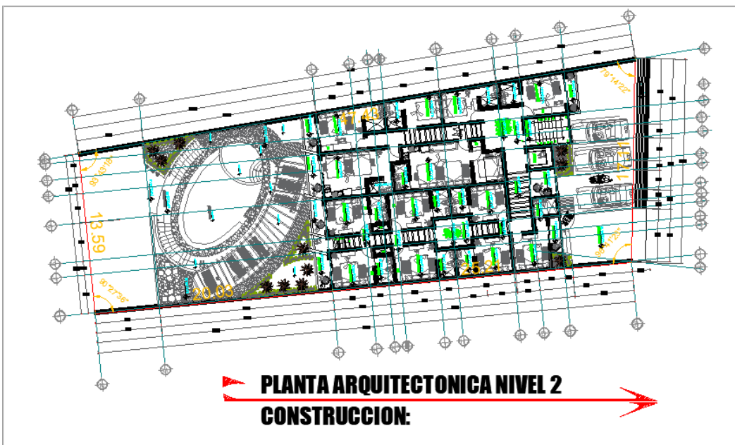
Imagen II.4 Detalle de planta arquitectónica del nivel 2 al 6
