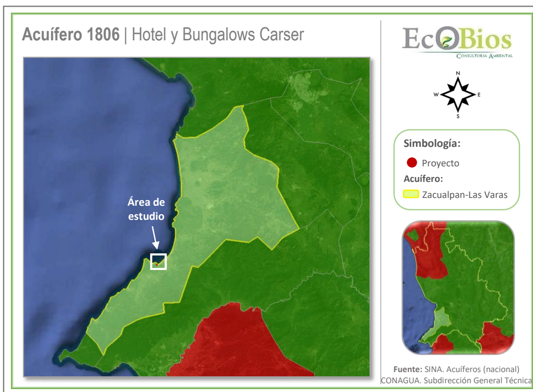
Figura IV.15 Ubicación del proyecto respecto al Acuífero 1806
