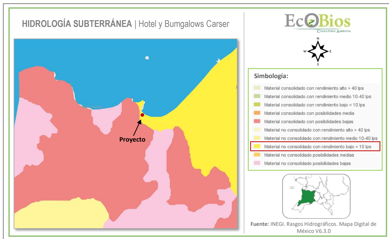
Figura IV.16 Hidrología Subterránea del área del proyecto
