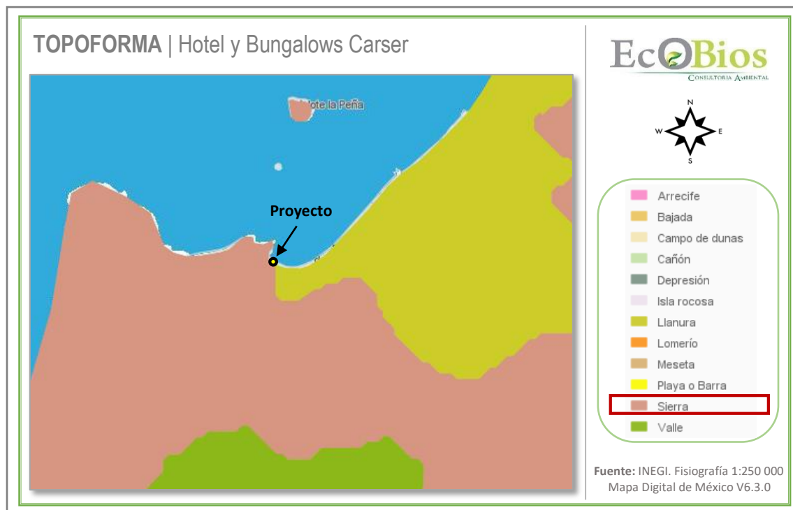
Figura IV.10 Topoforma en la que se encuentra el área del proyecto
