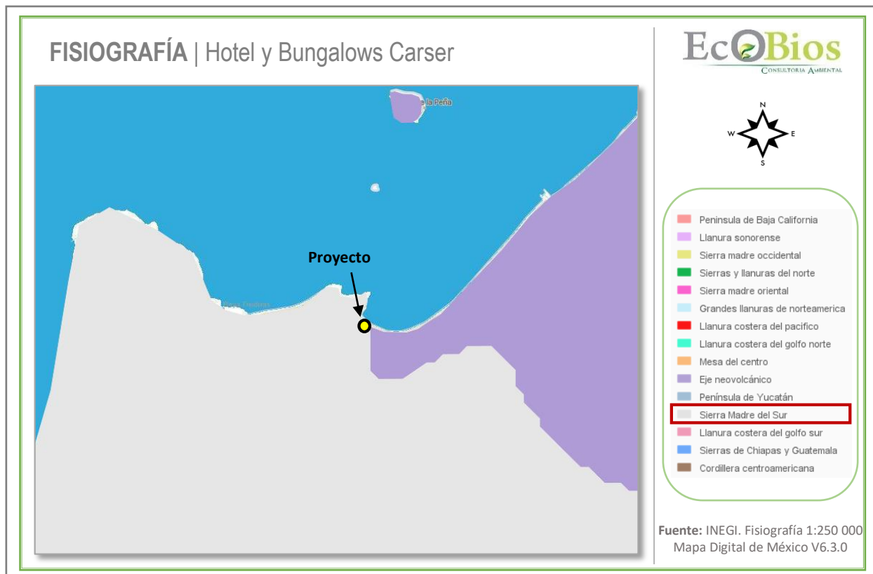
Figura IV.9 Fisiografía del área del proyecto
