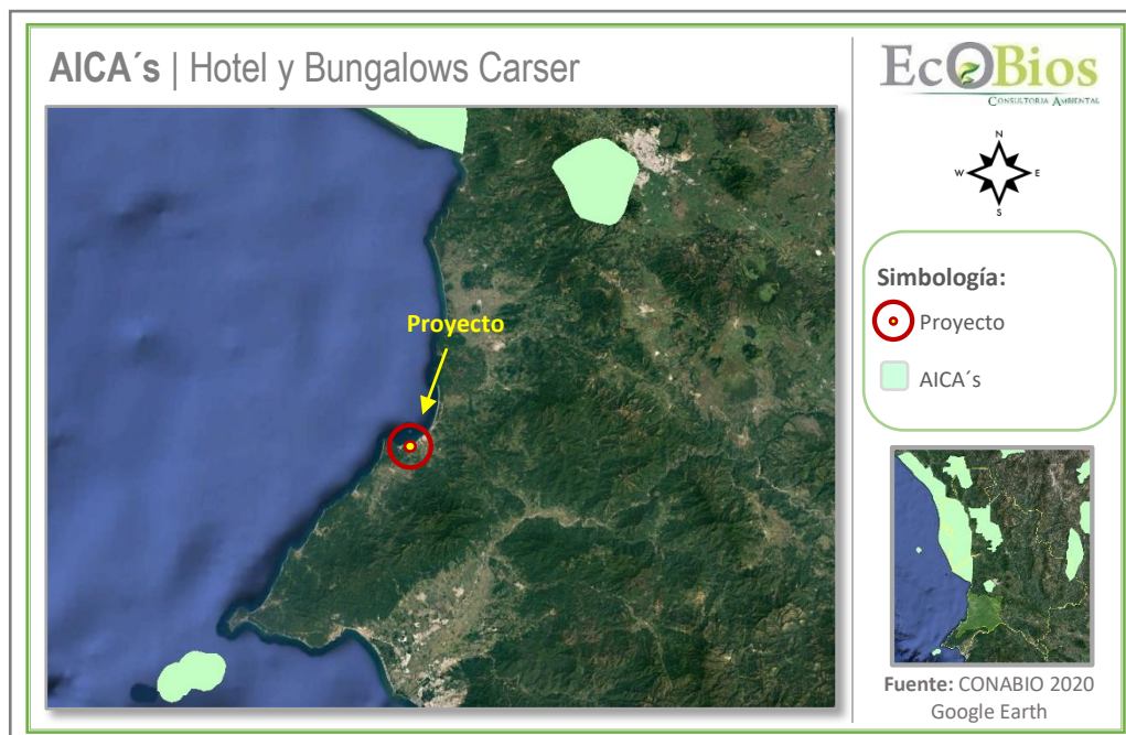
Figura III.5 AICA's de mayor proximidad al polígono del proyecto
