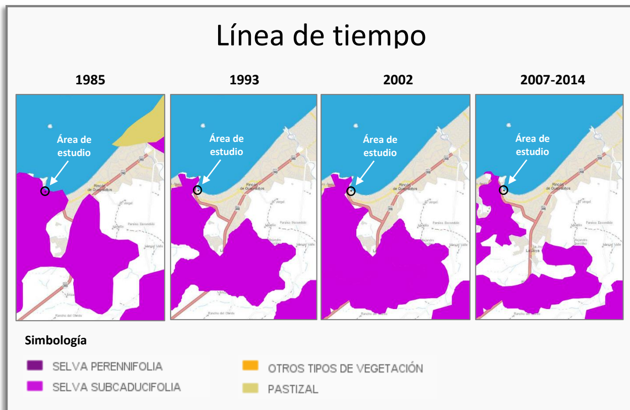
Imagen II.1 Línea de tiempo del Uso de suelo y vegetación en el área de estudio. Fuente: INEGI Mapa Digital V6.3
