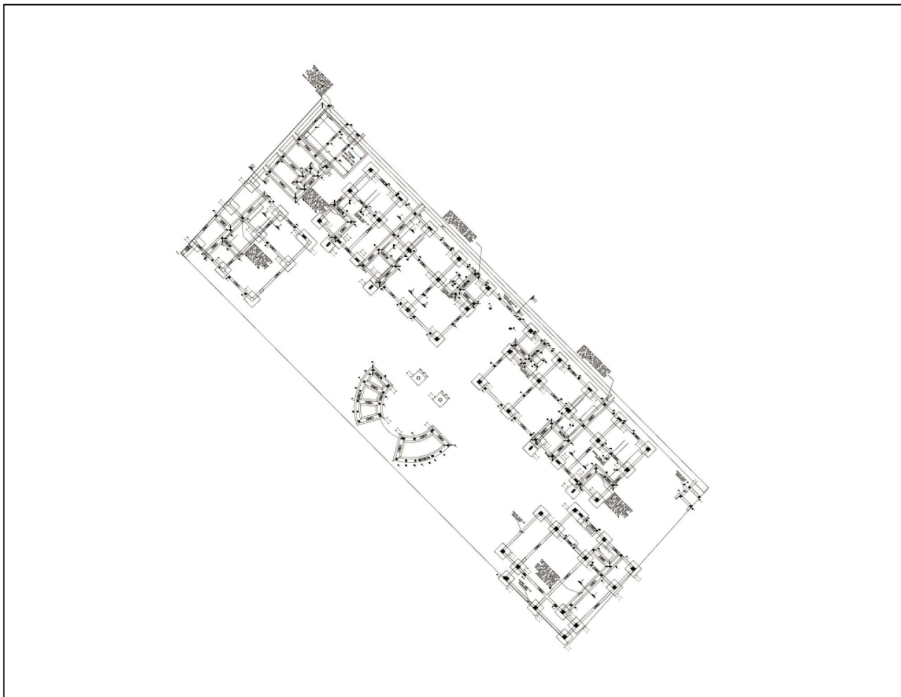
Figura 5 Plano de cimentación considera para el proyecto
