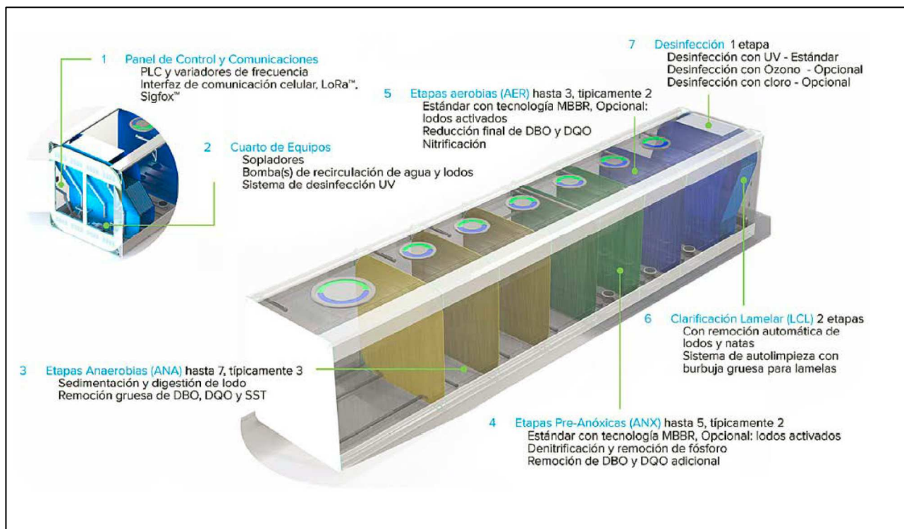
Figura 18 . Partes de Planta de Tratamiento de Aguas Residuales (PTAR)
