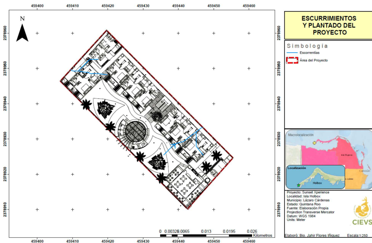
Figura 28 Ubicación de las zapatas aisladas de cimentación con relación a las escorrentías identificadas
