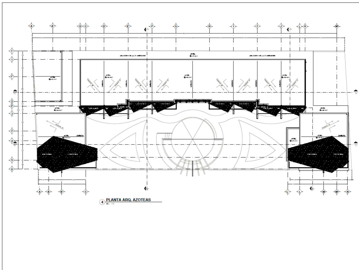
Figura 9. Plano conjunto de la Azotea del Proyecto Sunset Xperience Holbox
