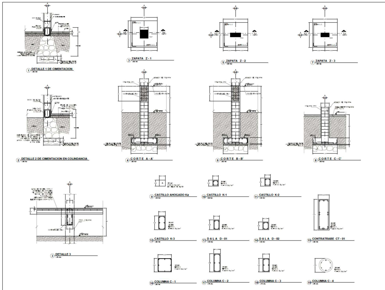
Figura 16 Detalles de castillo, zapatas aisladas, pilotes y columnas
