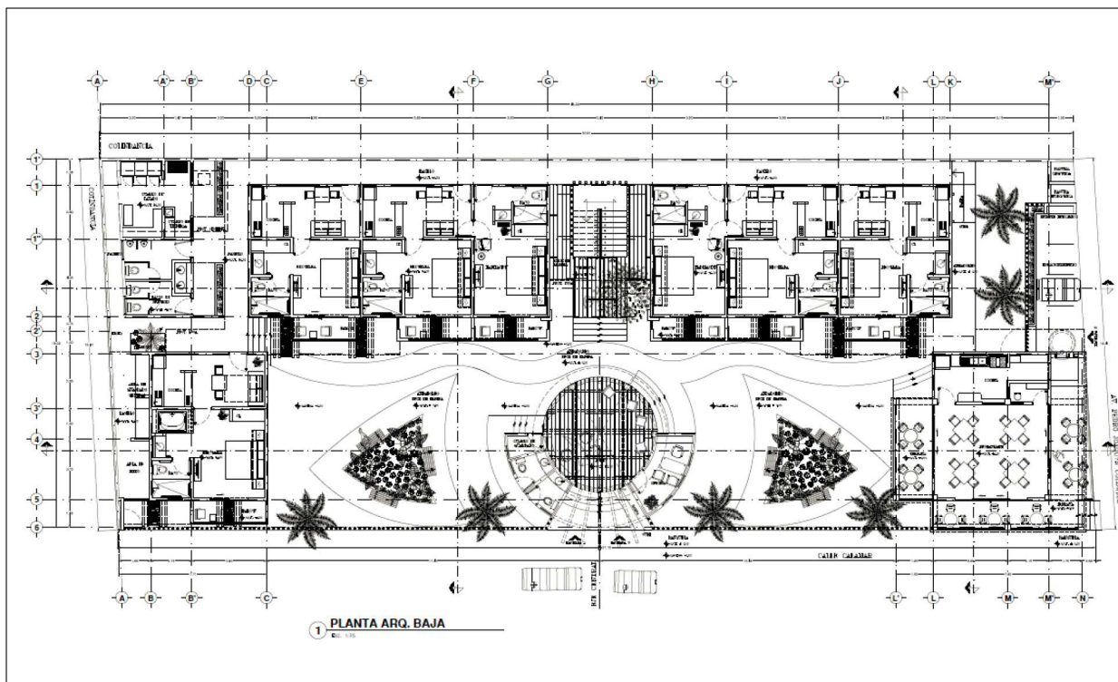
Figura 6 Plano planta baja del Proyecto Sunset Xperience Holbox
