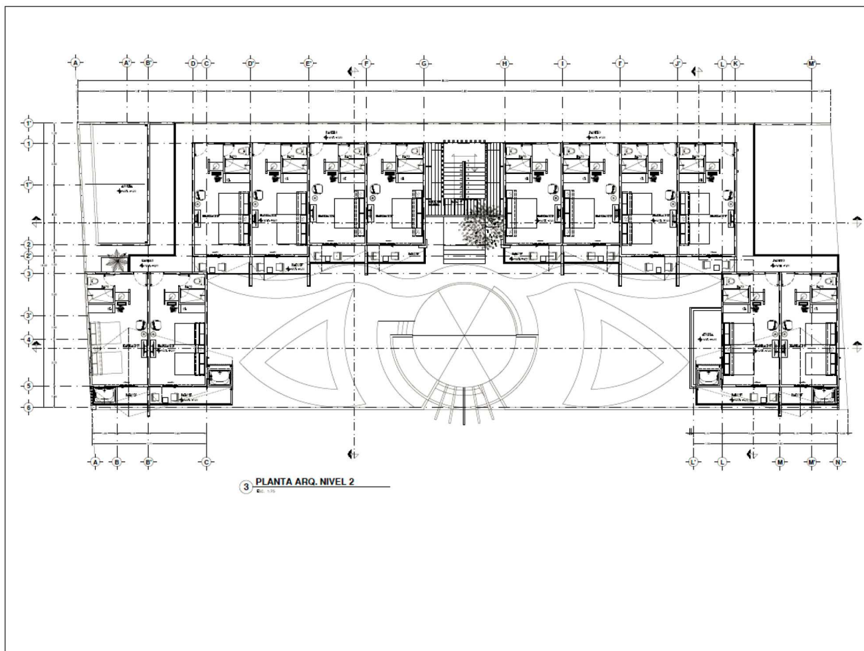
Figura 8 Plano planta nivel 2 del Proyecto Sunset Xperience Holbox
