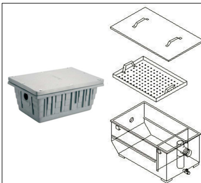
Figura 17 . Diseño de las trampas de grasas consideradas para instalar en cada uno de los lavaderos del proyecto.
