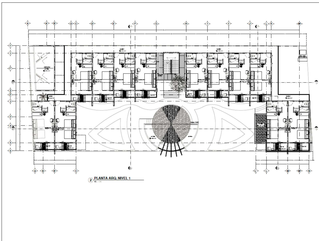
Figura 7 Plano planta nivel 1 del Proyecto Sunset Xperience Holbox
