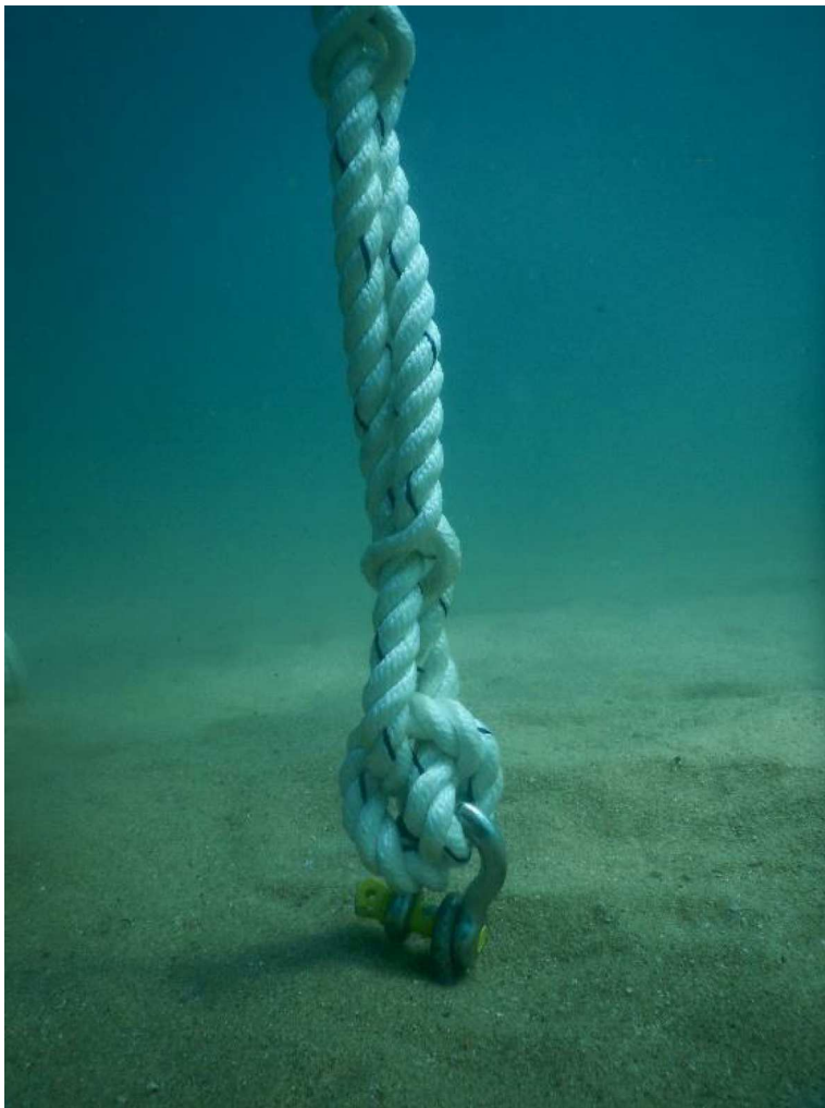
Figura 5.- Vista final de un anclaje manta raya, solo se ve el grillete de fijación.
