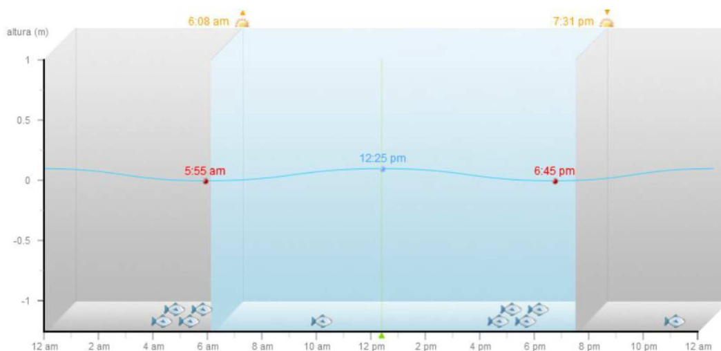
Figura 14.-Gráfico de pleamares y bajamares, donde se observa la primera bajamar fue a las 5:55 am y la siguiente bajamar será a las 6:45 pm.
