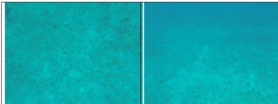
Figura 27.- zona de arenal.
