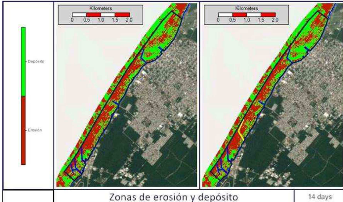
Figura 19.- Zonas de erosión y depósito dentro de la zona marina.
