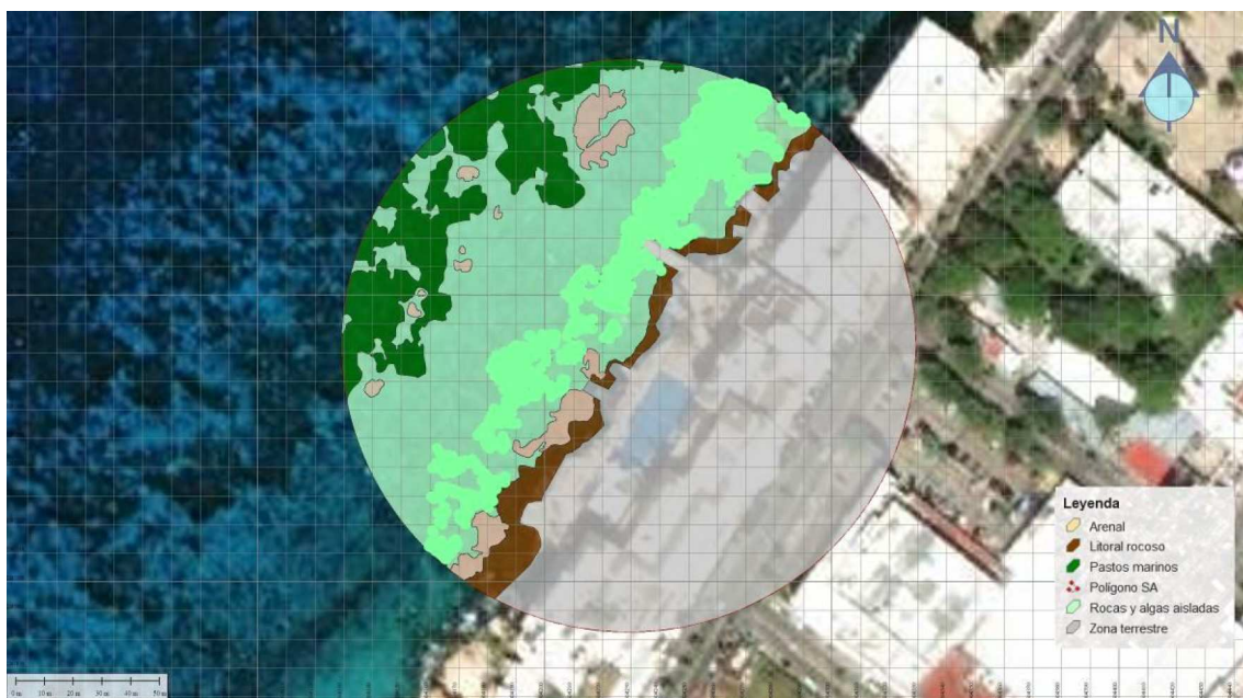
Figura 25.- Resultado de la fotointerpretación realizada y comprobada en campo.
