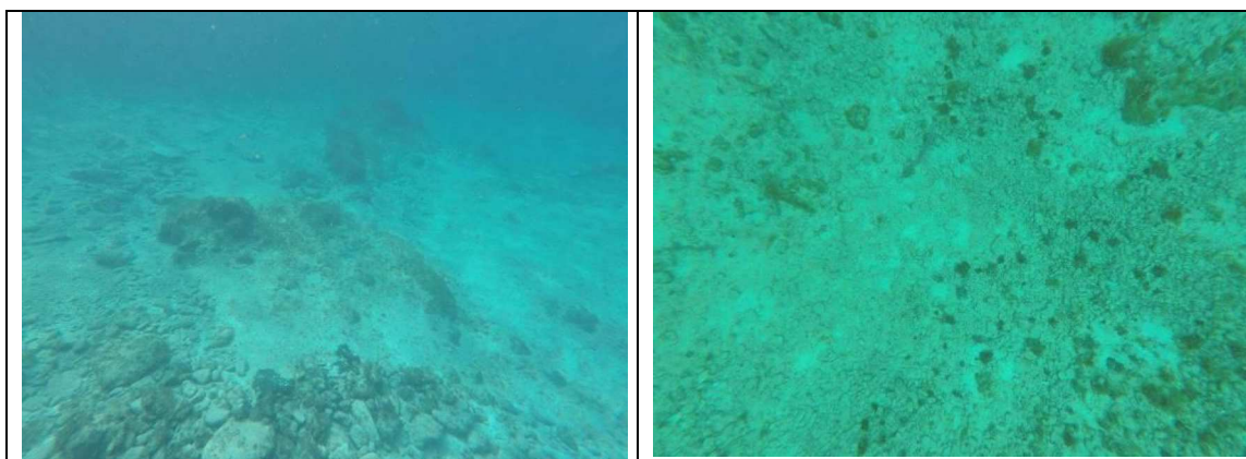
Figura 29.- Tipo de suelo conformado por sustrato arenoso y roca suelta y algas aisladas en la zona de influencia del proyecto.
