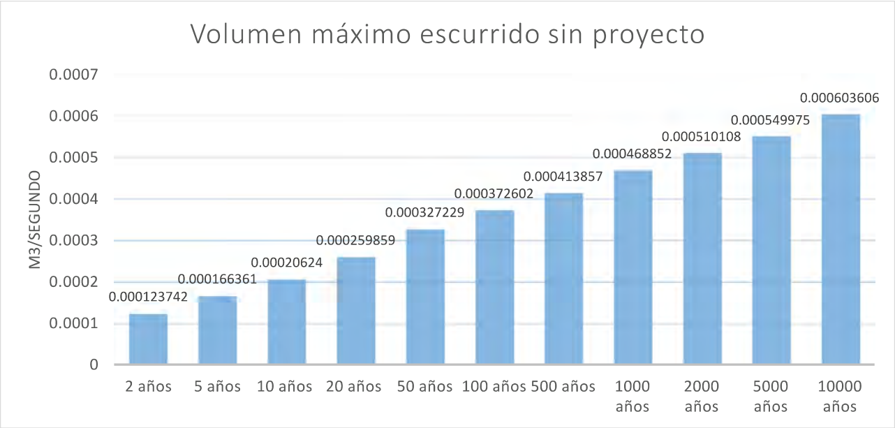
Figura 38 Grafica de volumen máximo escurrido sin proyecto
