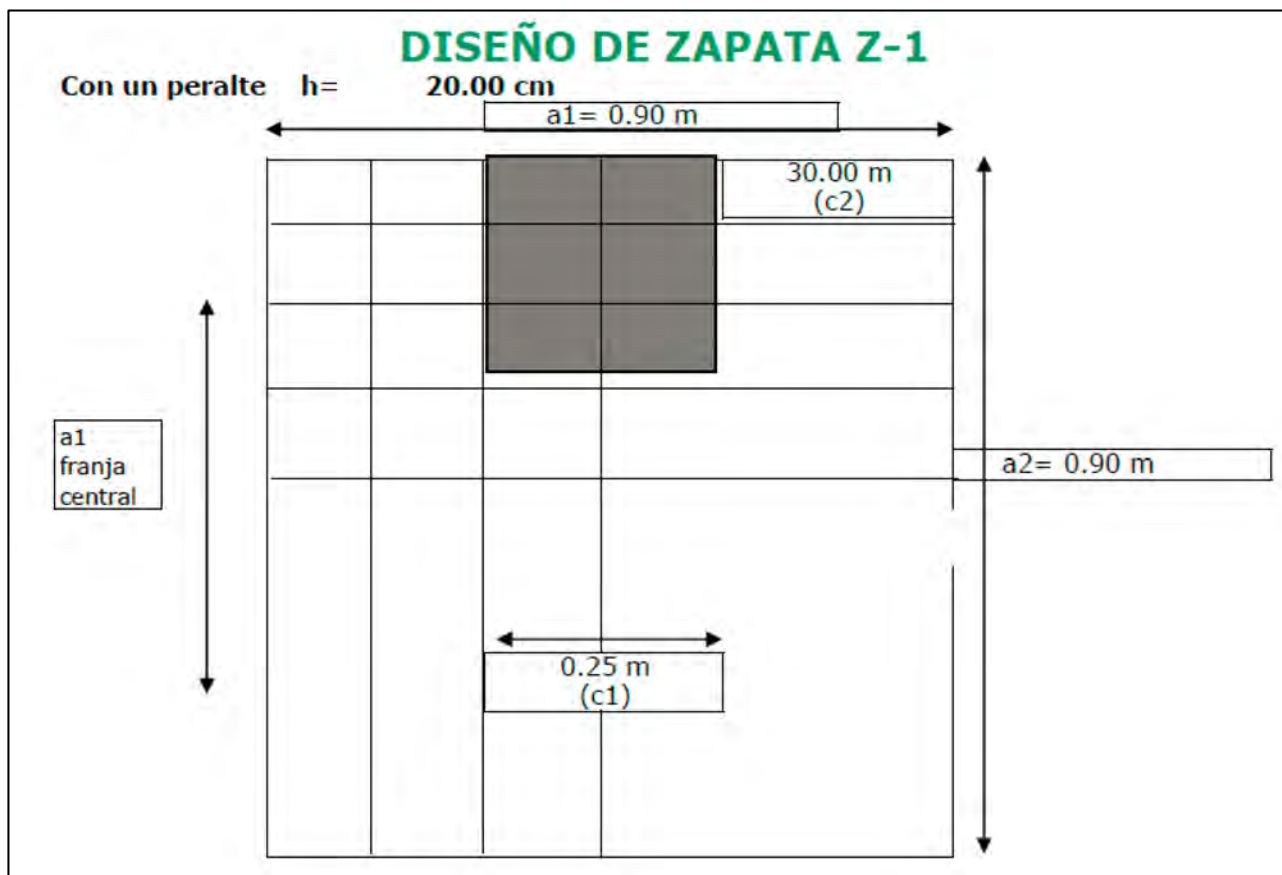
Figura 4 Detalles de zapata
