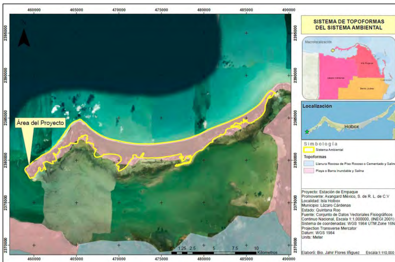
Figura 21 Topoformas del Sistema Ambiental
