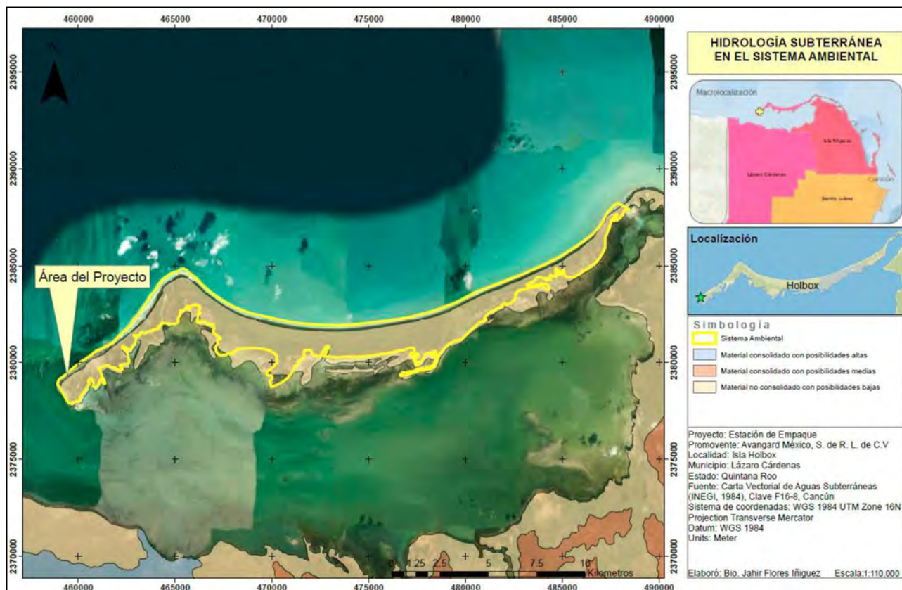
Figura 18 Mapa de la hidrología subterránea del Sistema Ambiental
