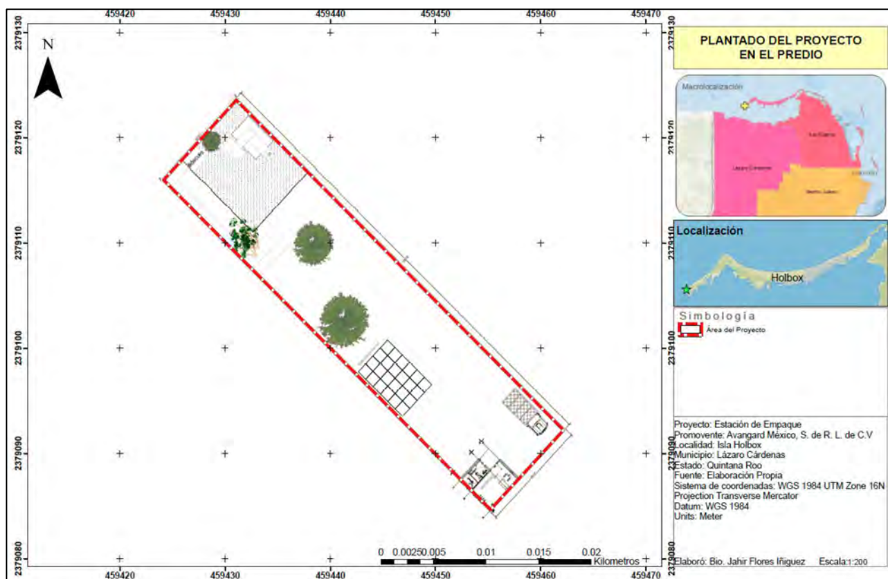
Figura 3 . Huella de desplante del proyecto sobre la superficie del terreno
