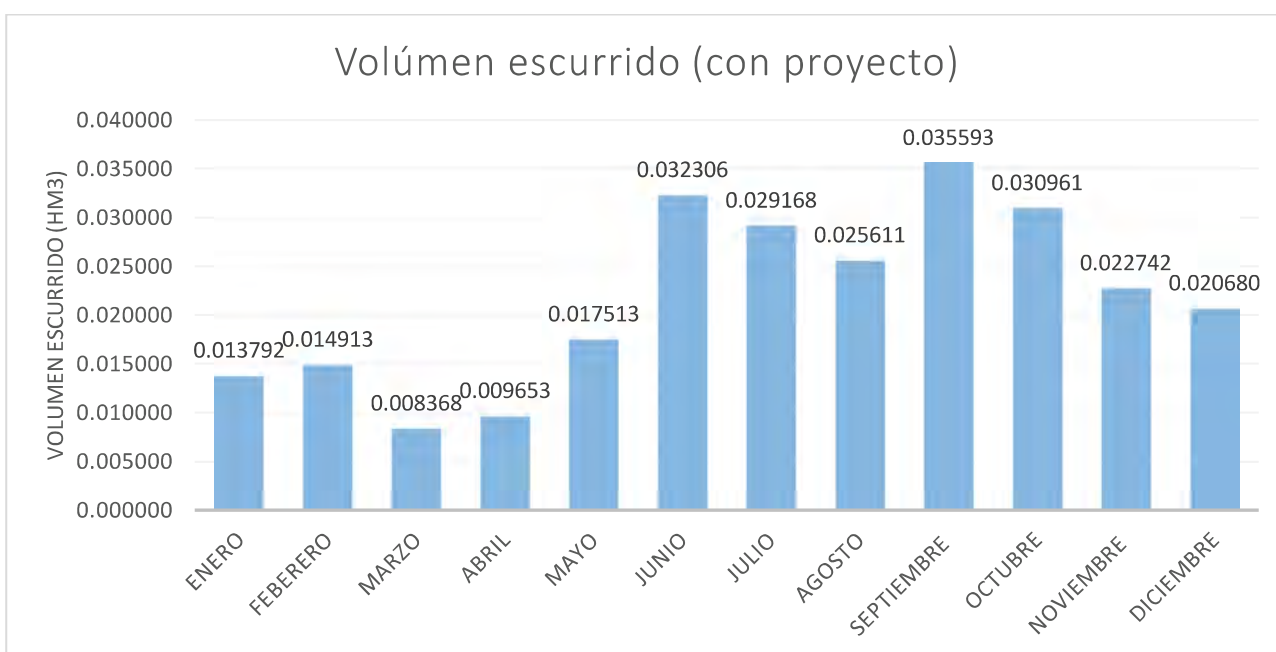
Figura 37 Grafica de volumen medio escurrido con proyecto
