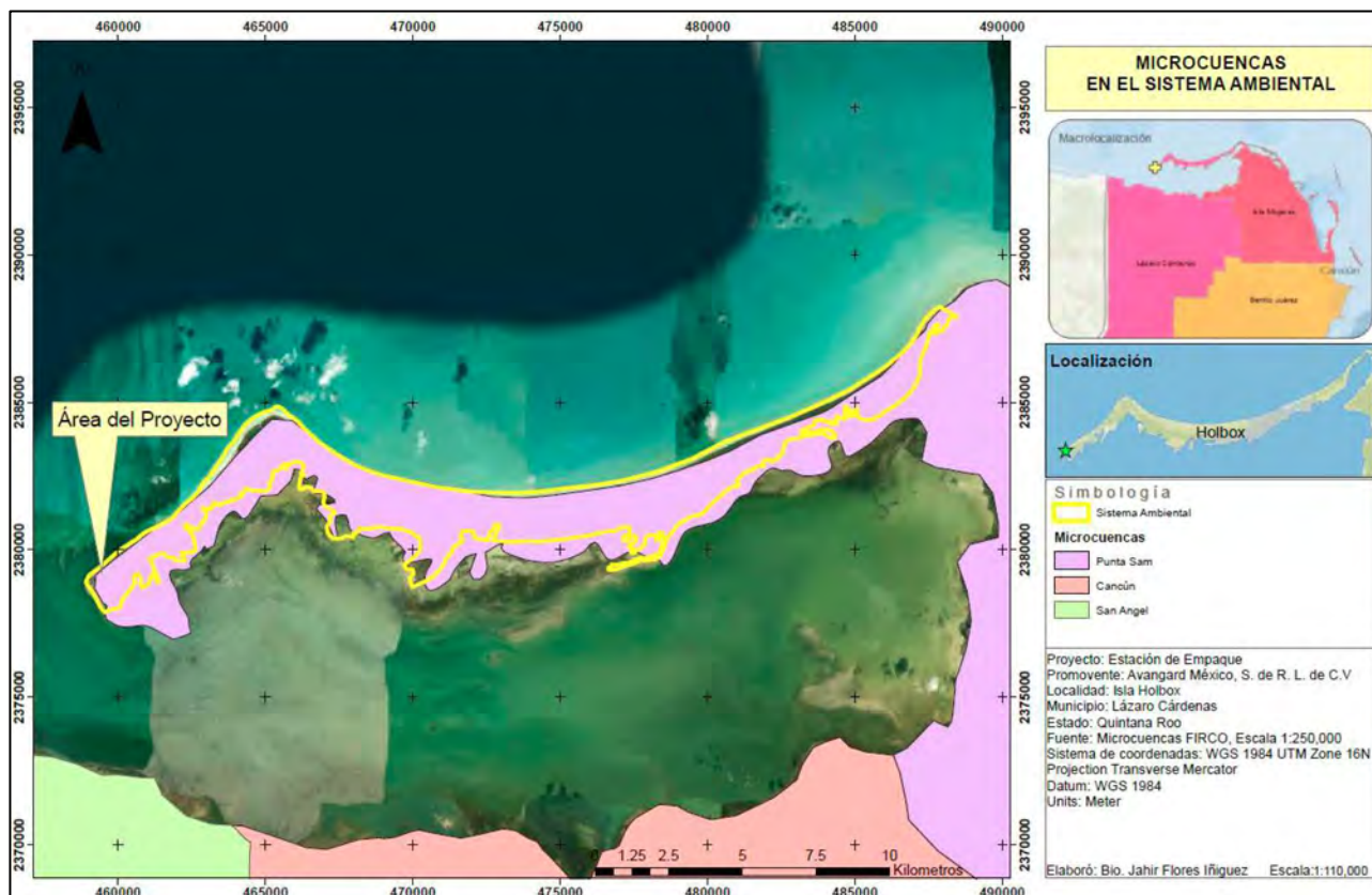
Figura 19 Microcuencas en el Sistema Ambiental
