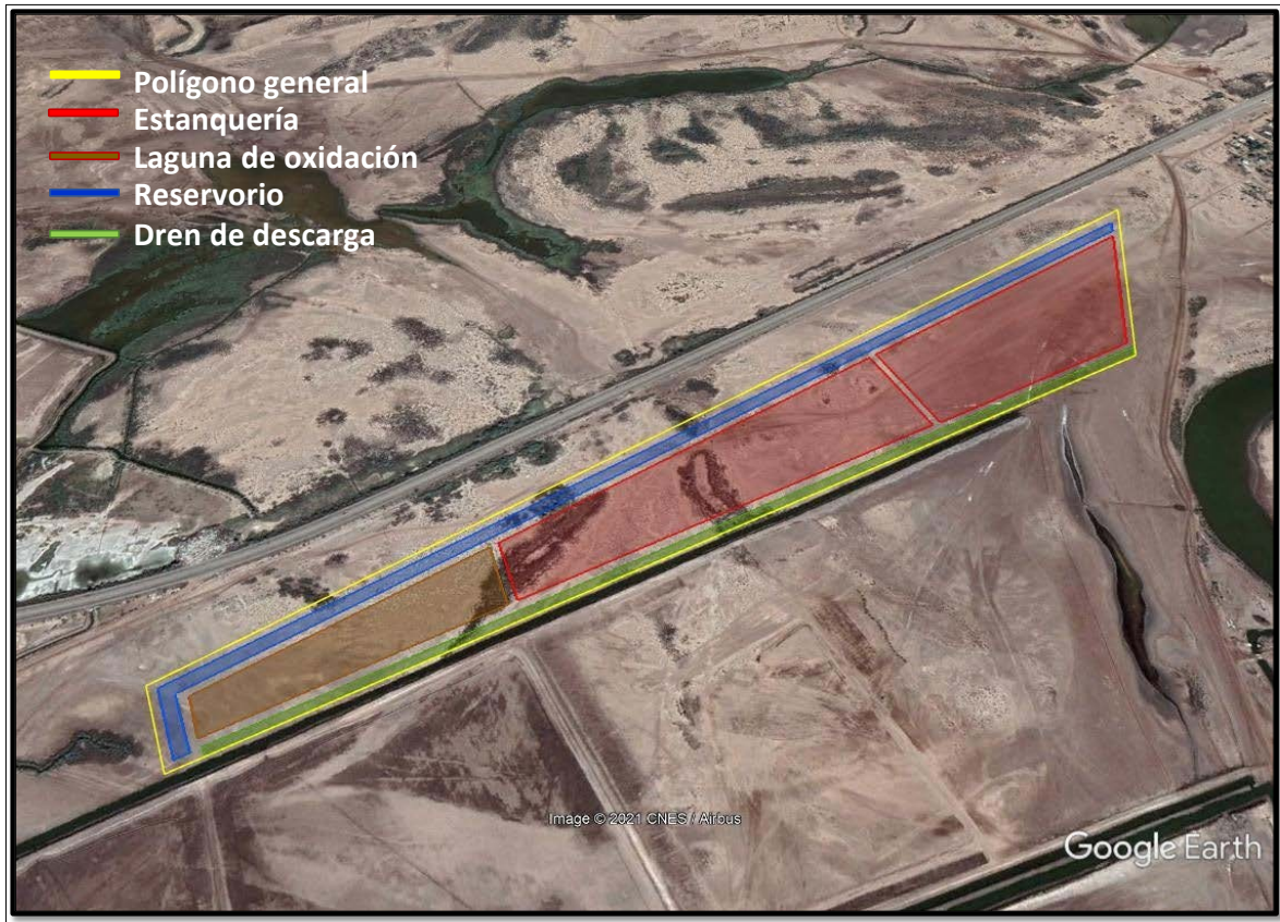
Figura II.1. Distribución de áreas en granja de cultivo de camarón.
