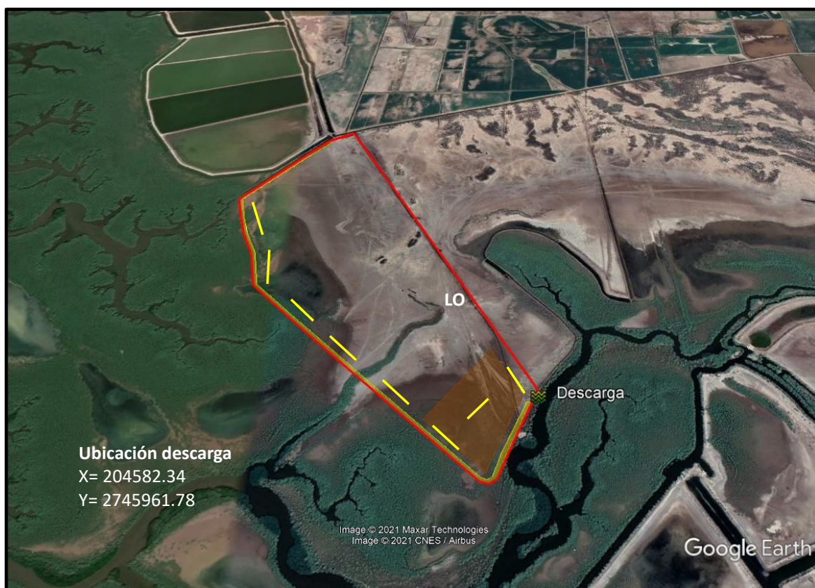
Figura II.6 Dren de descarga con sus flujos y punto de descarga
