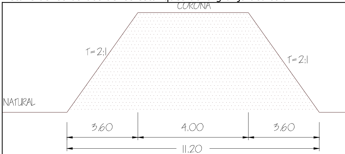
Detalle de los bordos de los estanques de la granja acuícola.
