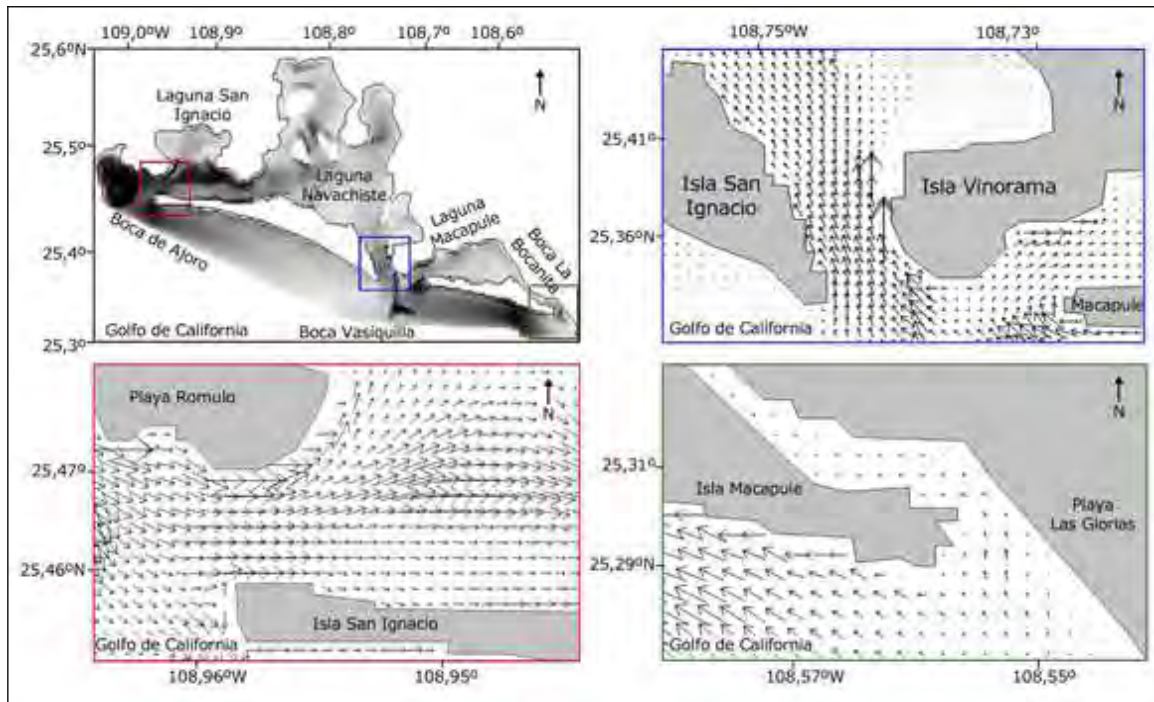
Distribución vectorial de corrientes durante el flujo de la marea, y el forzamiento del viento uniforme de 5 \text{ m s}^{-1} del noroeste
