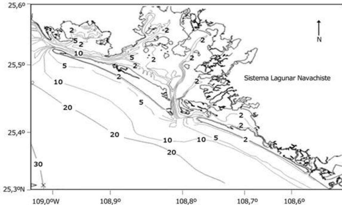
Batimetría de la región correspondiente al Sistema Lagunar Navachiste, y su región oceánica adyacente (profundidad en metros)
