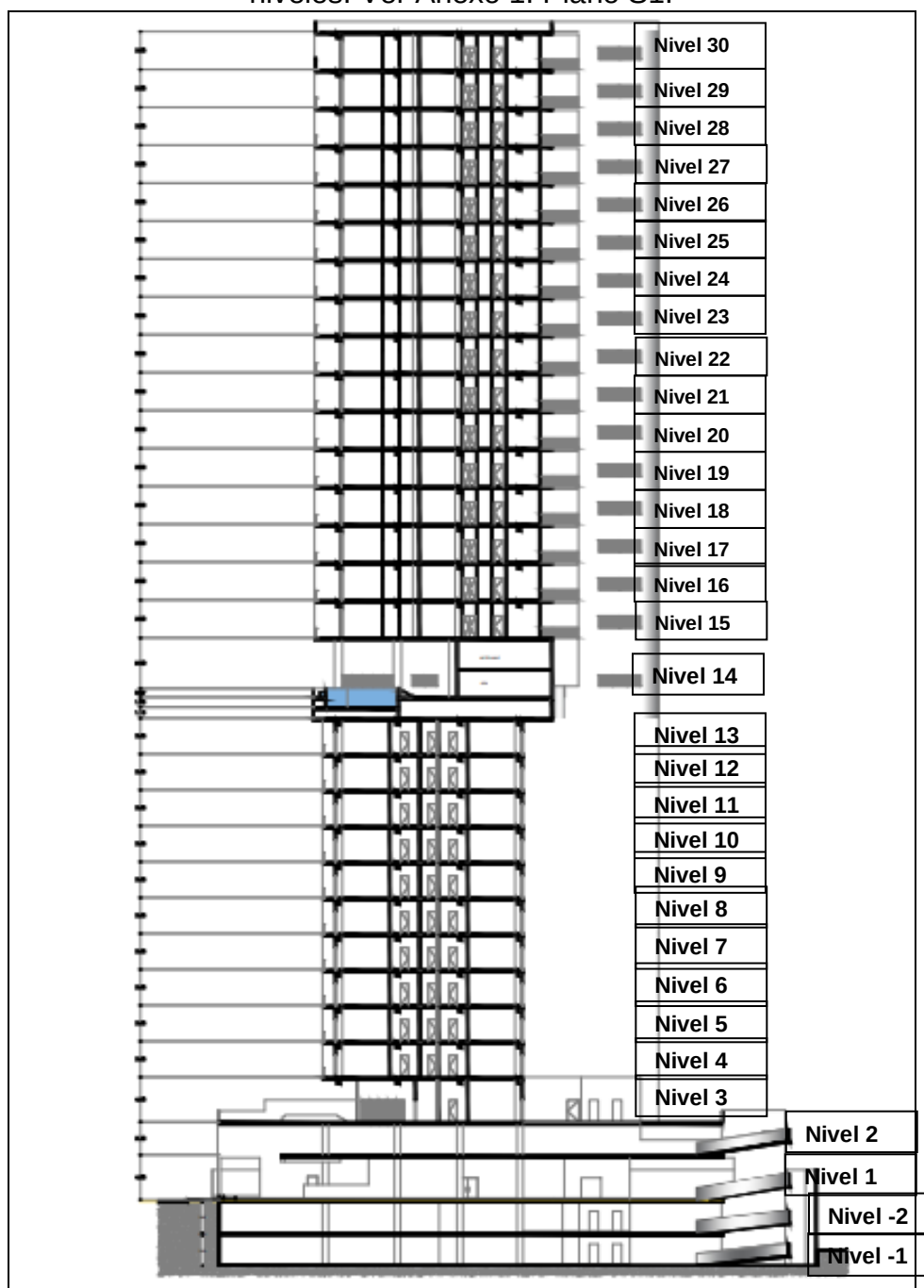
Imagen II.3.- Perfil de la torre condohotel Holiday Inn Express & Suites y sus 32 niveles. Ver Anexo 1. Plano S1.
