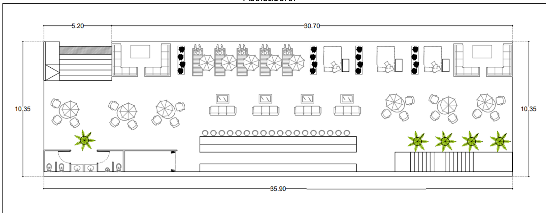
Imagen II.5.- Planta de distribución del asoleadero que se pretende construir en la ZOFEMAT. Ver Anexo 1, Plano 1-Asoleadero.
