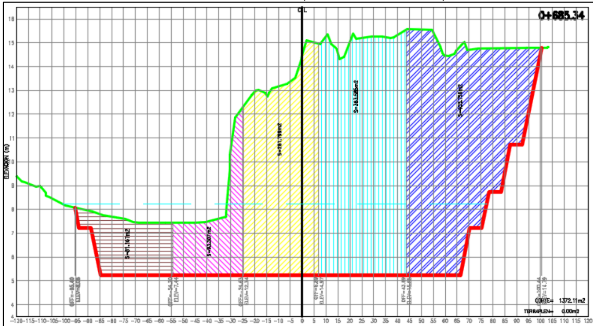
FIGURA 4. ESTACION 0+685.34 (PARTE FINAL DEL PROYECTO):
