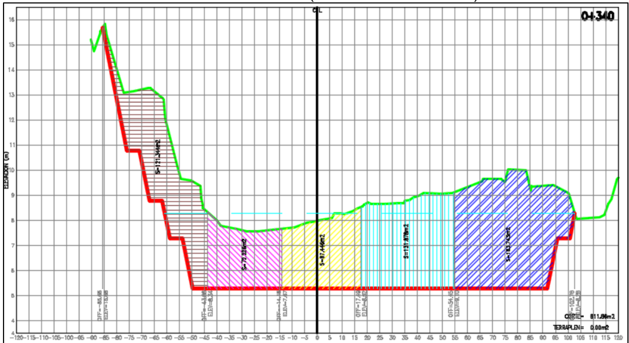
FIGURA 3. ESTACION 0+340.00 (PARTE CENTRAL DEL PROYECTO):
