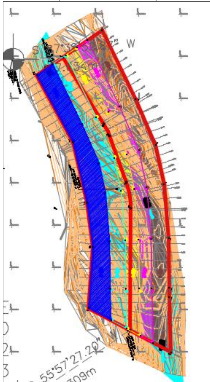
FIGURA 5. 118 FRENTES DE EXTRACCIÓN DIVIDIDOS EN 47 ESTACIONES O SECCIONES. (Plano Planta de extracción)
