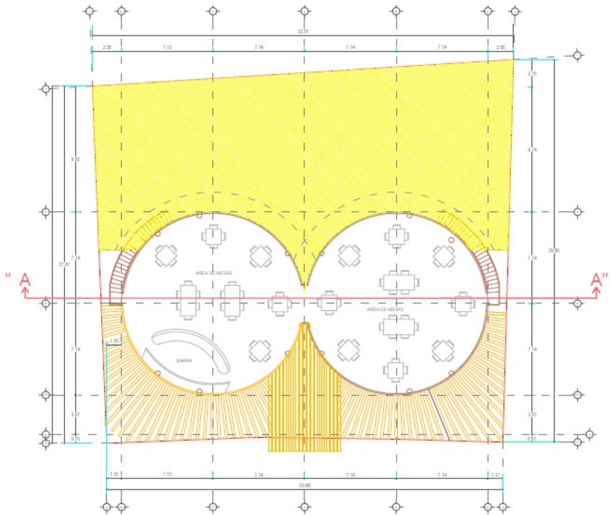
PLANTA ARQUITECTONICA ALTA
