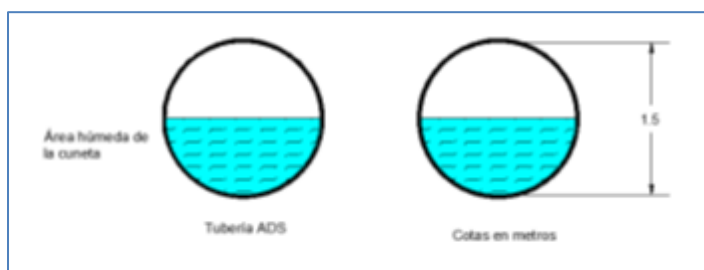
Figura III-25. Caracterización de tubería tipo ADS
