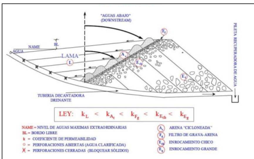
Figura II-15. Método constructivo “aguas abajo” con enrocamiento
