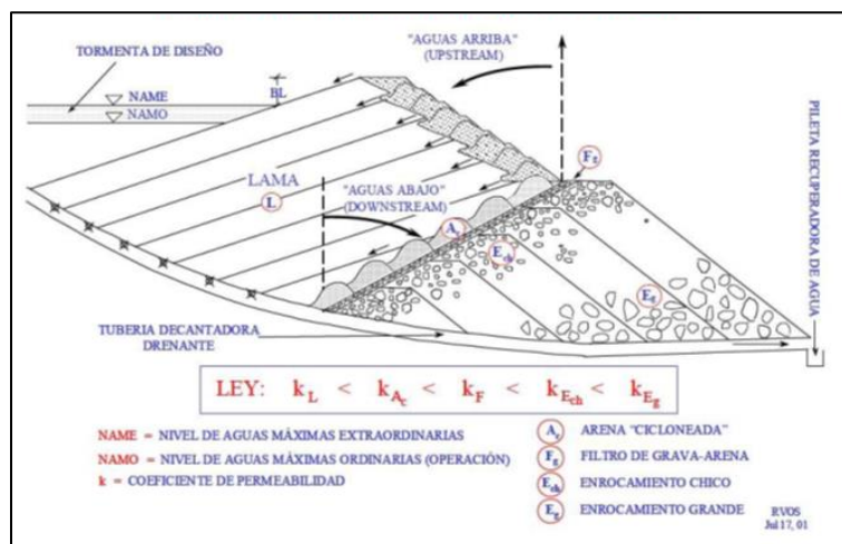
Figura II-16 .Método constructivo “aguas abajo y aguas arriba” con enrocamiento y arena cicloneada
