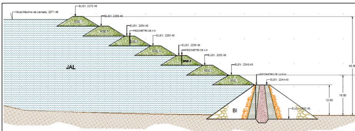
Figura III-27. Diseño geotécnico de un Depósito de jales filtrados
