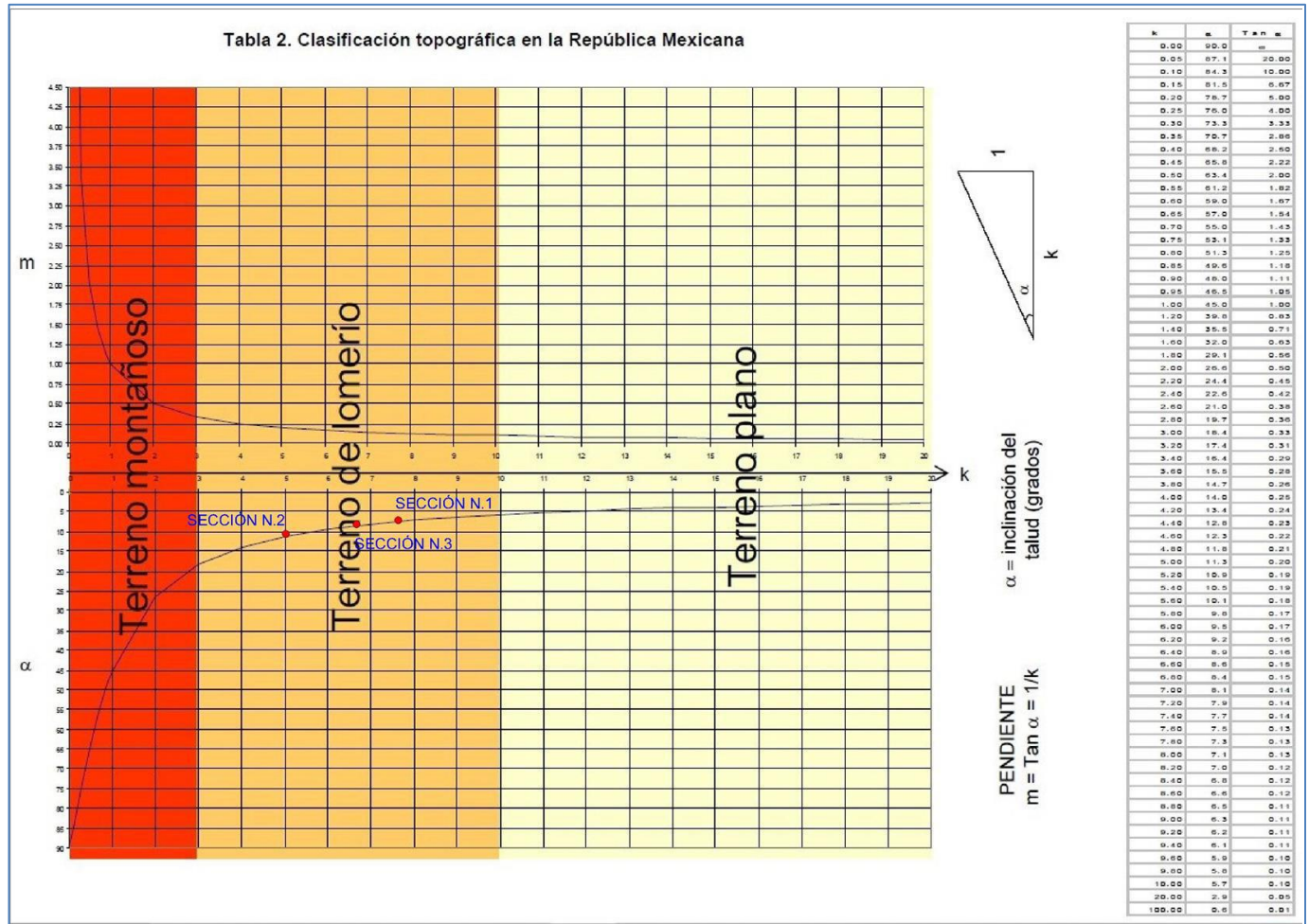
Figura II-6. Condición topográfica del sitio del proyecto de acuerdo a la Norma
