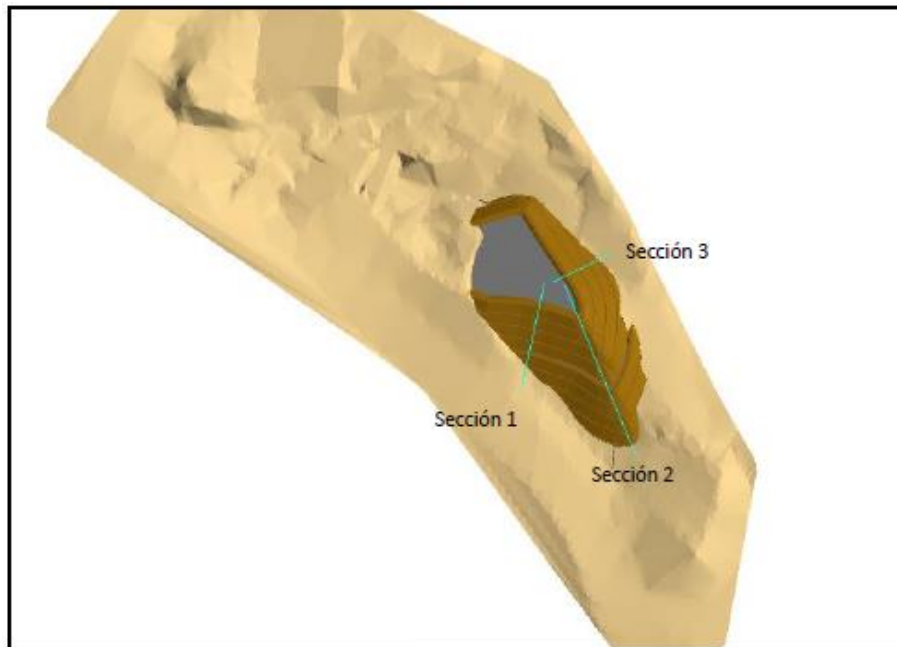
Figura II-22. Secciones utilizadas para el cálculo de estabilidad
