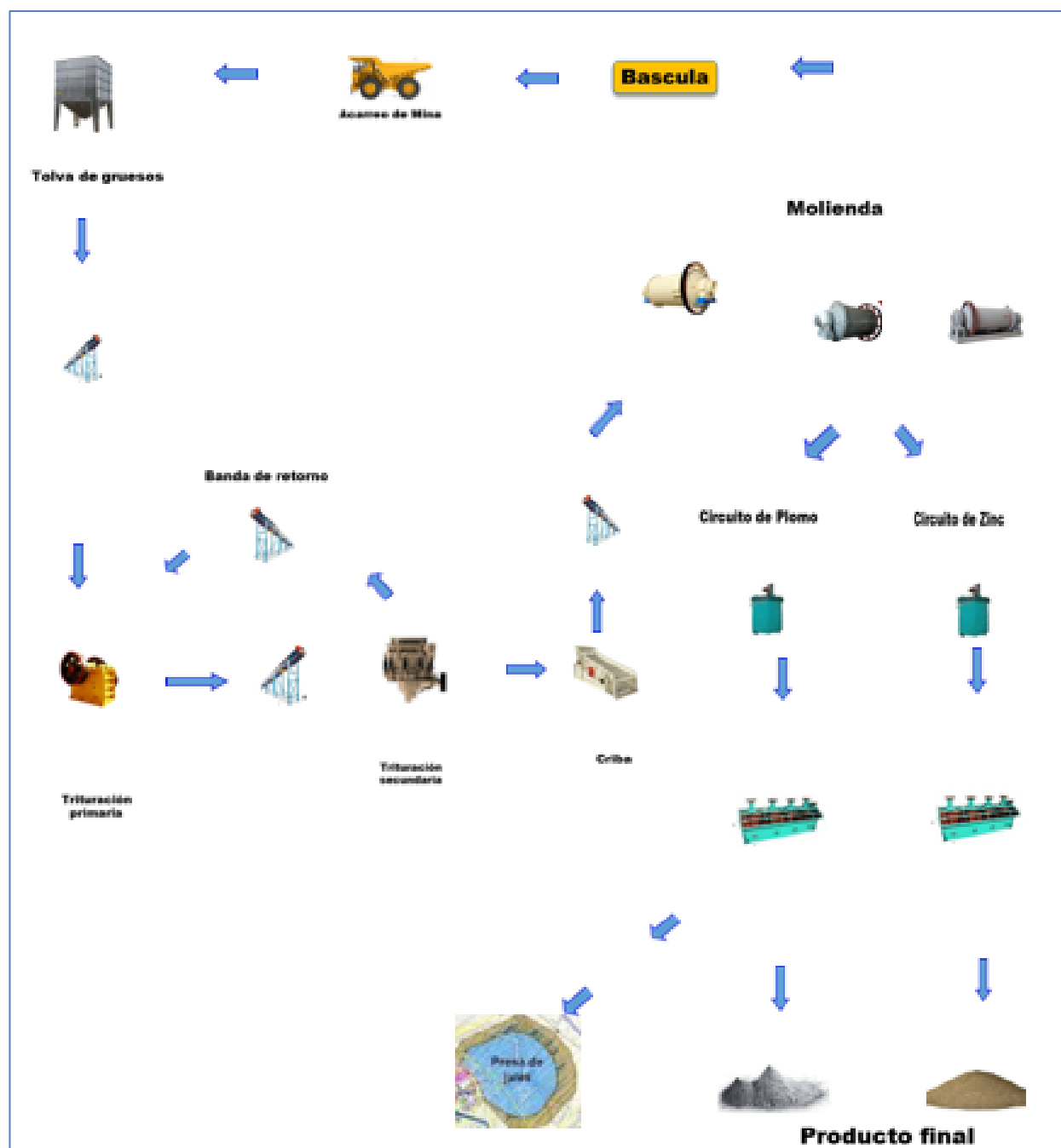
Figura II-28. Diagrama de flujo en el Beneficio de minerales y manejo de residuos
