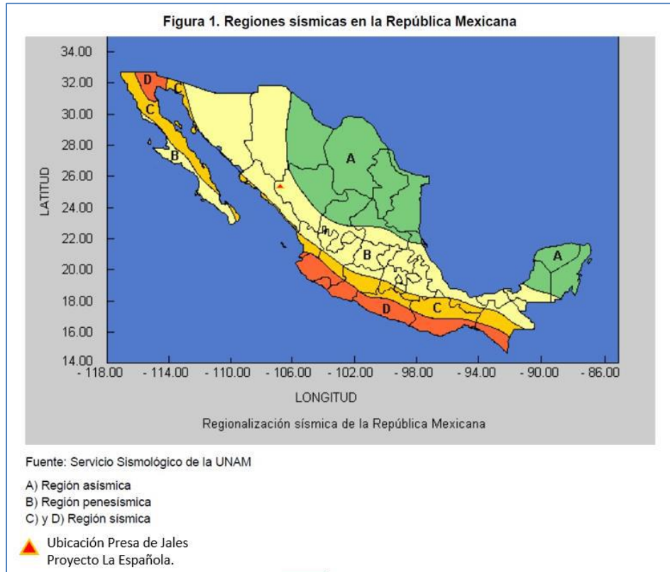
Figura III-9. Regiones sísmicas de la República mexicana
