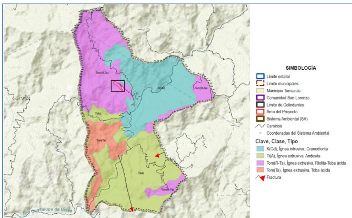
Figura IV-3. Tipo de Geología presente en el Sistema Ambiental
