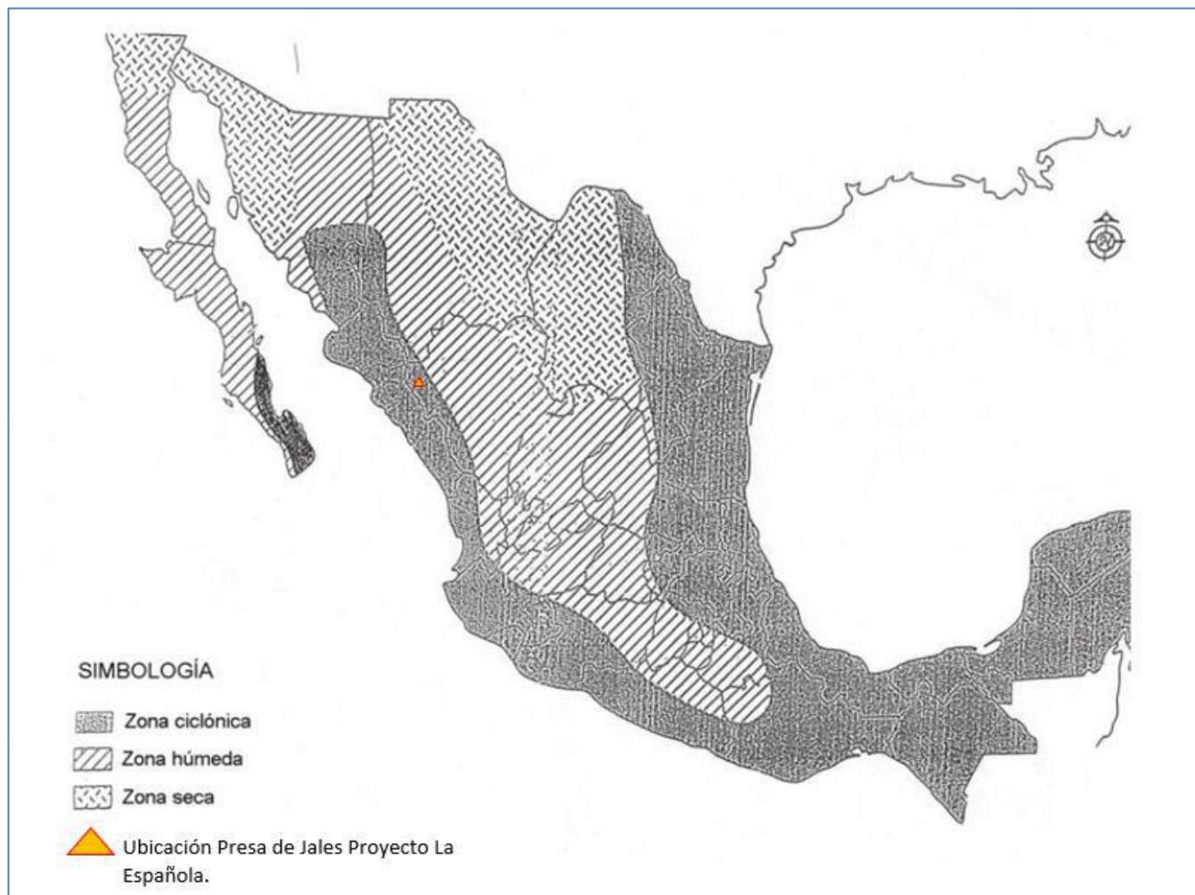
Figura II-2. Carta Hidrológica de la República Mexicana
