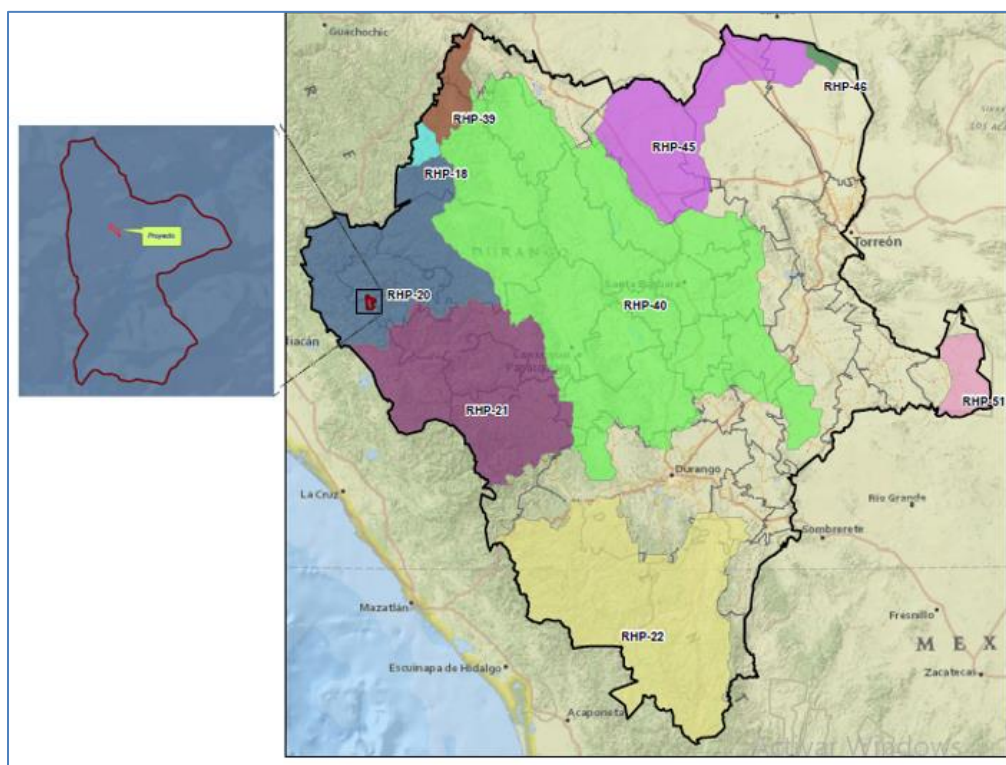
Figura III-3. Regiones hidrológicas prioritarias presentes en el proyecto
