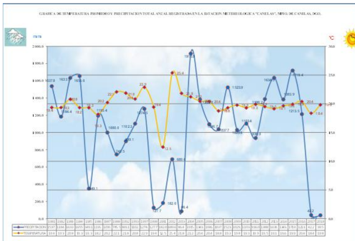
Figura IV-2. Gráfica representativa de la temperatura y precipitación media anual
