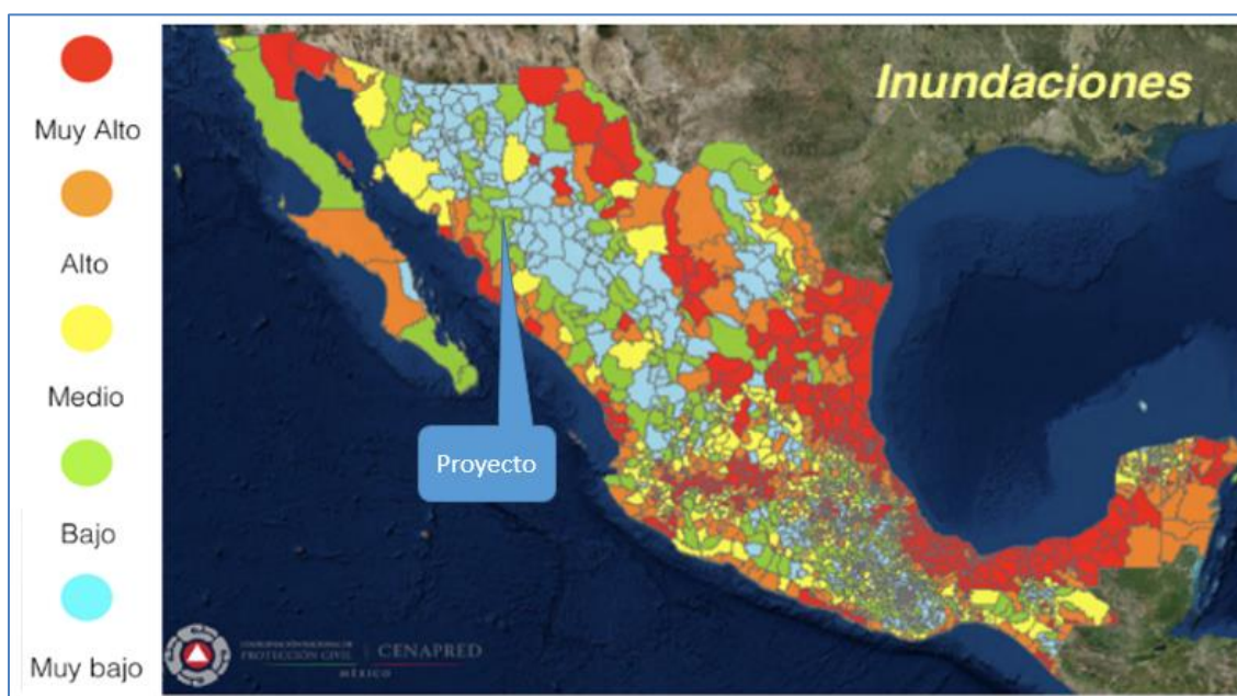
Figura IV-5. Ubicación del Sistema Ambiental con respecto a la susceptibilidad de peligro por inundación a nivel municipal
