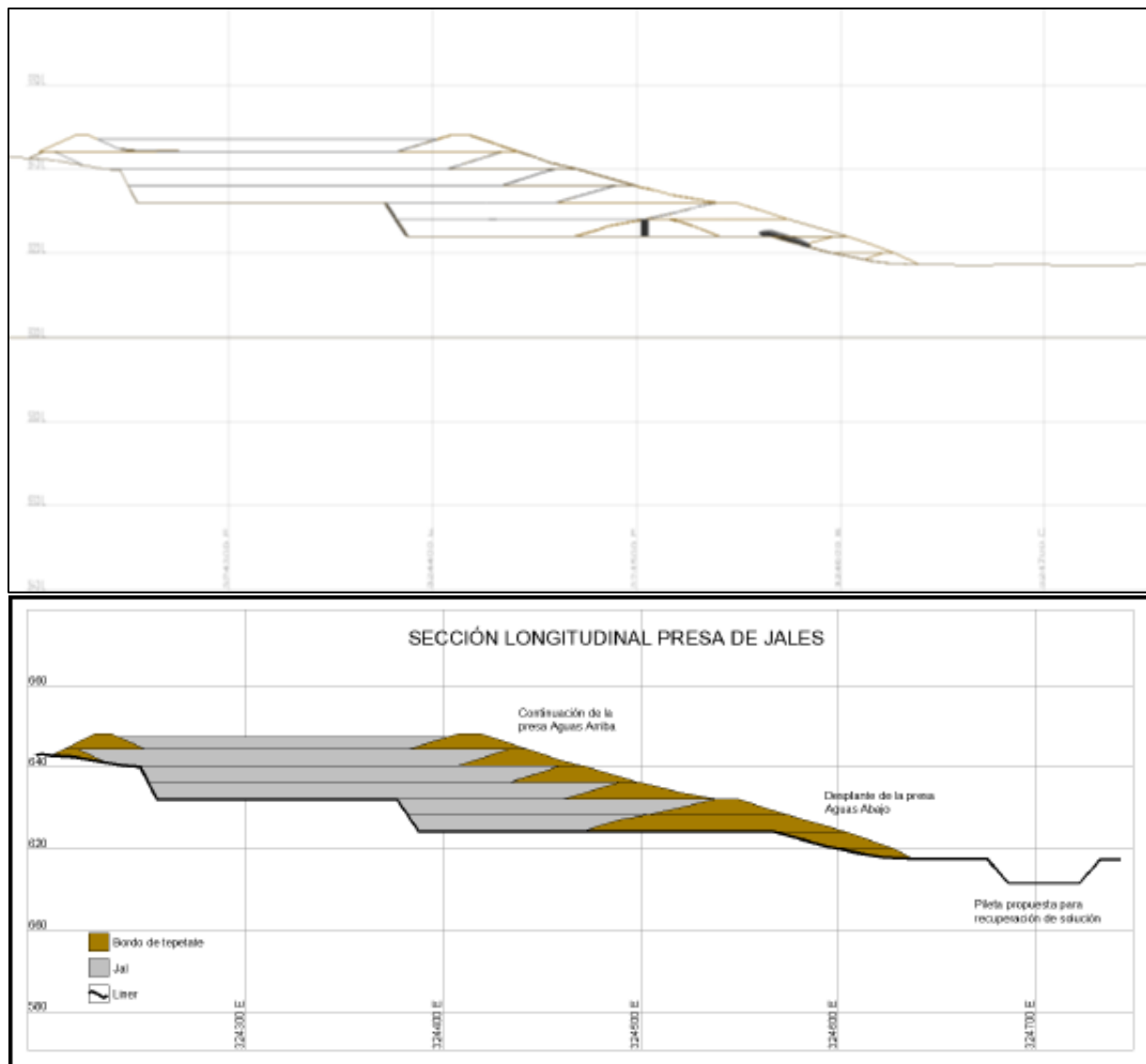
Figura II-21. Sección longitudinal del depósito de jales filtrados colmada
