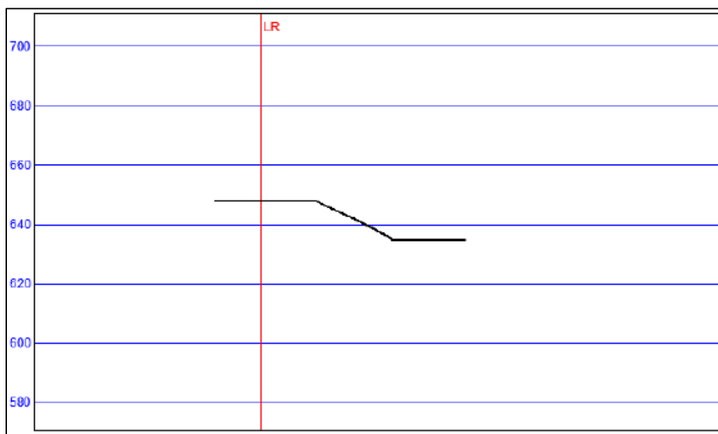
Figura II-25. Perfil topográfico – sección 3 – cálculo de estabilidad
