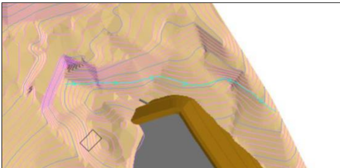
Figura II-26. Cuneta propuesta en la parte norte del depósito
