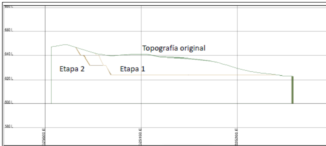
Figura II-11. Sección longitudinal indicando la topografía original y las etapas de corte 1 y 2
