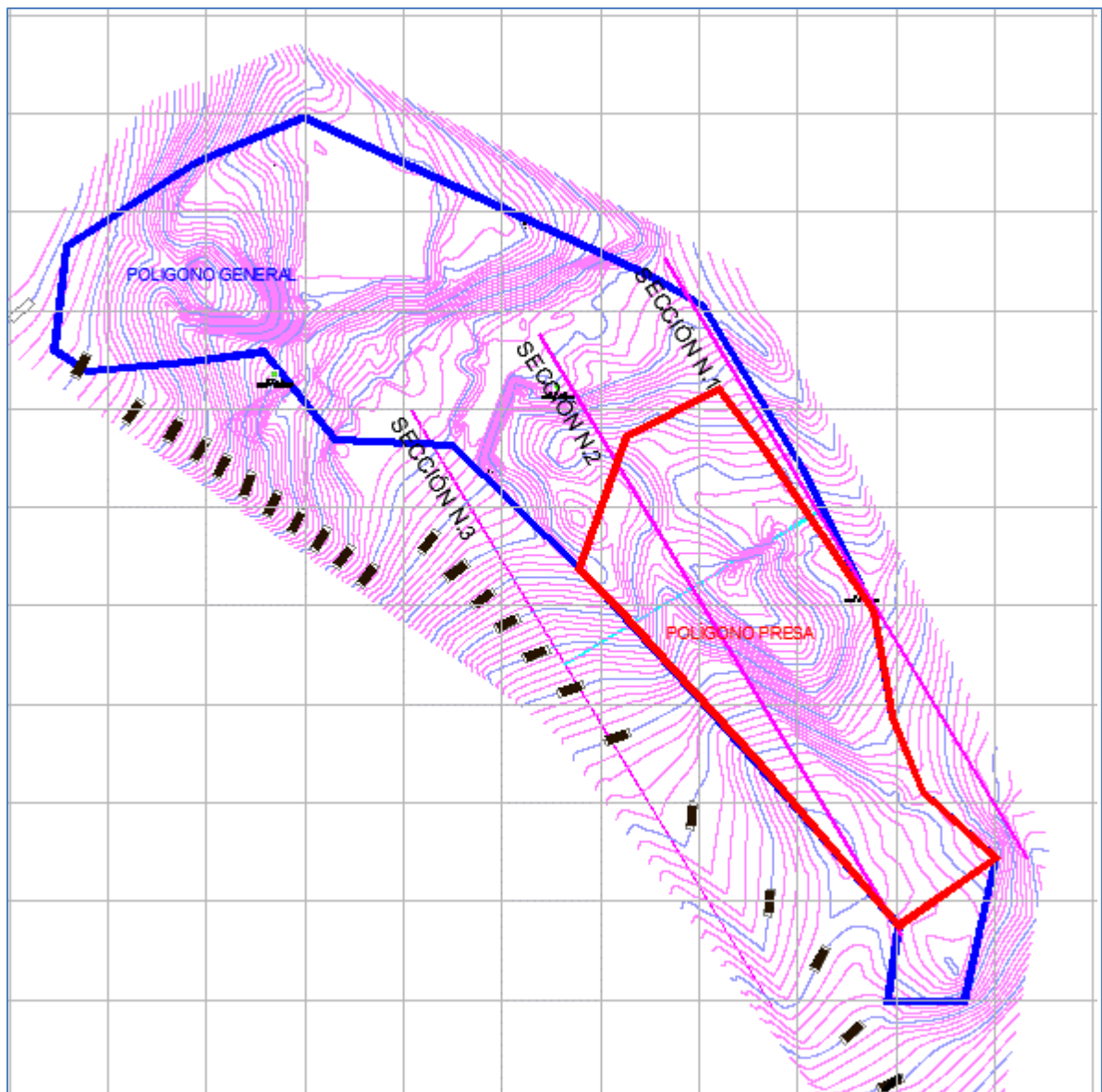
Figura II-3. Polígono general y secciones longitudinales
