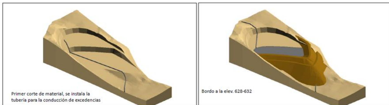
Figura III-26. Colocación de tubería de excedencias
