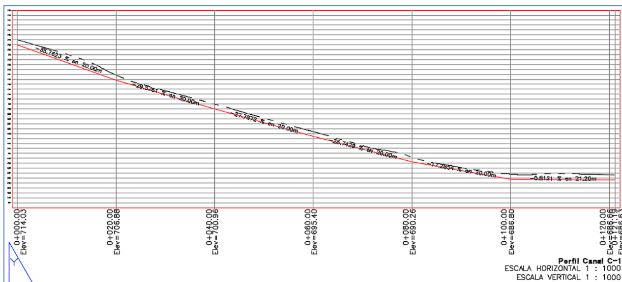
Figura III-21. Perfil natural y de proyecto del canal C-1
