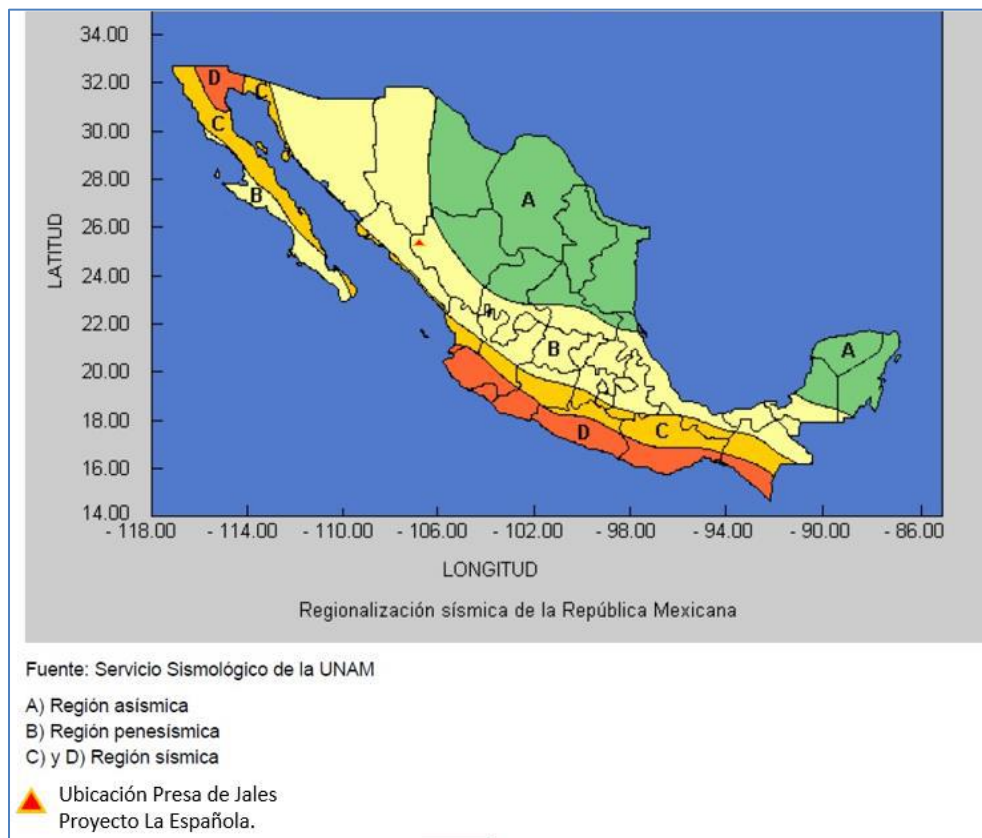
Figura II-7. Regiones sísmicas de la República Mexicana
