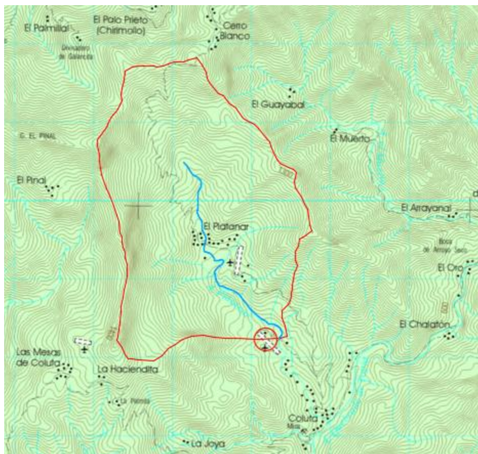
Figura III-16. Características fisiográficas del sitio del proyecto con respecto a la cuenca de aporte
