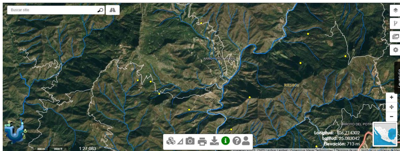
Figura IV-8. Hidrología superficial en el Sistema Ambiental
