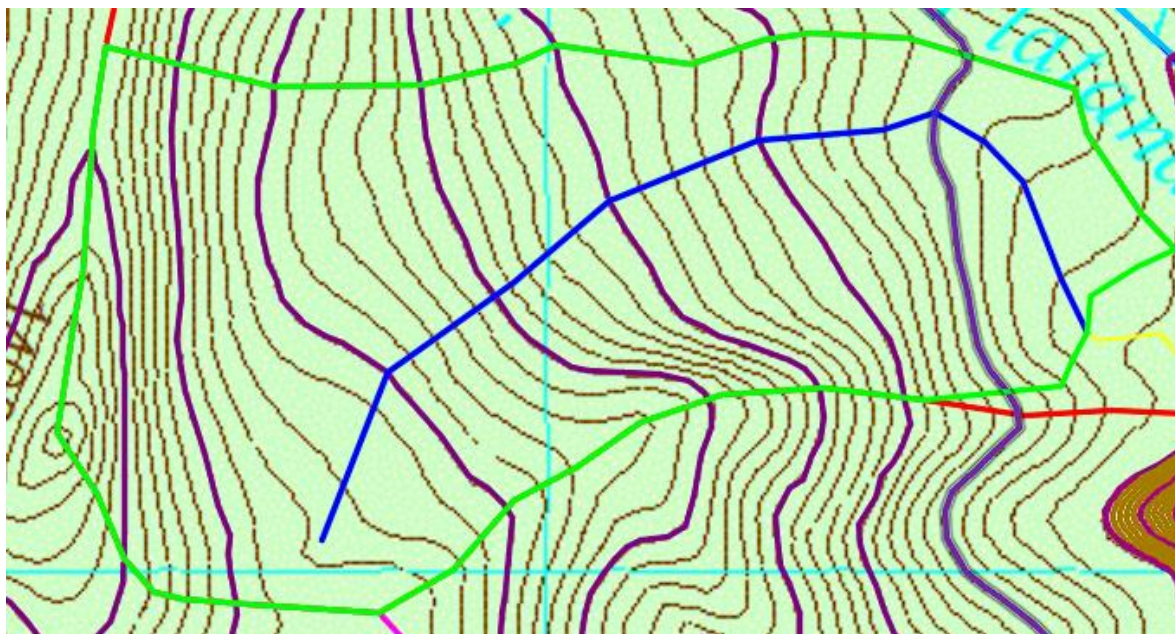
Figura III-24. Esguerrimiento de la cuenca de aportación
