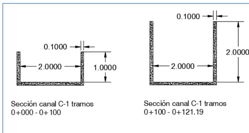
Figura III-23. Secciones transversales del canal C-1
