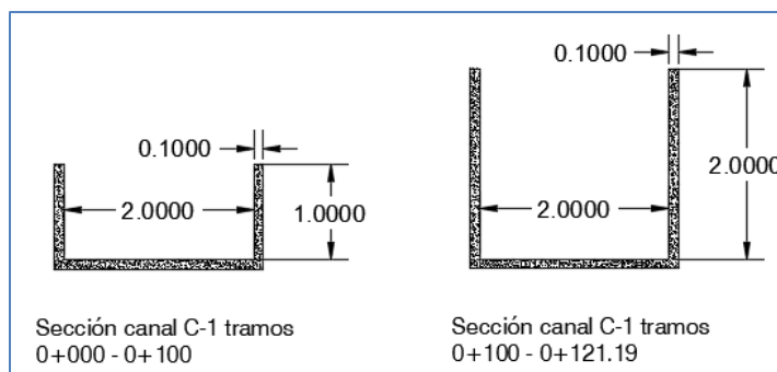
Figura III-19. Secciones de la obra de desvío
