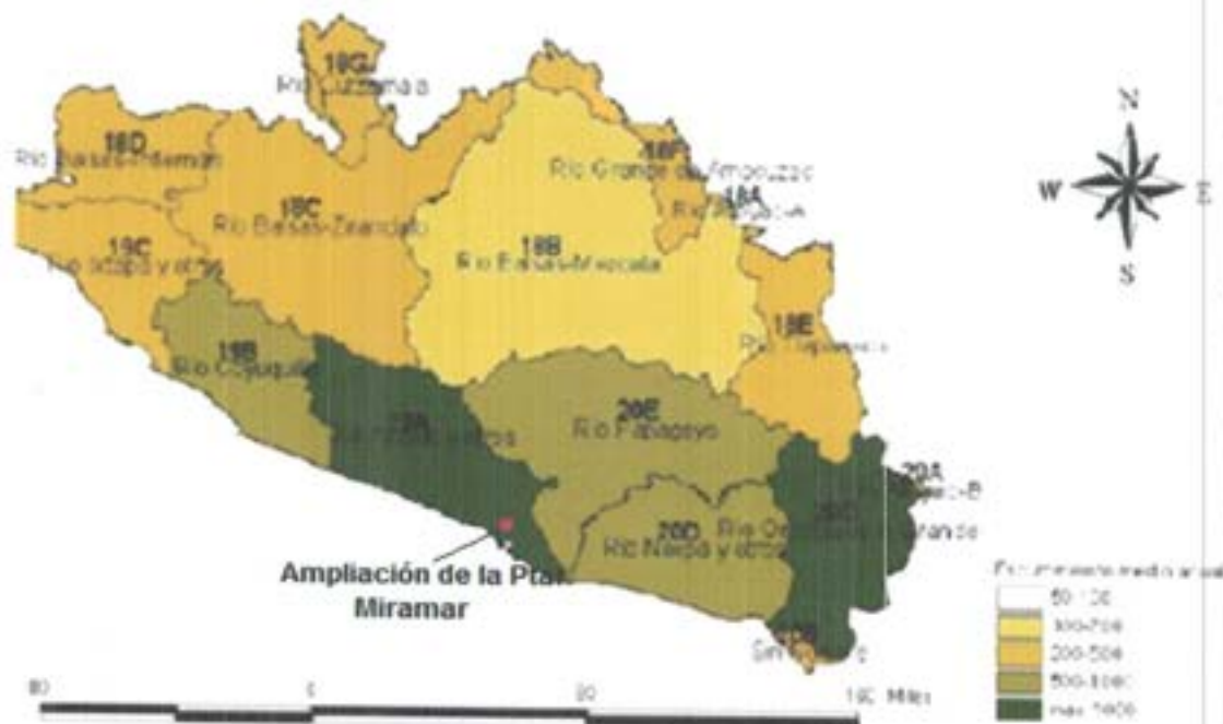
Cuencas hidrográficas y escurrimiento medio anual (en mm).
