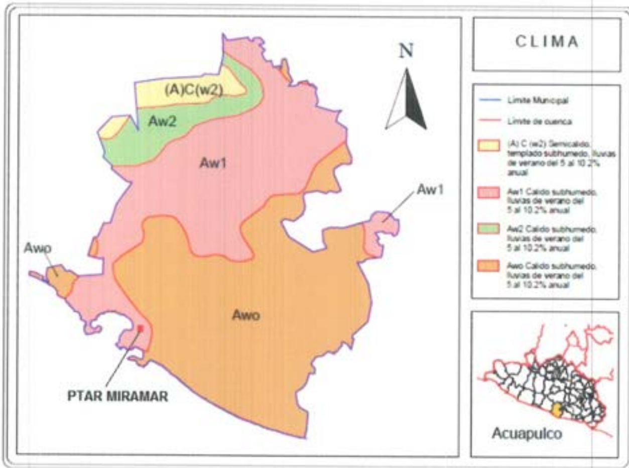
Clima en la ubicación del predio
