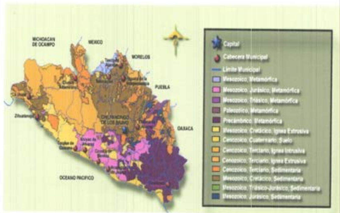
PLANO DE GEOLOGIA DEL ESTADO DE GUERRERO.
