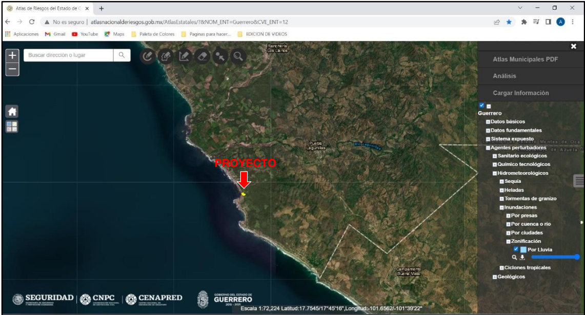
Ilustración IV.2.15. Riesgo a inundaciones para la región del proyecto.
