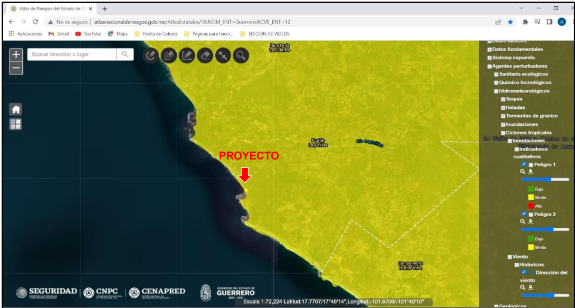
Ilustración IV.2.16. Riesgo a ciclones tropicales para la región del proyecto.
