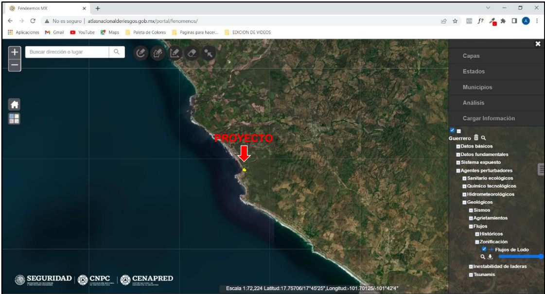
Ilustración IV.2.20. Riesgo de flujos de lodo para la región del proyecto.
