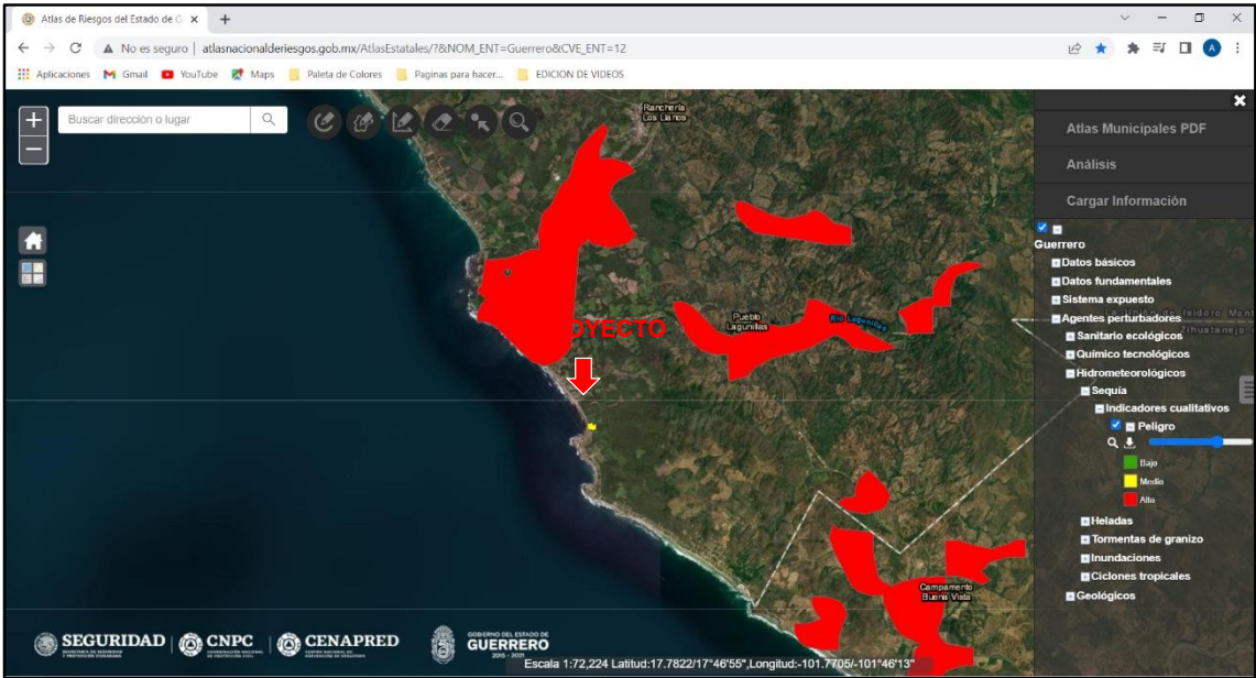
Ilustración IV.2.11. Riesgo de sequias para la región del proyecto.
