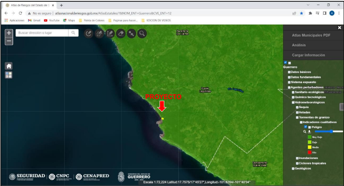
Ilustración IV.2.13. Riesgo de Tormentas de granizo para la región del proyecto.
