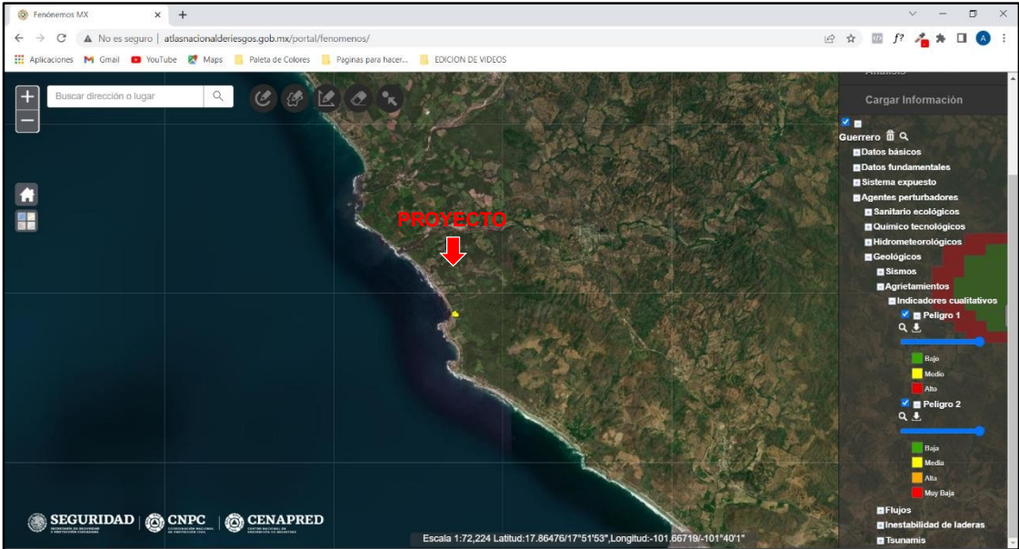
Ilustración IV.2.19. Riesgo de agrietamientos para la región del proyecto.
