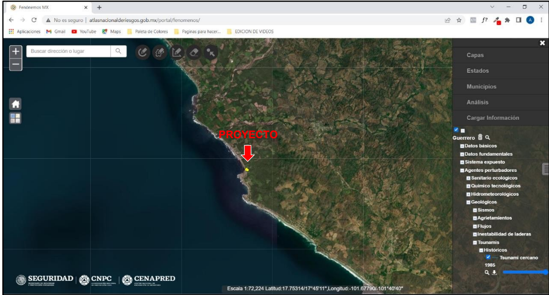
Ilustración IV.2.21. Riesgo de tsunami para la región del proyecto.
