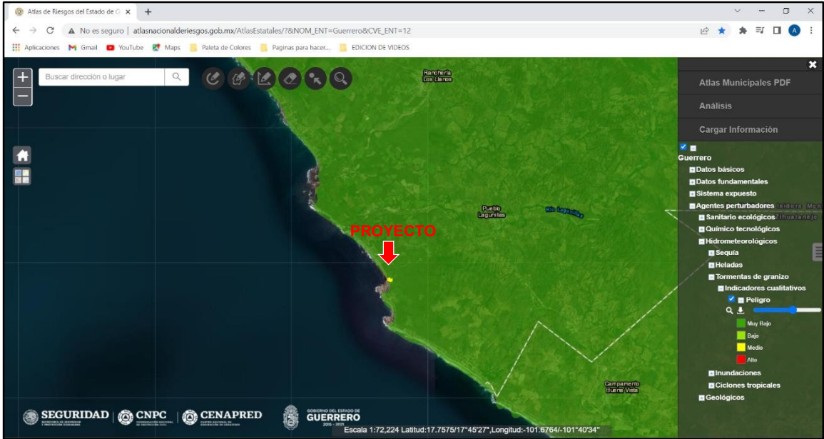
Ilustración IV.2.14. Riesgo de granizo para la región del proyecto.
