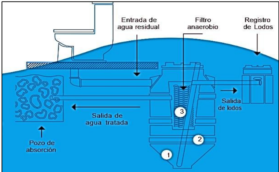
Ilustración II.2.5.2. Características de la Planta de Tratamiento.
