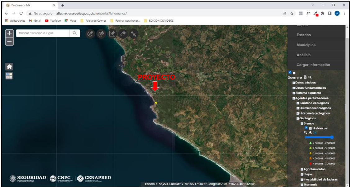
Ilustración IV.2.18. Riesgo a sismos para la región del proyecto.
