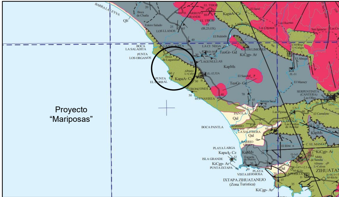
Ilustración IV.2.6. Carta geológica de la zona del proyecto.
