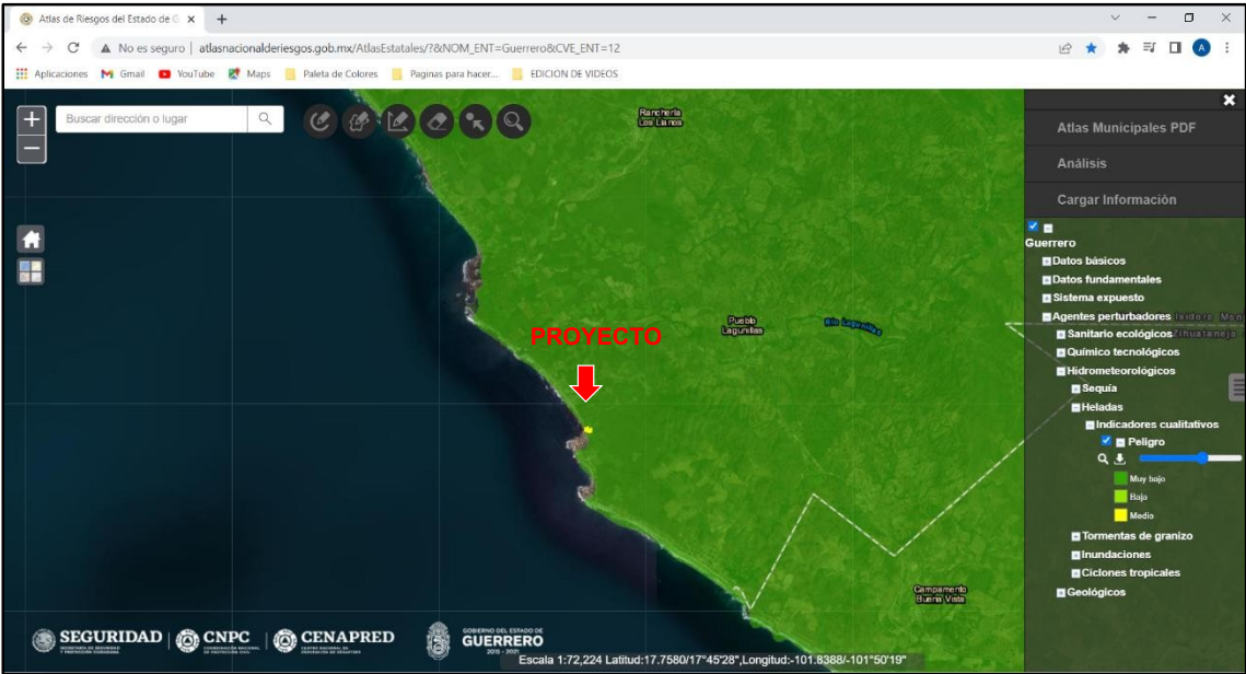
Ilustración IV.2.12. Riesgo de heladas para la región del proyecto.
