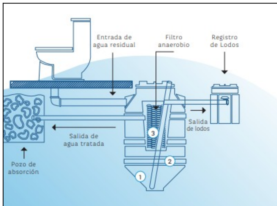
Ilustración II.2.5.2. Proceso del Biodigestor.
