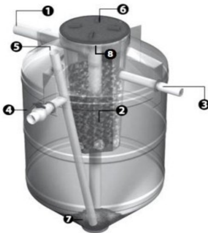
Ilustración II.2.5.3. Componentes del Biodigestor.
