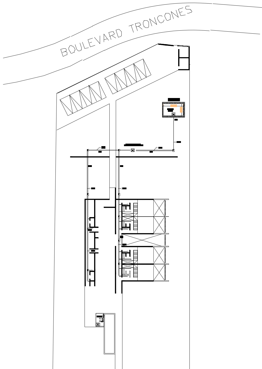
Imagen 10. Plano de sistema de tratamiento de aguas residuales.
