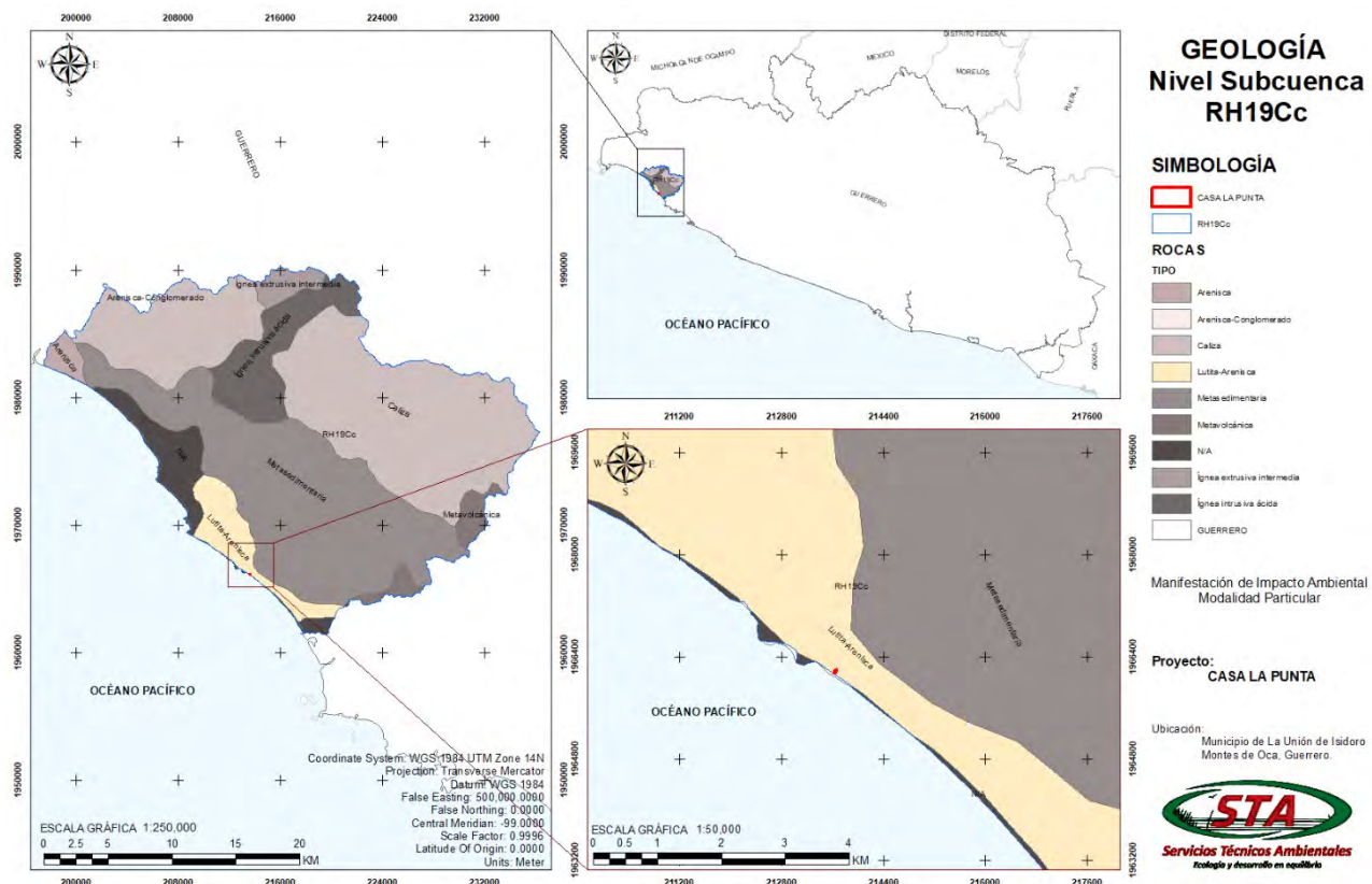
Imagen 24. Muestra la geología para el área de influencia del proyecto, el cual corresponde a lutita-arenisca. Fuente: www.inegi.org.mx
