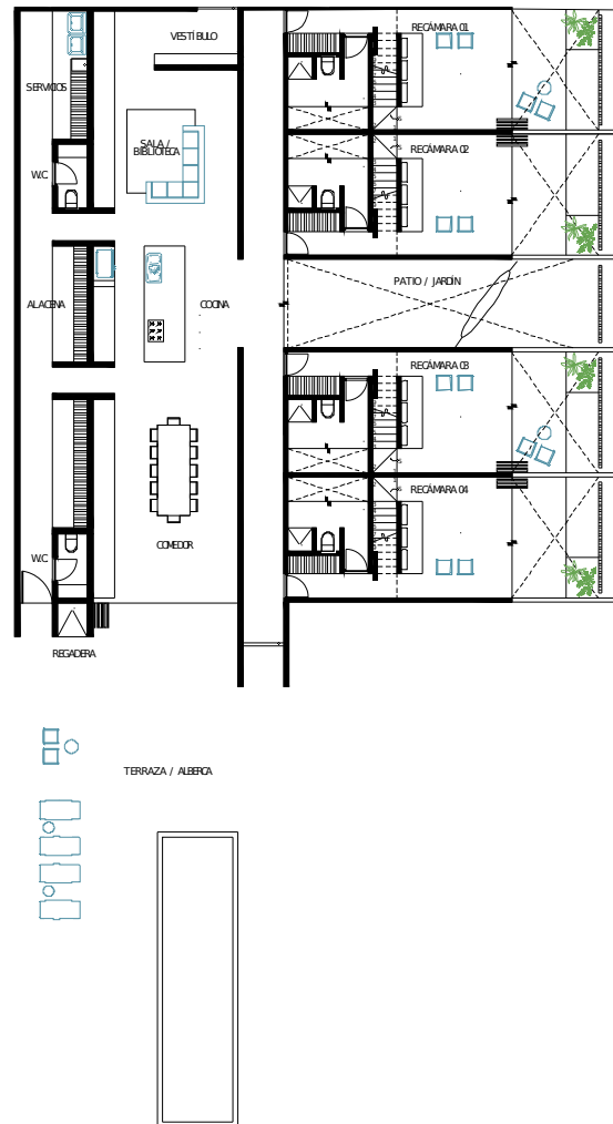
Imagen 14. Dimensiones del proyecto propuesto.
