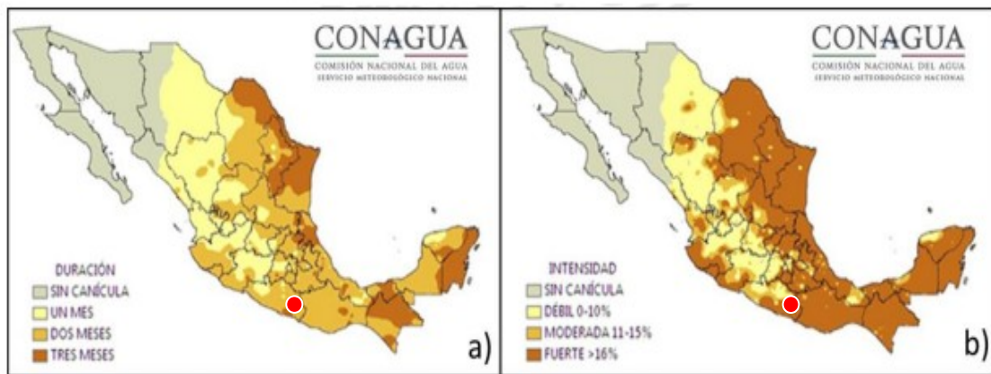
Fig. 2. a) Duración de la canícula en meses, b) Intensidad de la canícula en %. Para el cálculo de los mapas se utilizó información disponible de 985 estaciones en el periodo mayo-septiembre de 2014 en el Sistema de Información Hidroclimatológica (SIH) de la Gerencia de Aguas Superficiales e Ingeniería de Rios-Conagua, cualquier cálculo posterior podrá resultar diferente.
