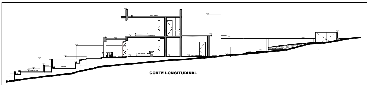
Imagen 13. Corte longitudinal.
