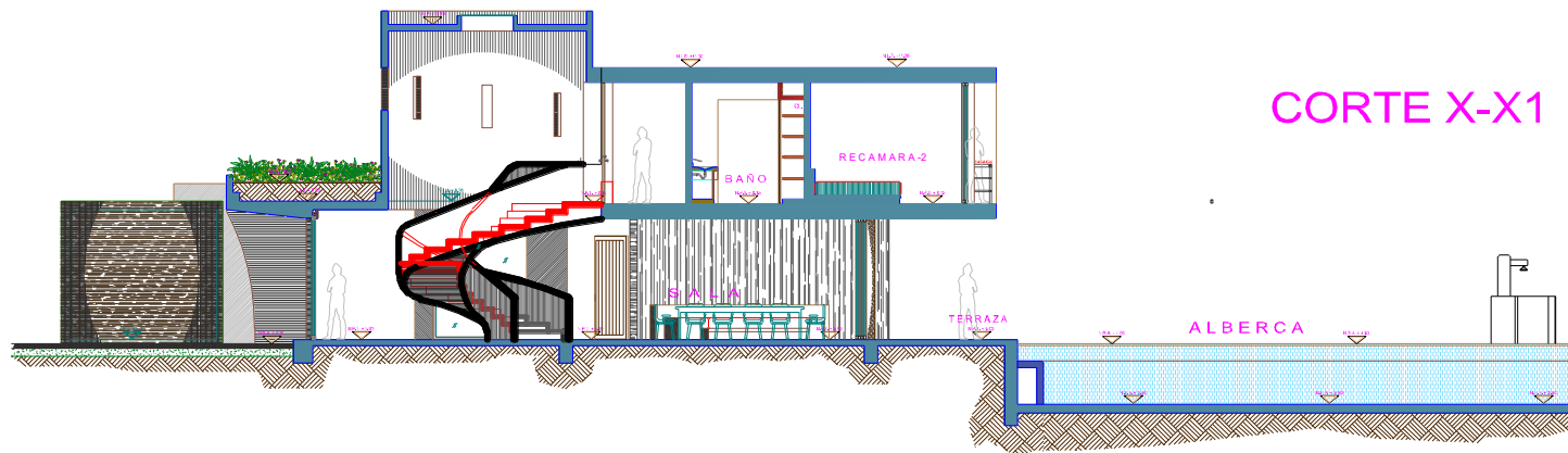
Imagen 07. Presenta los cortes de las obras propuestas al interior del lote 50 B.
