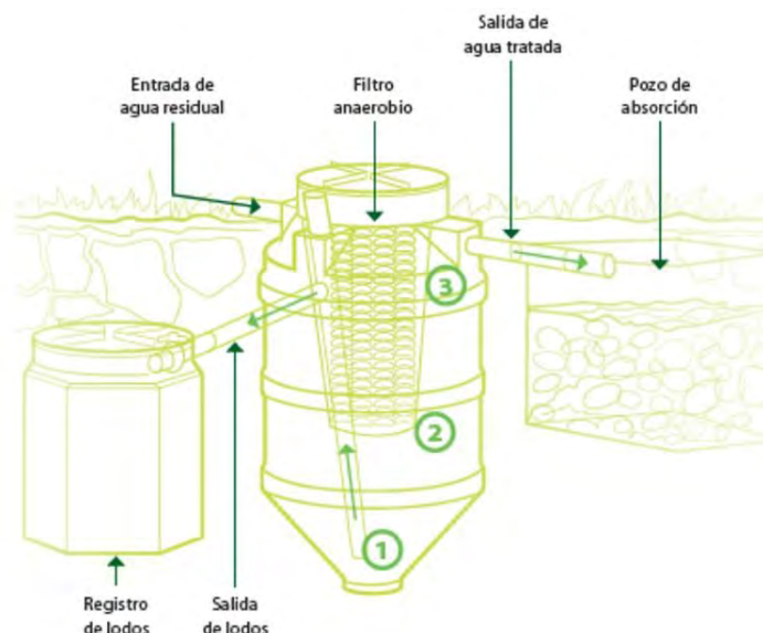
Imagen 26. Ficha técnica biodigestor autolimpiable
