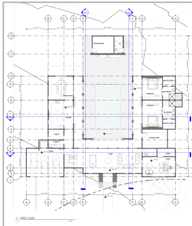
Figura II.5 Diagrama general del proyecto
