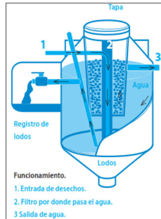
Imagen 7. Funcionamiento del Biodigestor Autolimpiable
