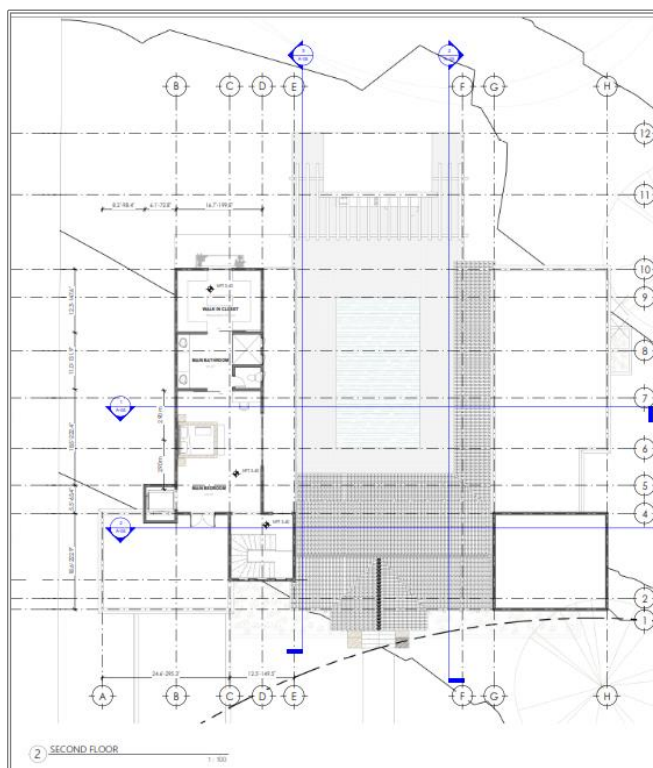
Imagen 2. Detalle del diagrama del polígono de la casa segundo nivel
