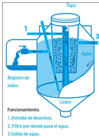
Imagen 1. Funcionamiento del Biodigestor Autolimpiable
