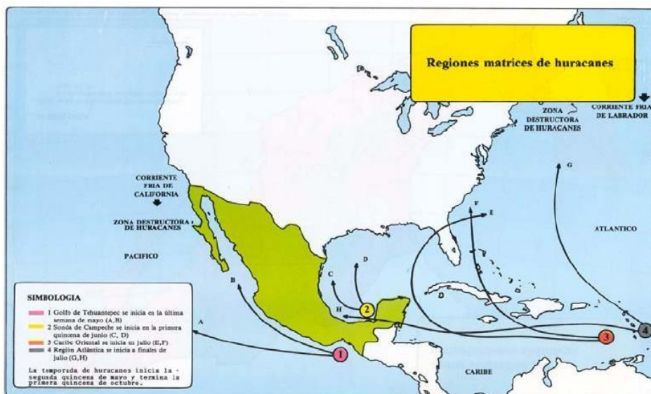
Figura IV.2. Regiones matrices de huracanes
