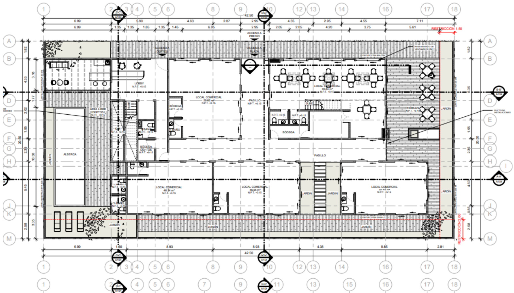
Planta arquitectónica Planta Baja
