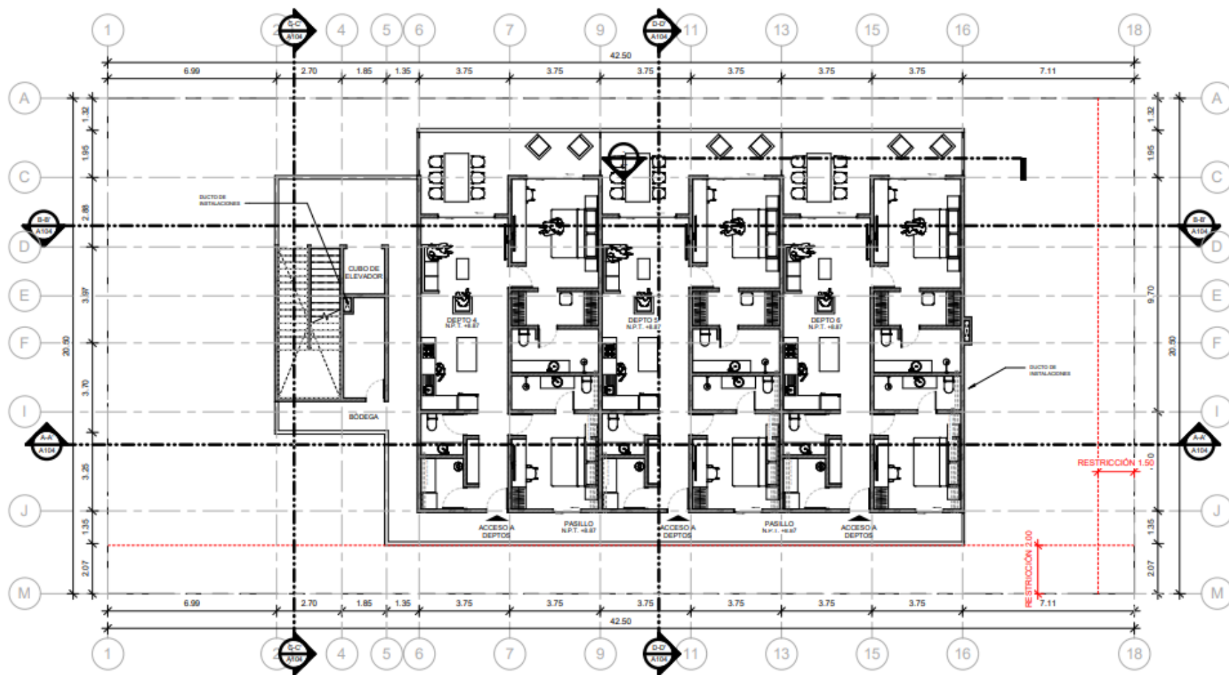
Planta arquitectónica Segundo Nivel
