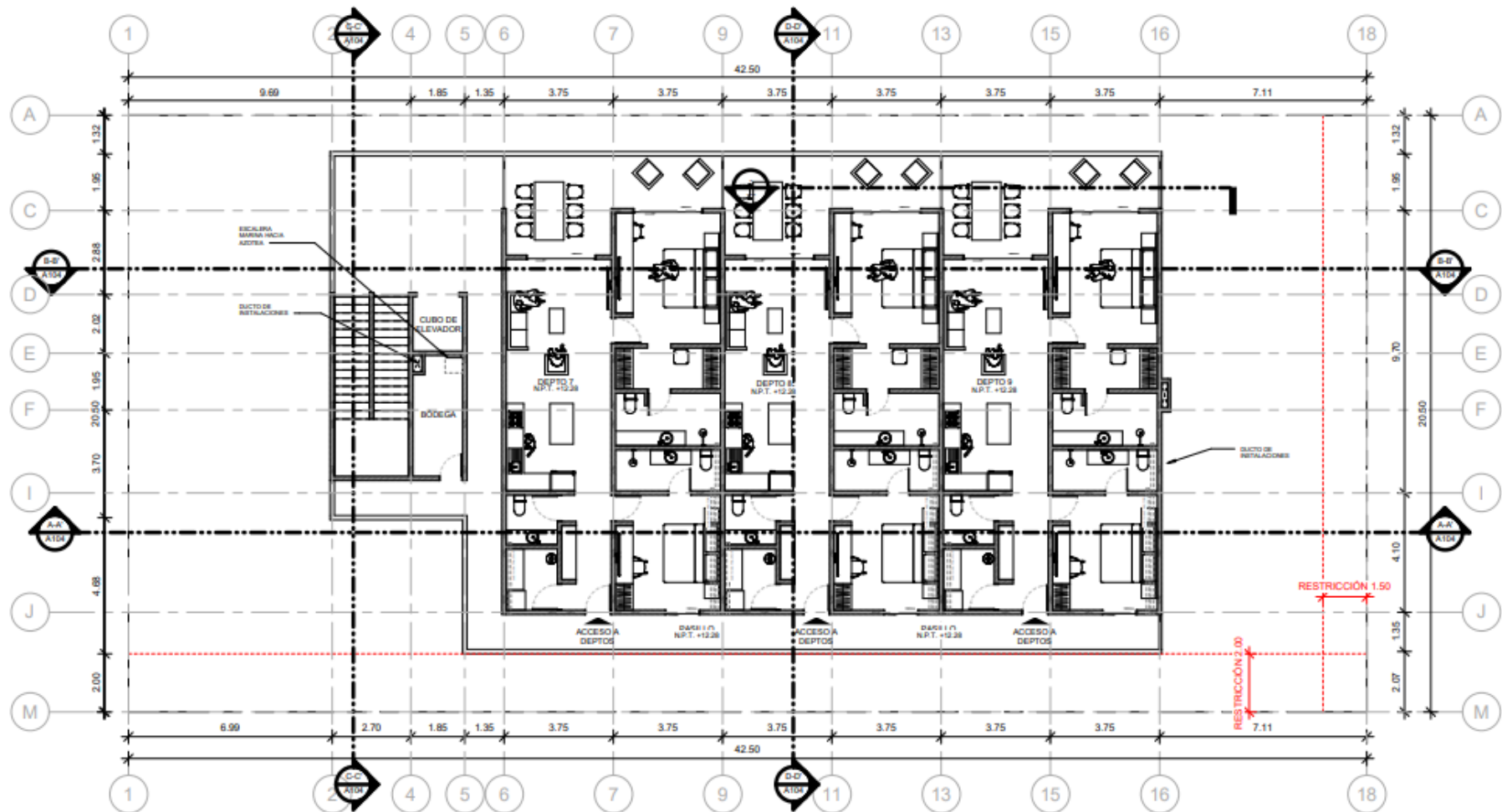
Planta arquitectónica Tercer Nivel
