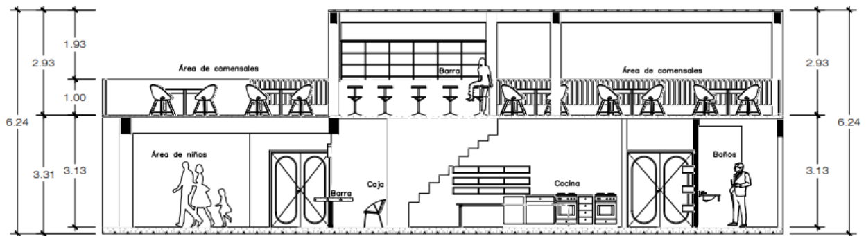
Imagen 10. Corte vertical de la planta arquitectónica.
