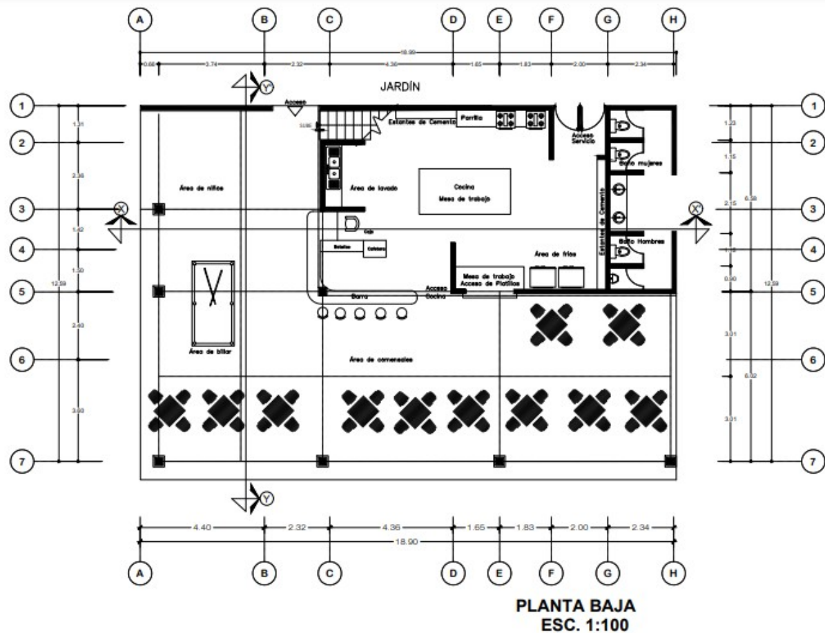
Imagen 9. Planta arquitectónica del Restaurante Rockaway.
