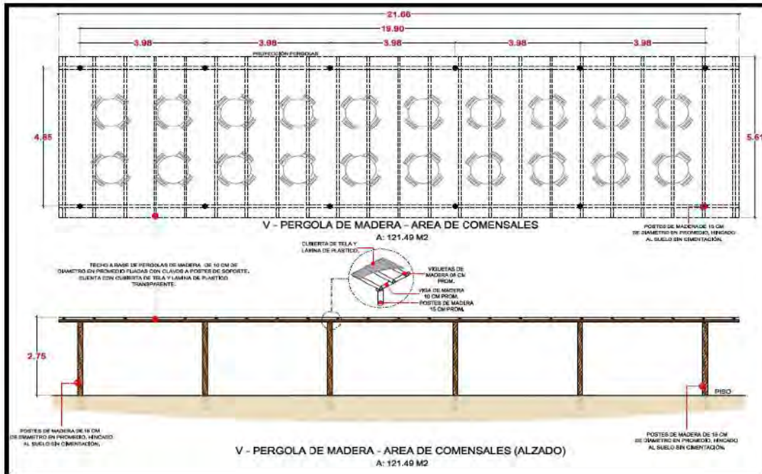
Imagen 14. Pérgola usos múltiples (comensales)
