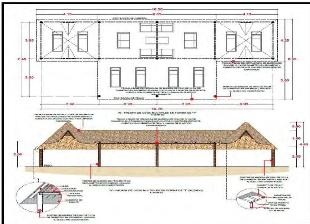
Imagen 13- Palapa de usos múltiples en forma de T
