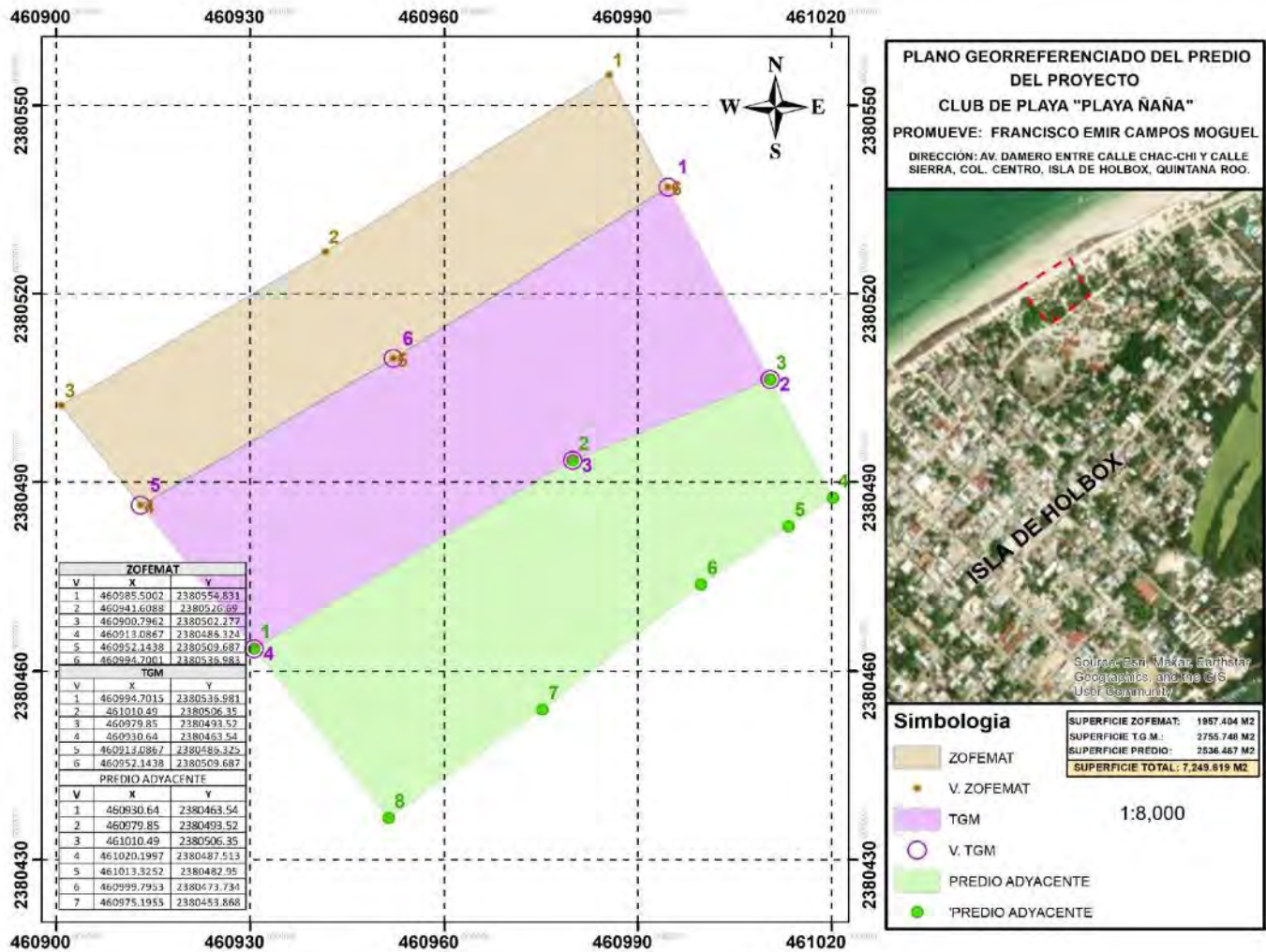
Imagen 2. Plano georreferenciado del predio del Proyecto (por zona)
