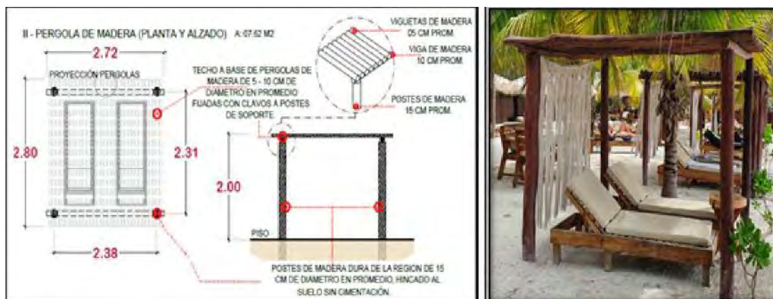
Imagen 10. 10 pérgolas de madera (Instalación sancionada por la PROFEPA )
