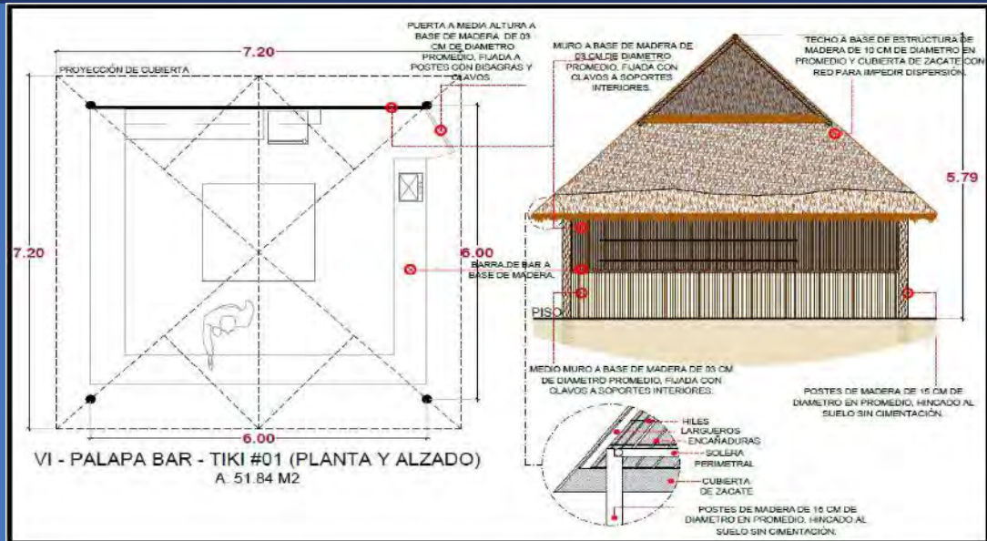
Imagen 15.1 Palapa bar Tiki # 1 (PROPUESTA DE AMPLIACION)
