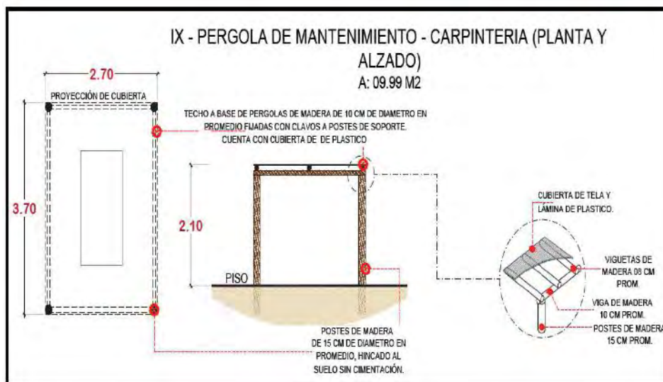
Imagen 19. Pérgola de mantenimiento.
