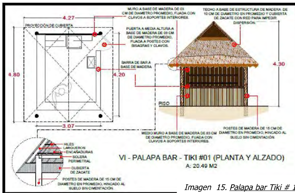
Palapa Bar # 1 (Tiki).
