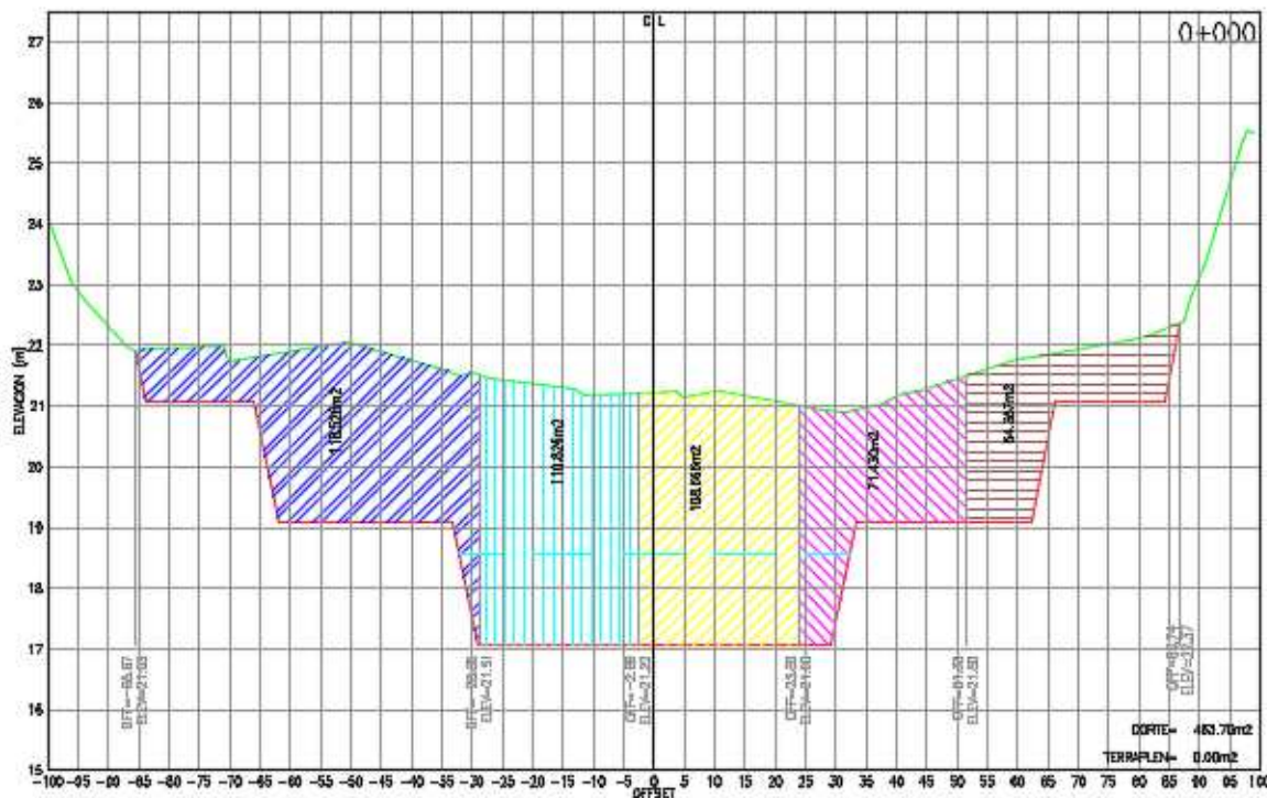
FIGURA 2. ESTACION 0+000.000 (Aguas más arriba del proyecto): AREA DE TERRAPLEN = 0.00 m 2 AREA DE CORTE = 463.70 m 2
