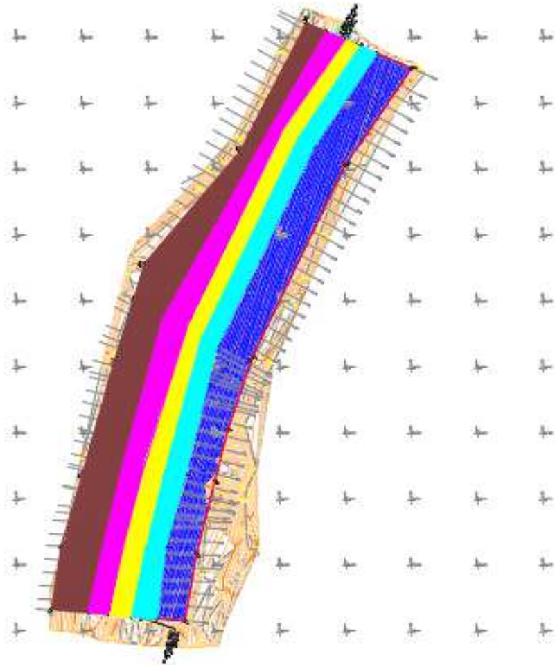
FIGURA 7. 2 SECCIONES, 5 FRENTES DE EXTRACCIÓN DIVIDIDOS EN 32 ESTACIONES. (PLANO PLANTA DE EXTRACCIÓN)
