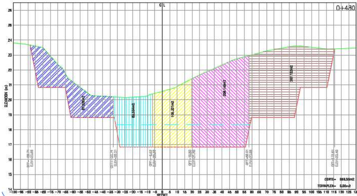
FIGURA 3. ESTACION 0+480.000 (Parte central del proyecto): AREA DE TERRAPLEN = 0.00 m 2 AREA DE CORTE = 698.95 m 2
