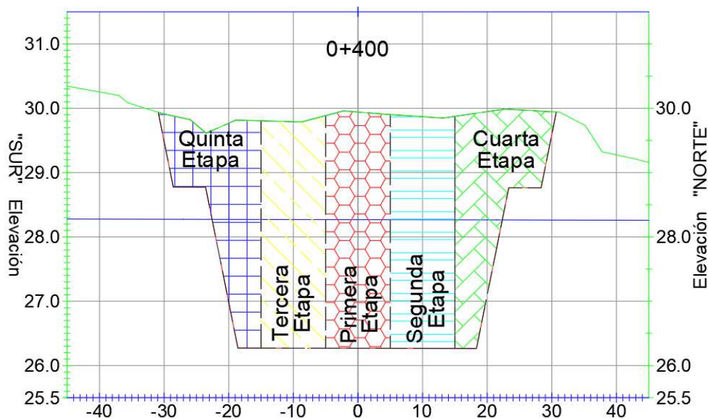
Imagen No. 7.- Sección de extracción típica.
