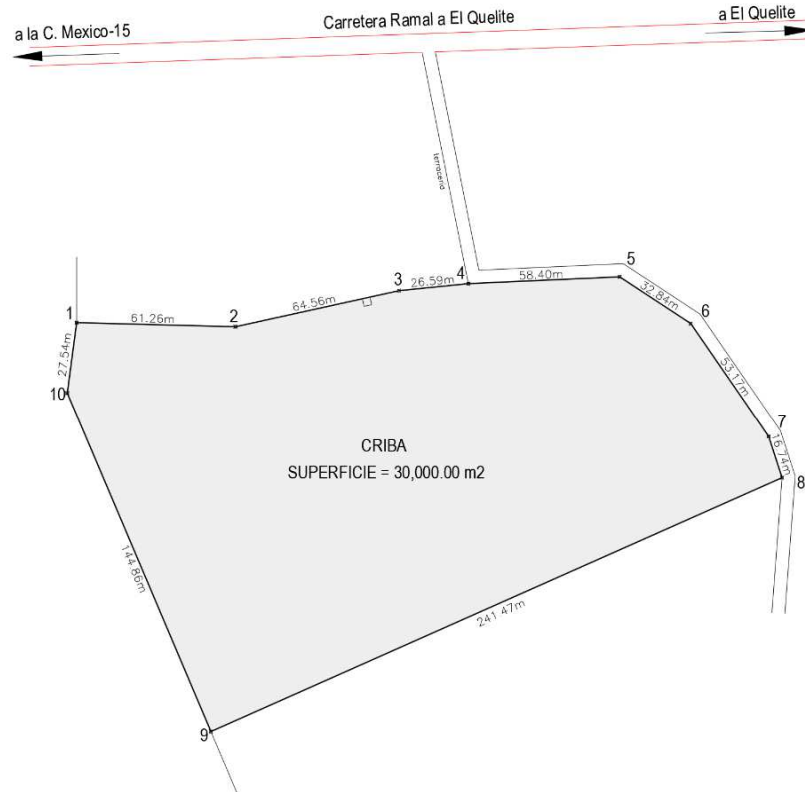
Imagen No. 19.- Dimensiones de la criba.
