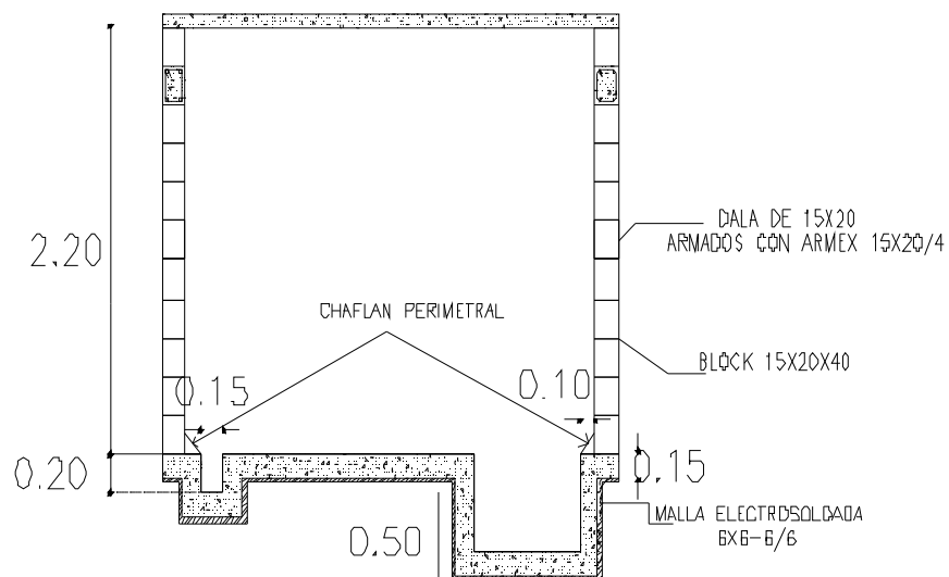
Imagen No. 13.- Diseño del almacén temporal de residuos peligrosos.
