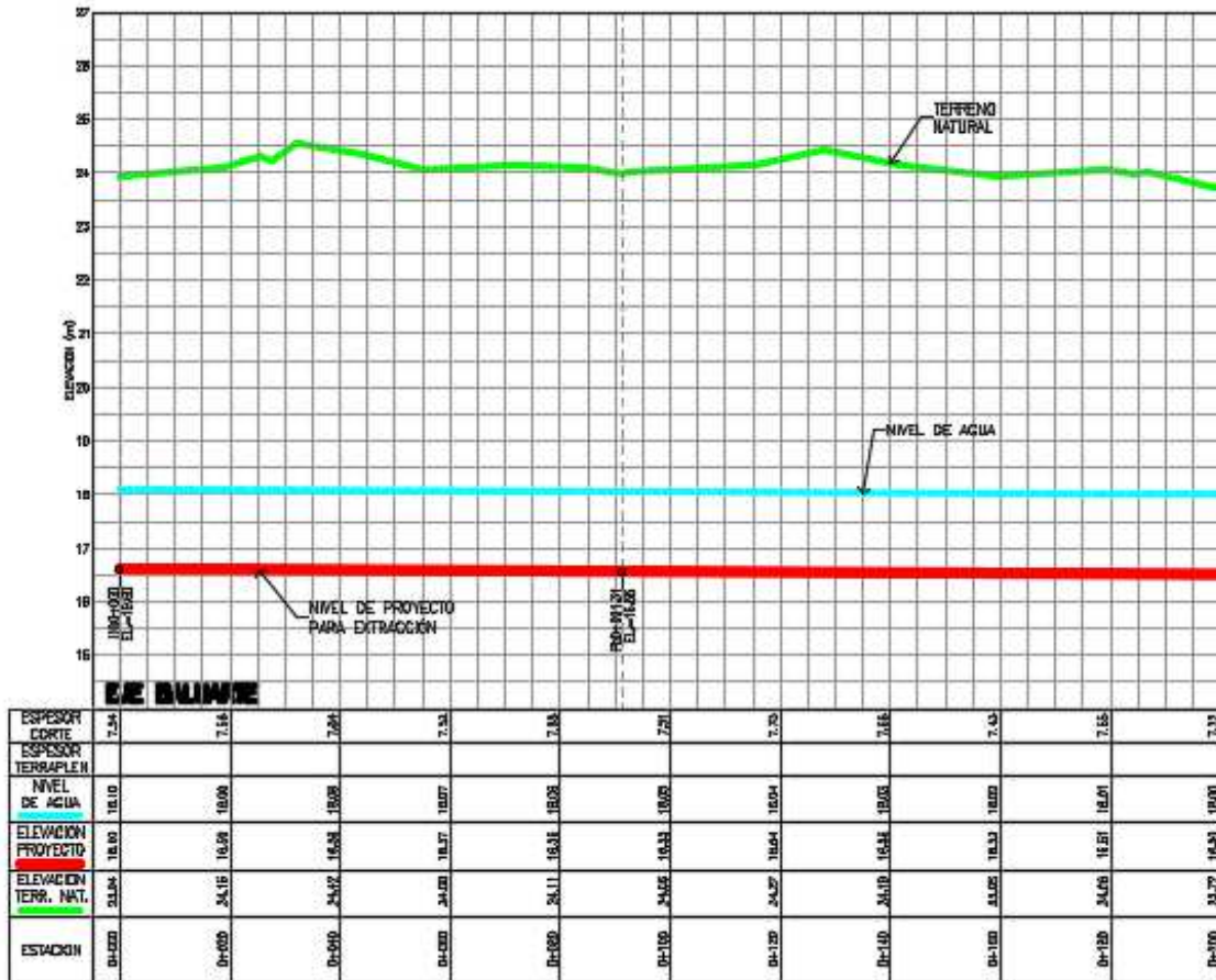
FIGURA 5. CORTE TRANSVERSAL, DE LA ESTACIÓN 0+000.000 A LA ESTACIÓN 0+360.000.
