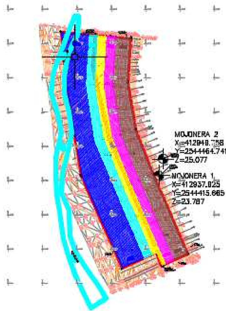
FIGURA 7. 2 SECCIONES, 5 FRENTES DE EXTRACCIÓN DIVIDIDOS EN 41 ESTACIONES. (PLANO PLANTA DE EXTRACCIÓN)
