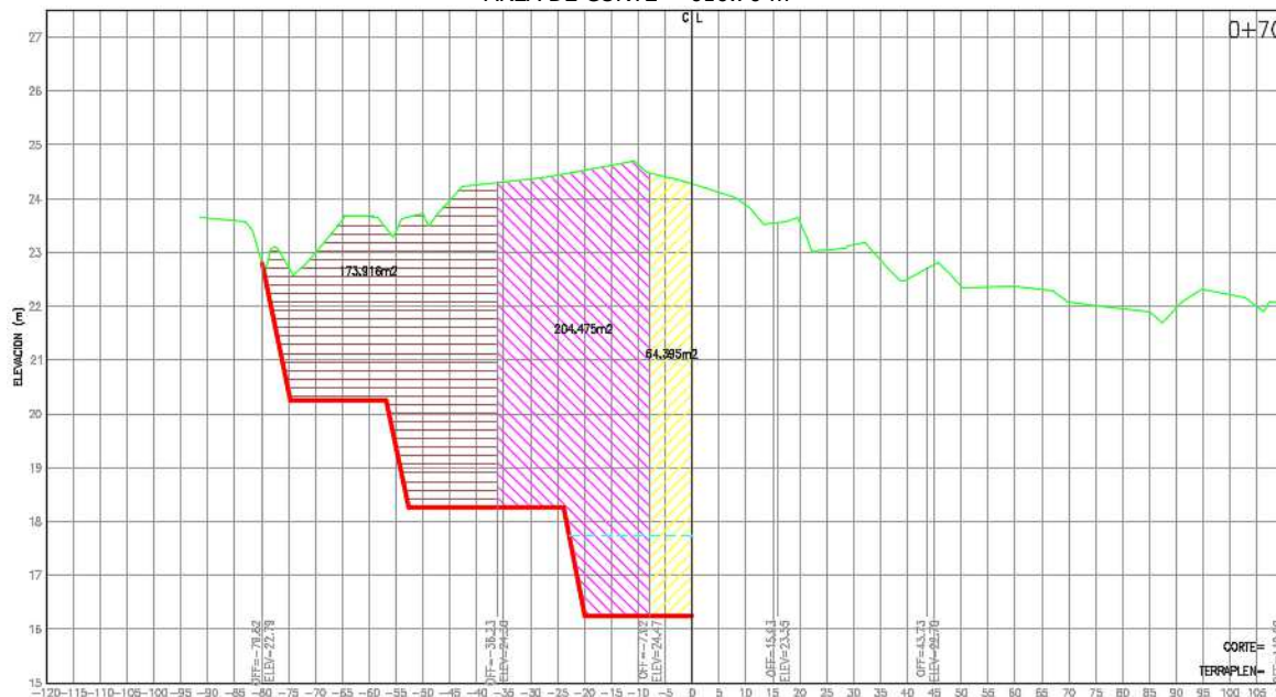
FIGURA 4. ESTACION 0+706.93 (Parte final del proyecto):
