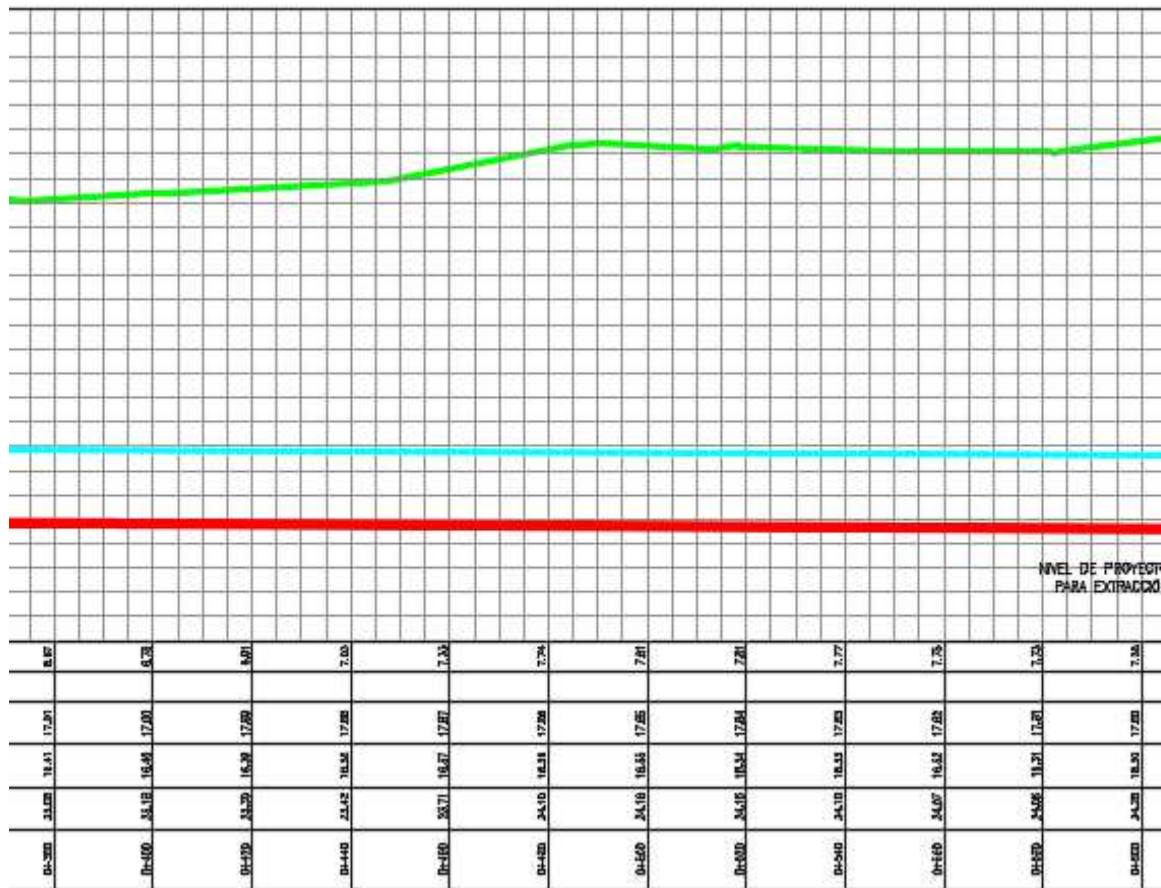
FIGURA 6. CORTE TRANSVERSAL, DE LA ESTACIÓN 0+380.000 A LA ESTACIÓN 0+706.930.
