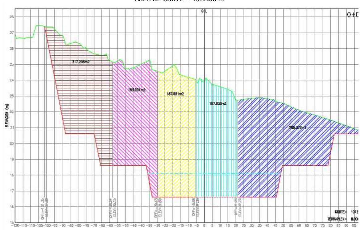
FIGURA 2. ESTACION 0+000.000 (Aguas más arriba del proyecto): AREA DE TERRAPLEN = 0.00 m 2 AREA DE CORTE = 1072.08 m 2
