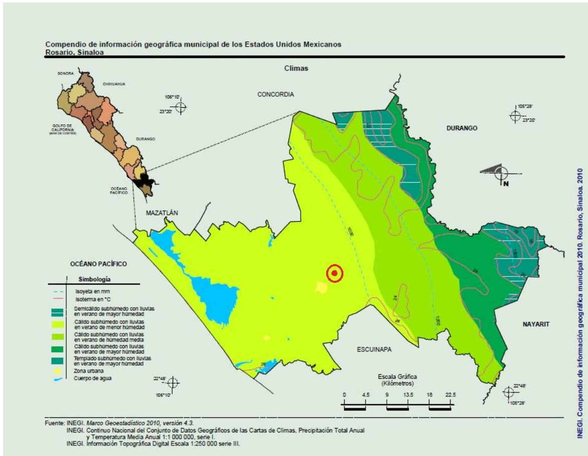
Imagen IV.13. Clima del Municipio de Rosario. INEGI.
