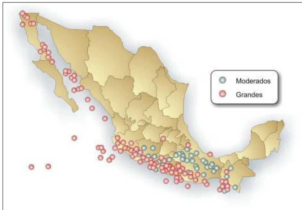
Imagen VI.17. Sismos moderados y grandes en México.
