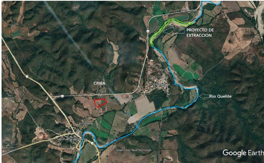
Imagen No. 16.- Imagen satelital de la ubicación de la criba en relación al proyecto.
