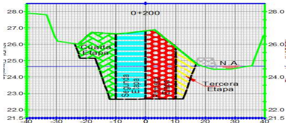
Imagen No. 7.- Sección de extracción típica.
