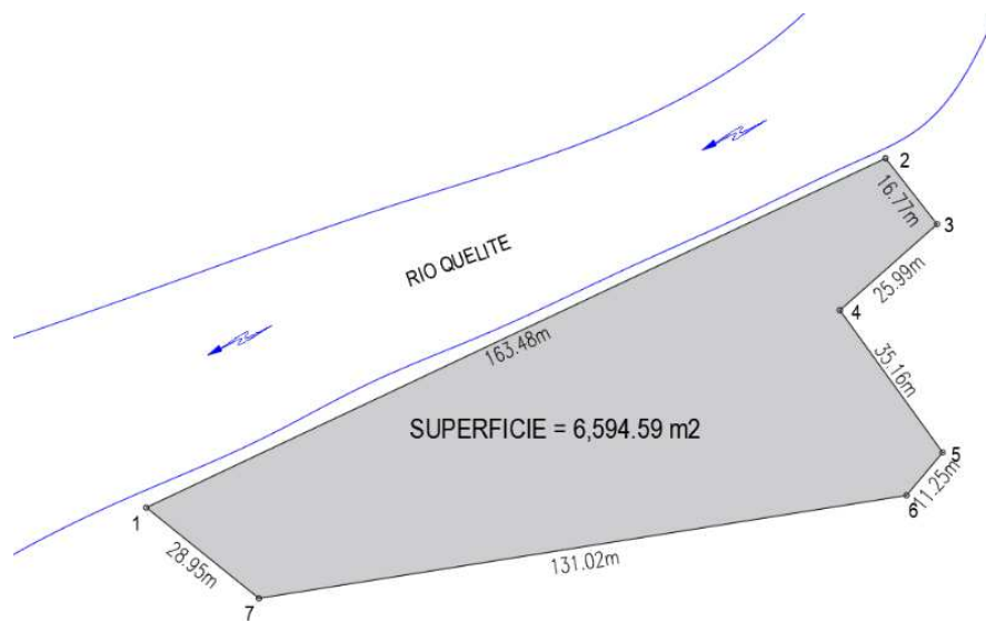
Imagen No. 42. Dimensiones área rescate y reubicación
