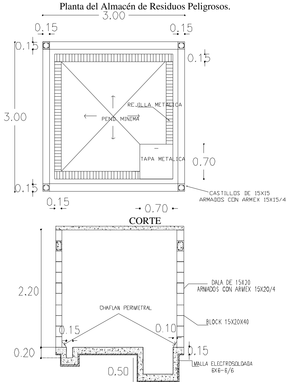
Imagen No. 12.- Diseño del almacén temporal de residuos peligrosos.
