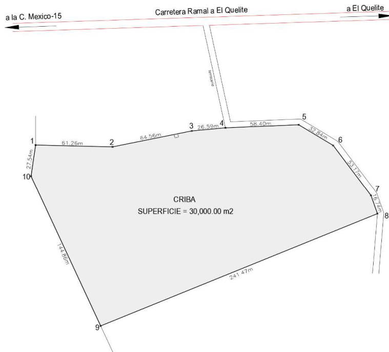
Imagen No. 18.- Dimensiones del polígono de la criba.
