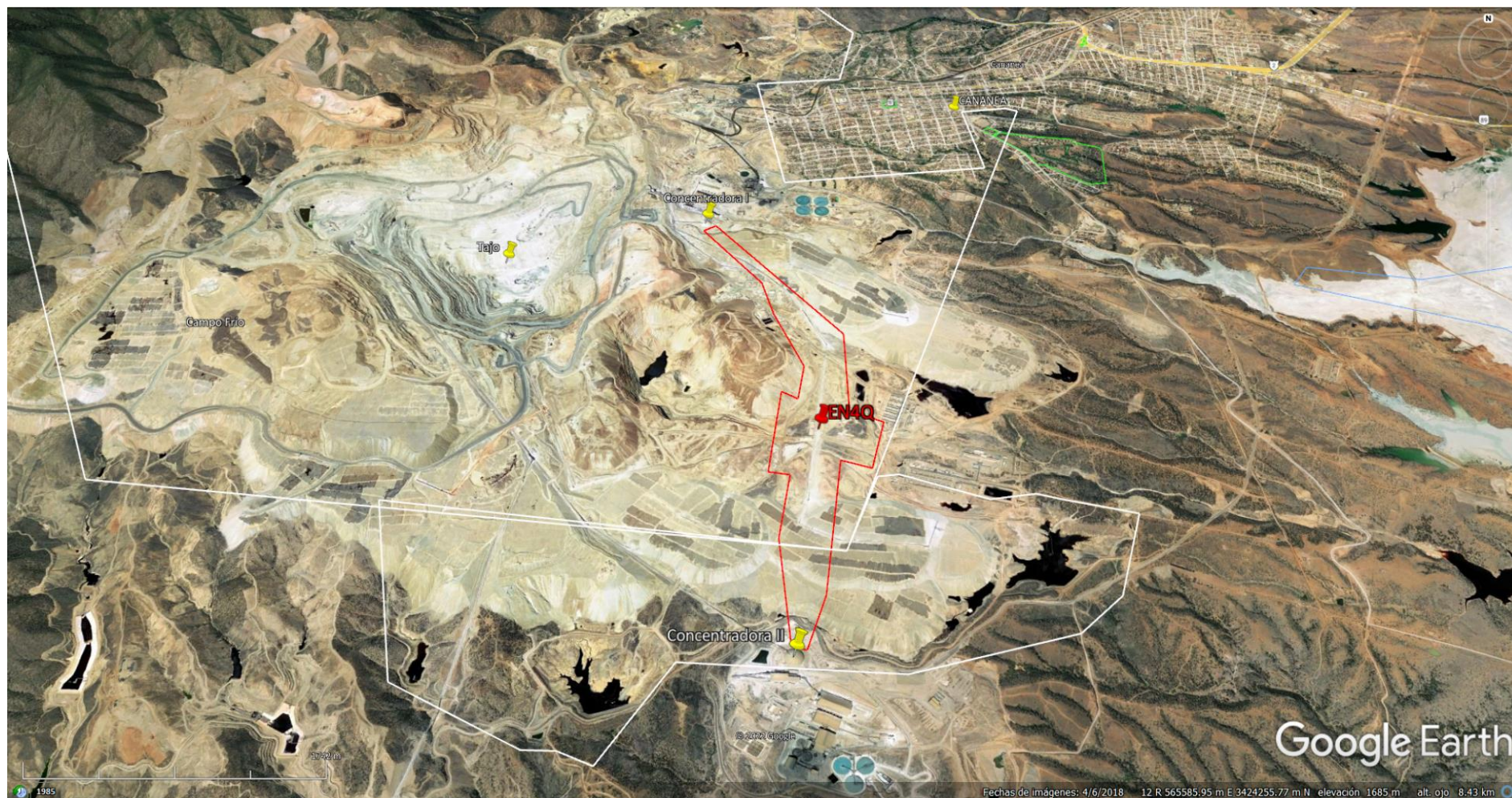
Figura II. 3. En rojo poligonal del predio del proyecto EP4Q, la marca de posición indica el sitio del nuevo edificio, desde ahí partirán las bandas hacia los domos de las Concentradoras I y II. La línea blanca delimita dos de los terrenos propiedad de Buenavista del Cobre donde se localizará el predio destinado al proyecto EP4Q
