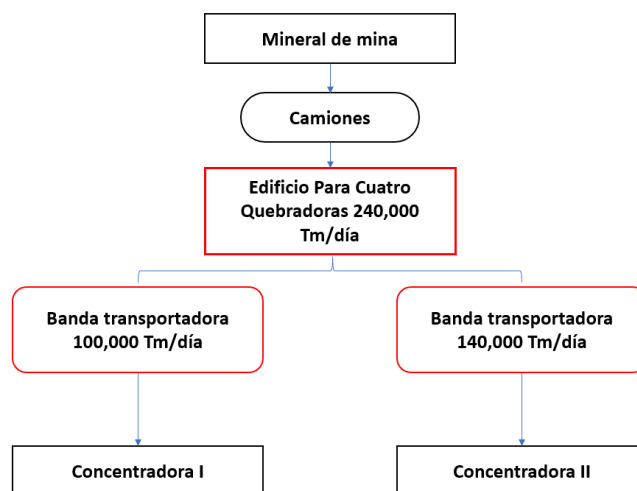
Figura II. 1. Diagrama de bloque del proyecto EP4Q. Con línea roja se representan los bloques de los componentes del proyecto.
