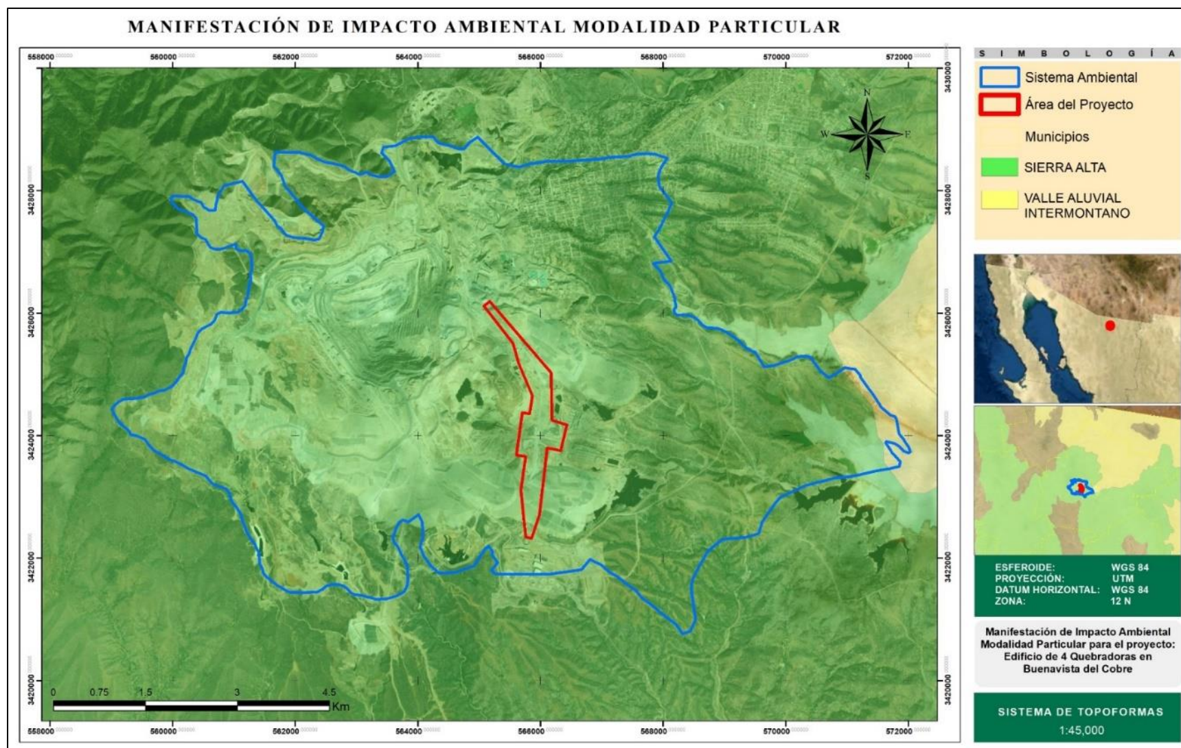
Figura IV. 13. Sistema de Topoformas presentes en el Sistema Ambiental
