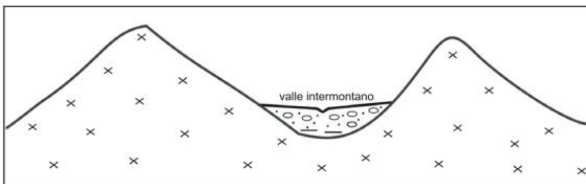
Figura IV. 10. Ejemplo de un valle intermontano aluvial.
