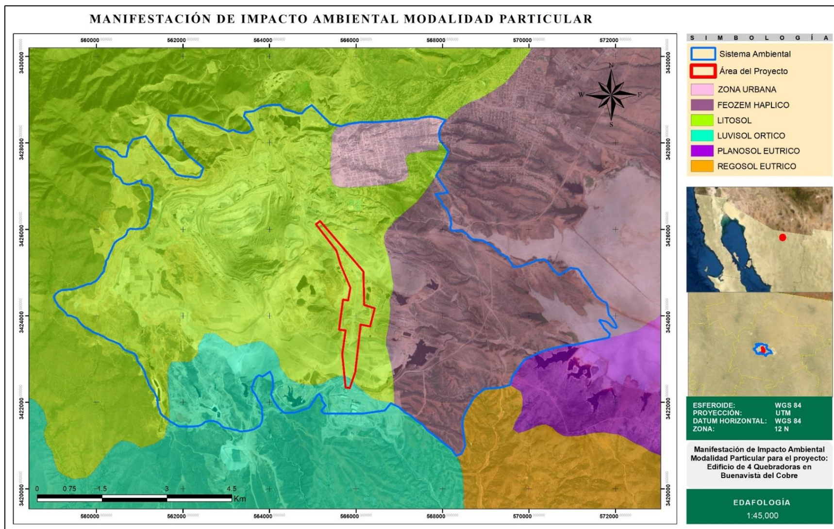
Figura IV. 15. Tipo de suelos presentes en el Sistema Ambiental
