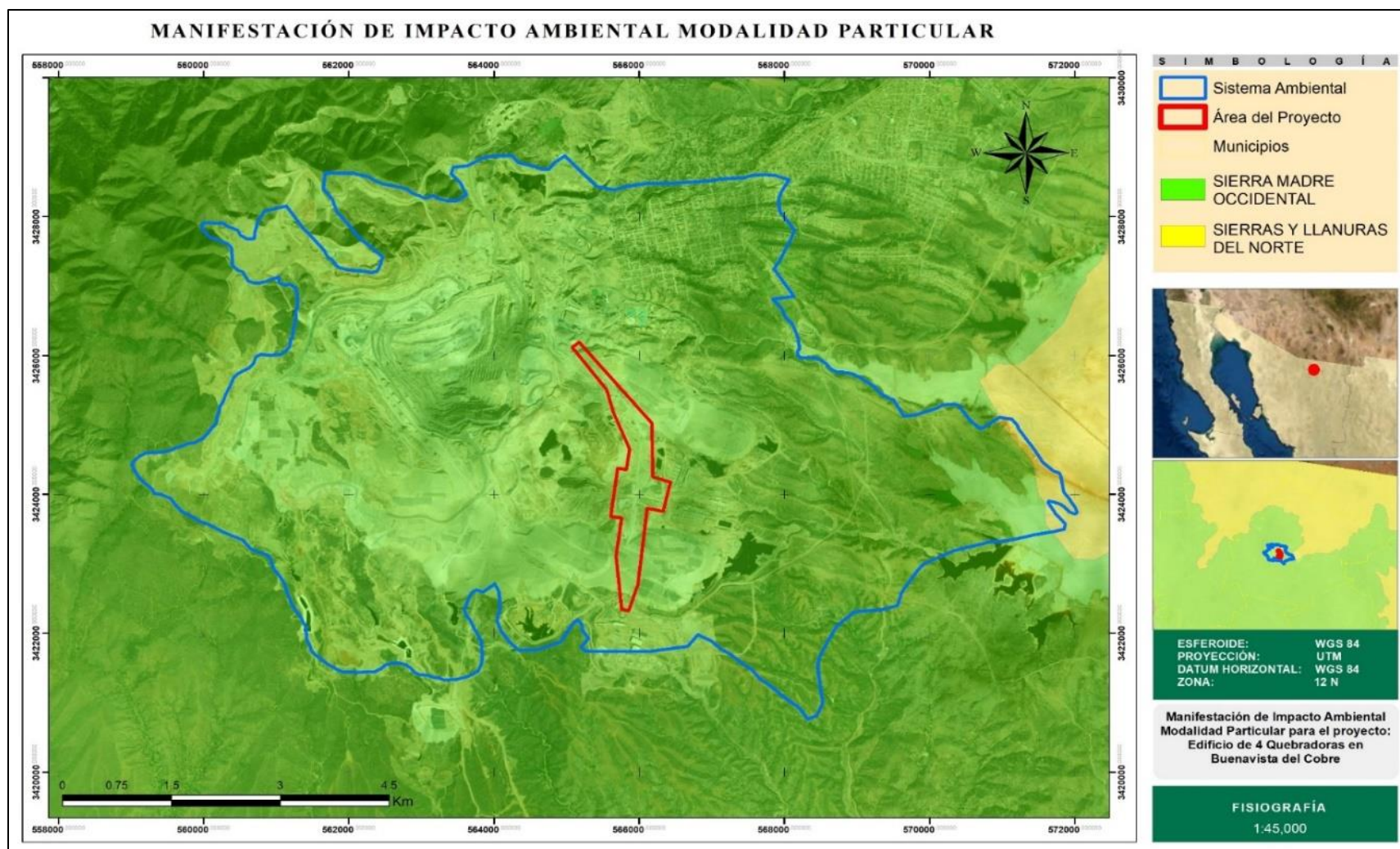
Figura IV. 11. Provincias Fisiográficas presentes en el Sistema Ambiental
