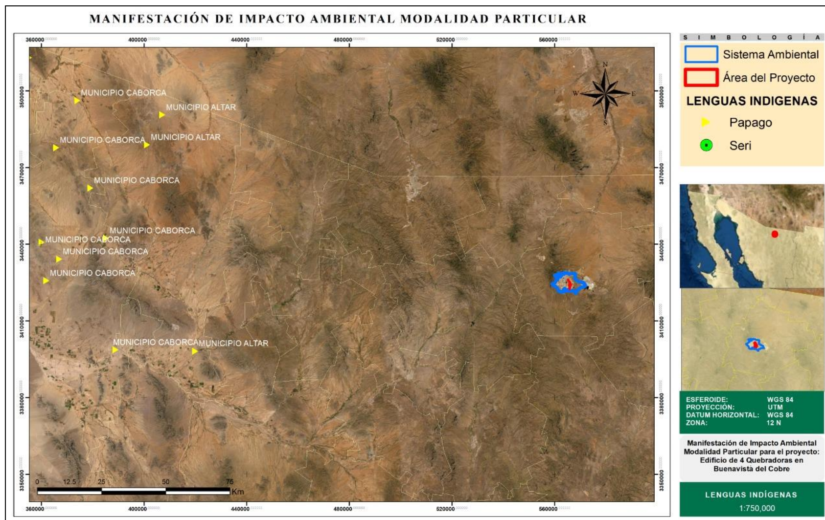
Figura III.2.- Presencia de zonas donde se hablan lenguas indígenas y presentan población Mayo-Yaqui.
