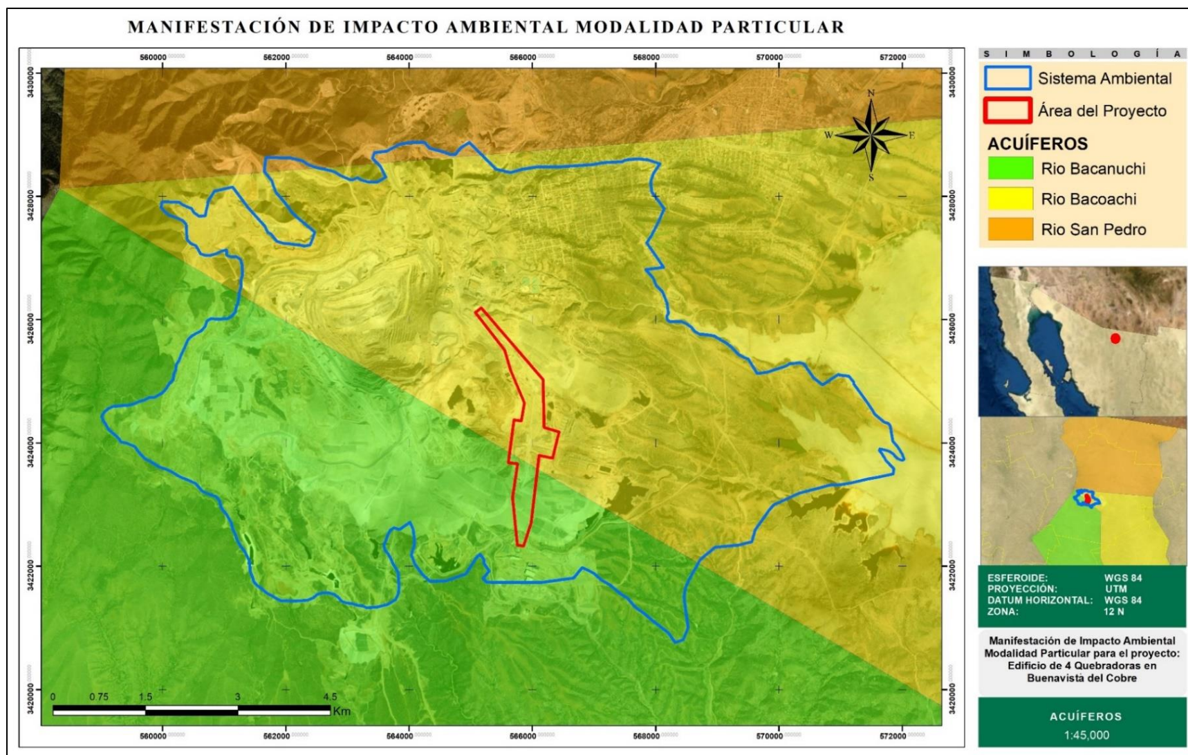
Figura IV. 19. Sistema de Acuíferos presentes en el Sistema Ambiental
