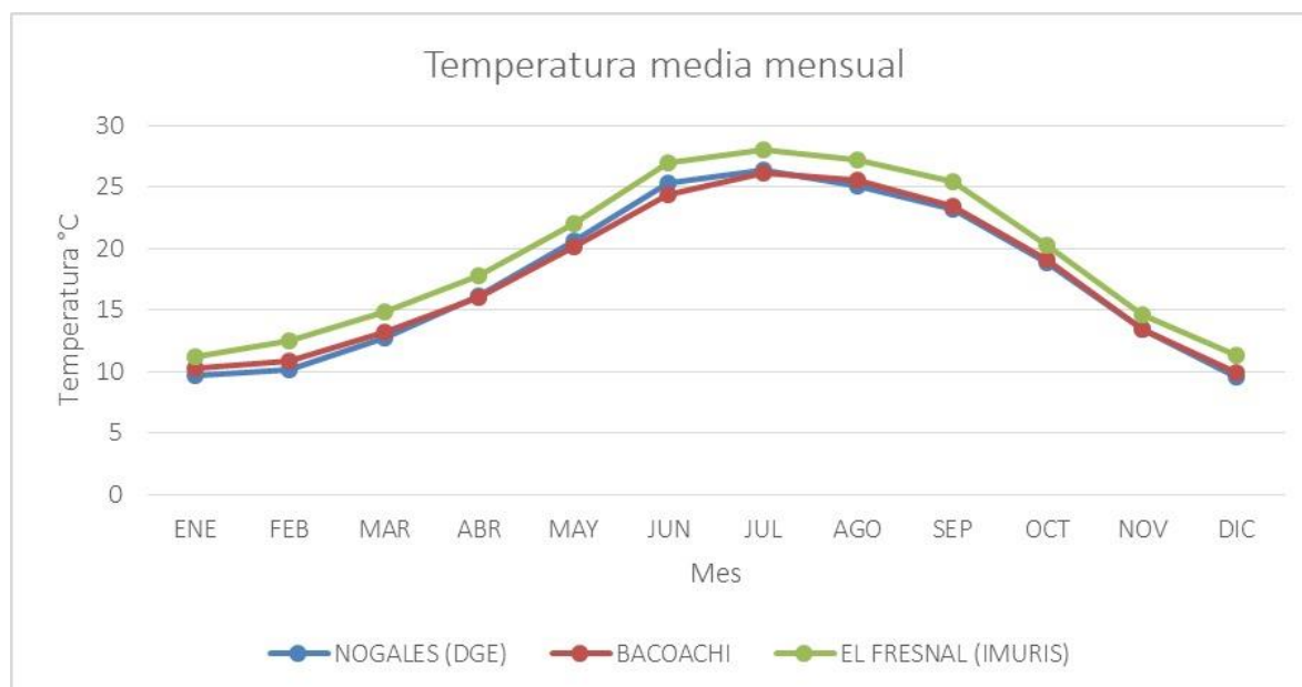
Figura IV. 4. Gráfica de comportamiento de la temperatura de las estaciones meteorológicas.
