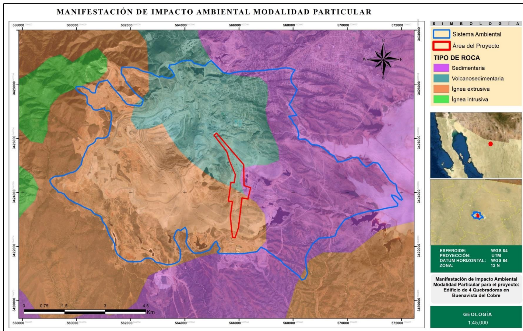
Figura IV.14. Tipos de rocas presentes en el Sistema Ambiental
