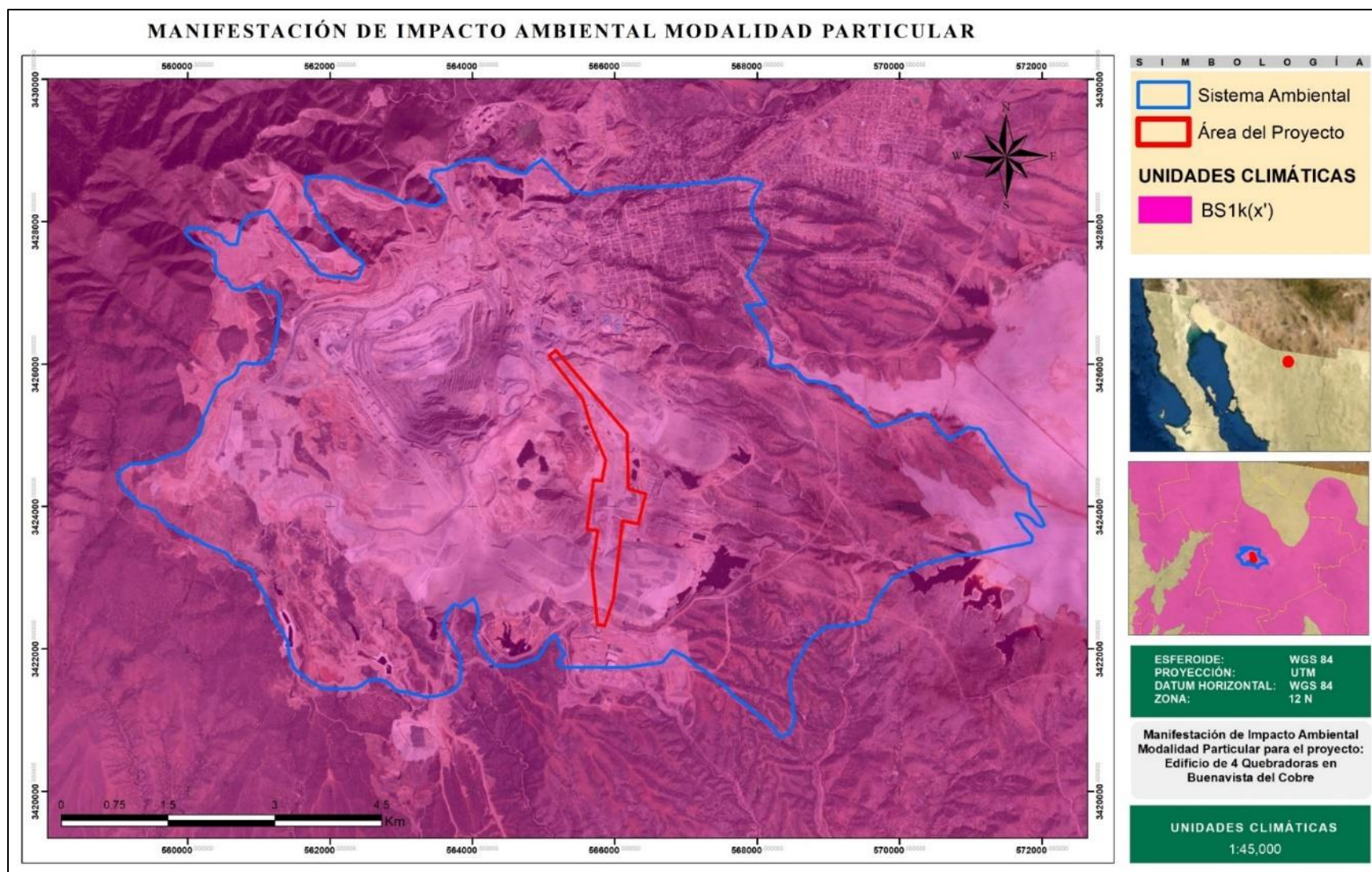
Figura IV. 3. Unidades climáticas en el Sistema Ambiental
