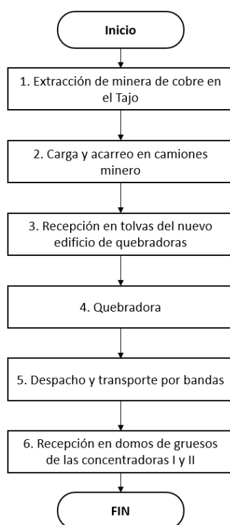
Figura II. 7. Diagrama de bloques para el proceso que se realizará en el proyecto EP4Q.
