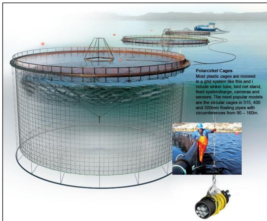
Imagen 14. Diagrama general de jaula marina circular.
