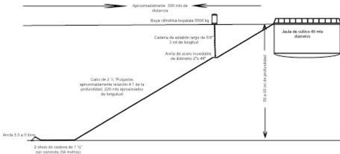
Imagen 18. Sistema de anclaje para las jaulas de cultivo.
