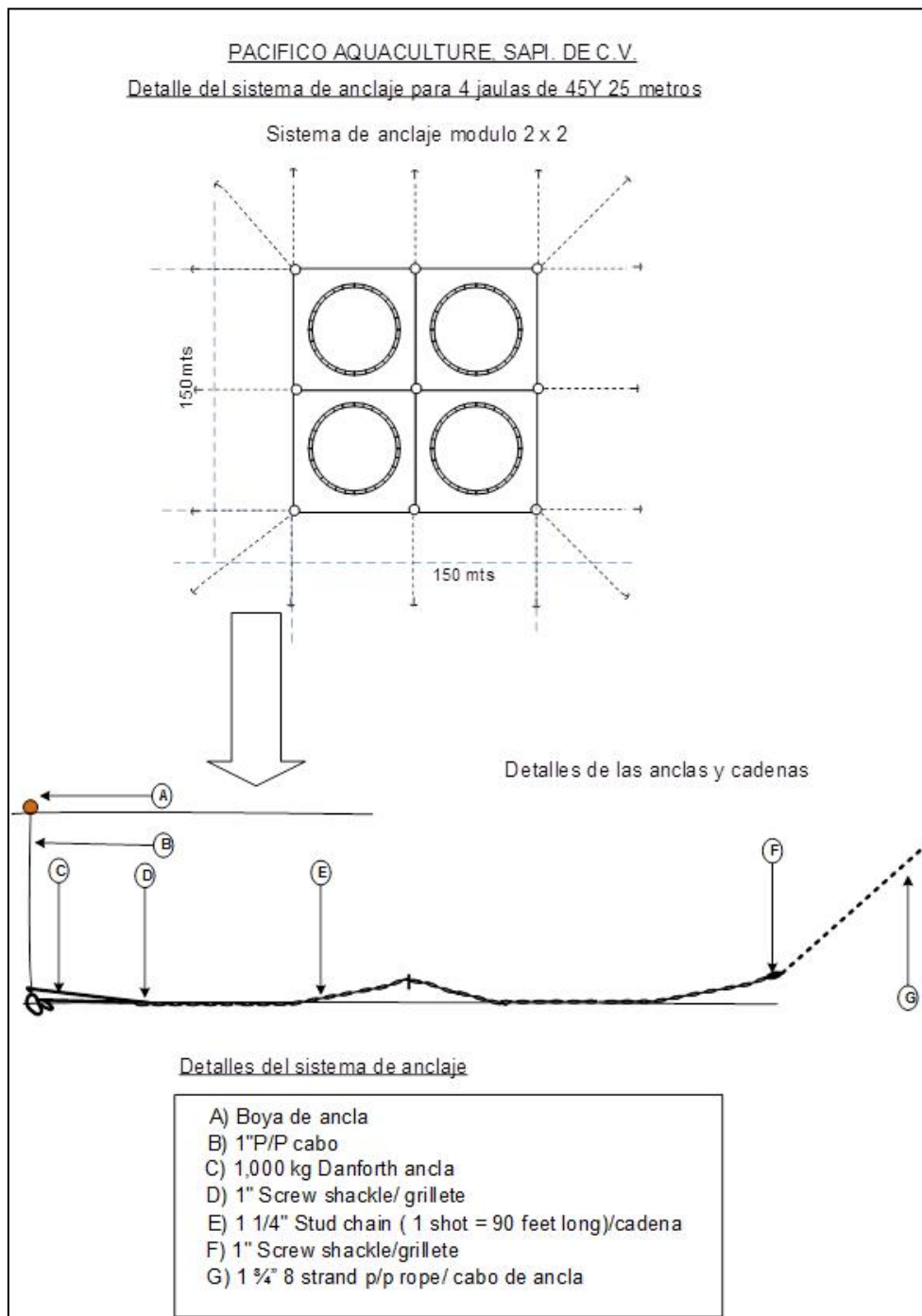
Imagen 16. Diseños de sistemas de anclaje, así como la distribución para las estas.
