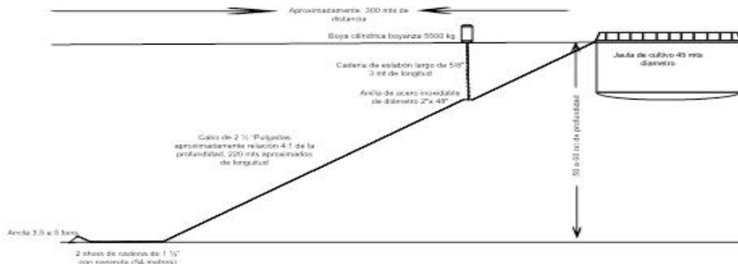
Imagen 4. Representación de un sistema de anclaje y sus dimensiones.
