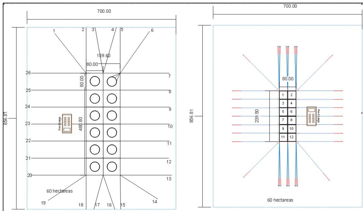
Imagen 17. Distribución de los módulos de utilizar jaulas circulares (izquierda) o de utilizar jaulas cuadradas (derecha), las jaulas de 8x8x10 mts, estarían situadas dentro de las jaulas de mayor tamaño para protección.
