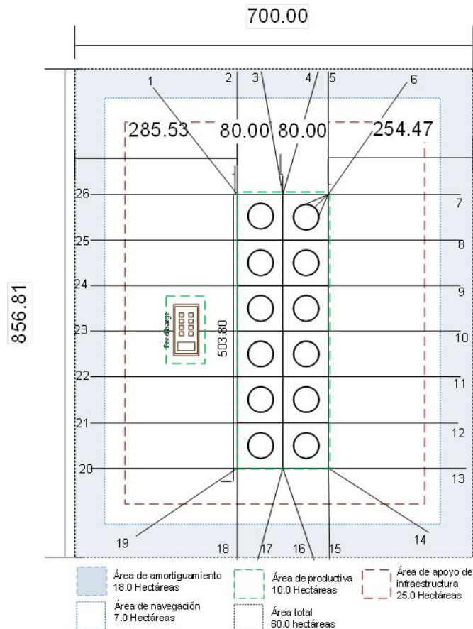
Imagen 3. Representación de un módulo de cultivo y sistema de anclaje, con sus dimensiones.
