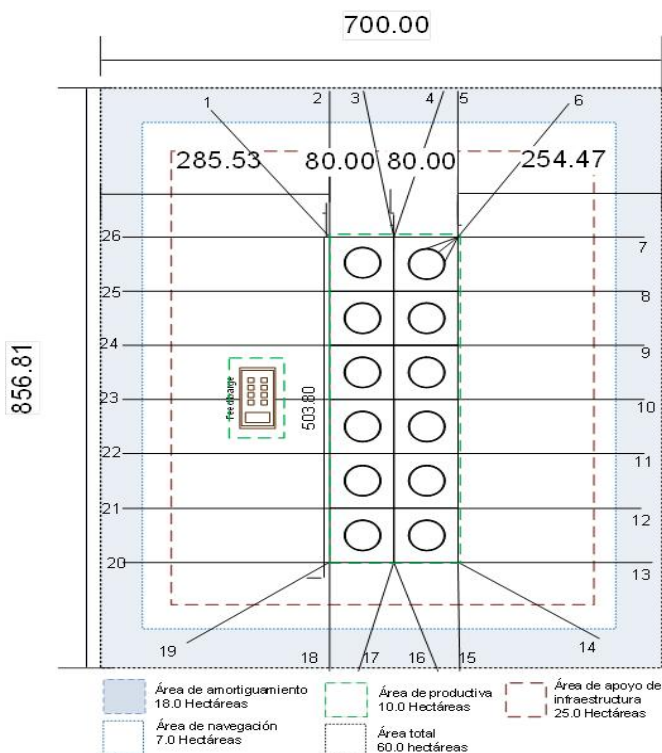
Imagen 3. Representación de un módulo de cultivo y sistema de anclaje, con sus dimensiones.
