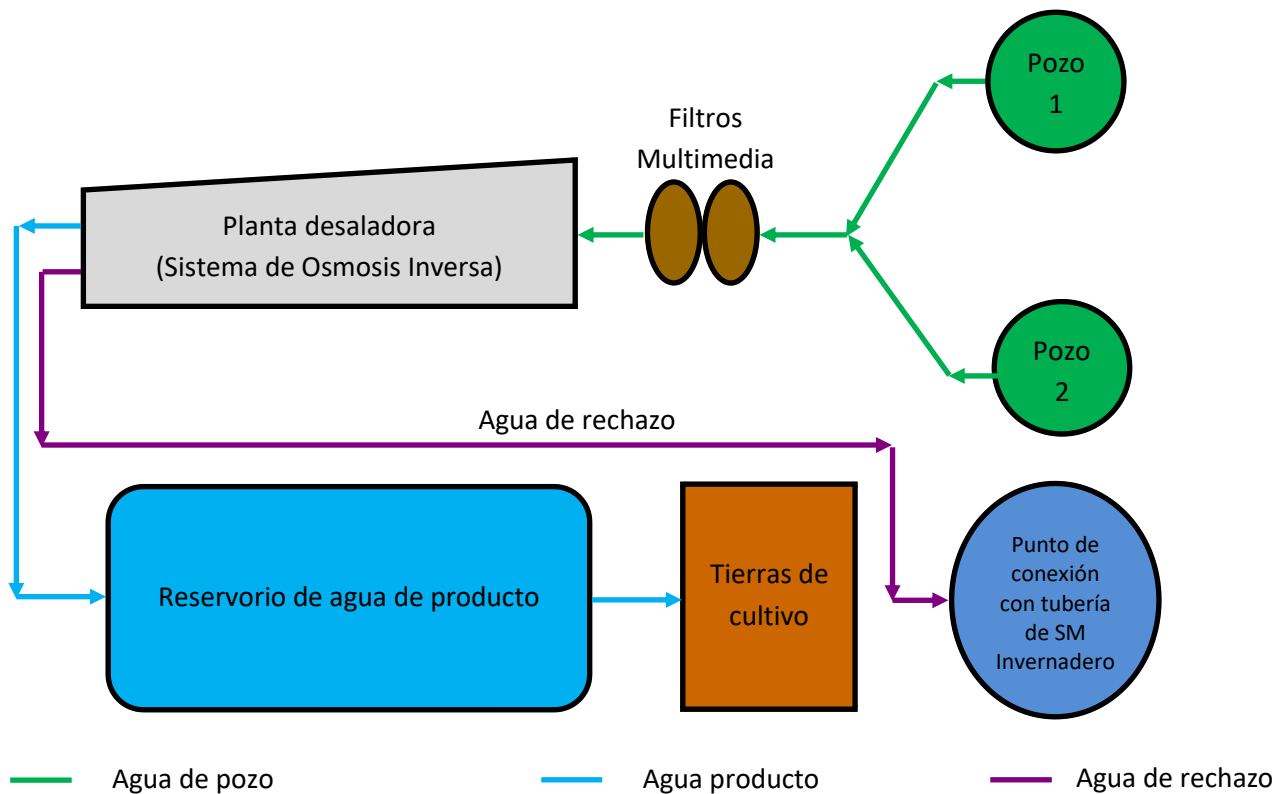
Figura 7. Diagrama de flujo del agua desde su extracción, tratamiento, uso y su punto conexión.
