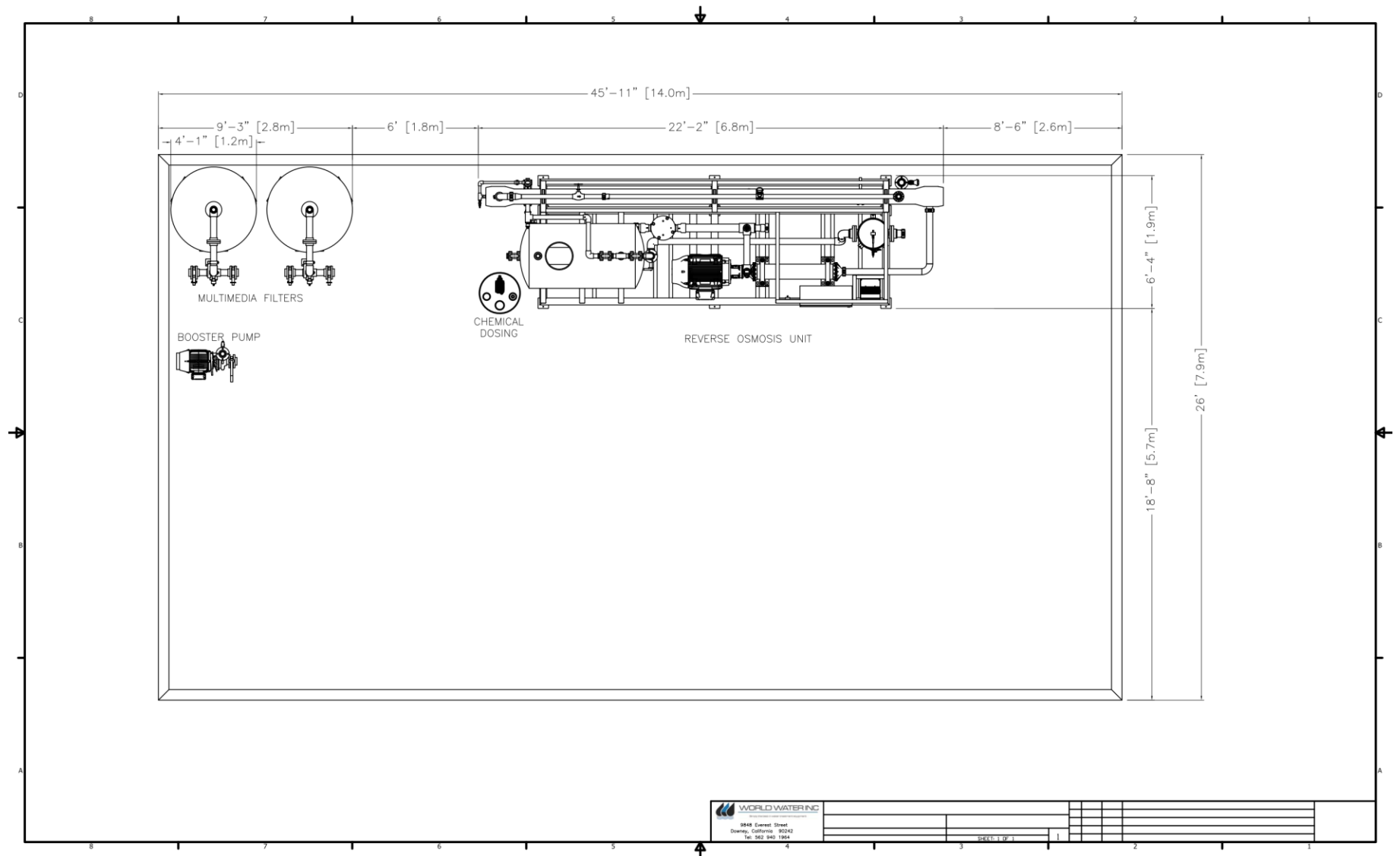
Figura 6. Diagrama del sistema de osmosis inversa que se planea instalar para este proyecto.
