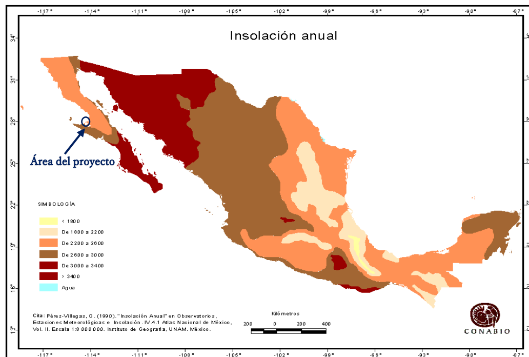
Figura 31. Insolación anual en el territorio mexicano (en horas). Pérez-Villegas, 1990
