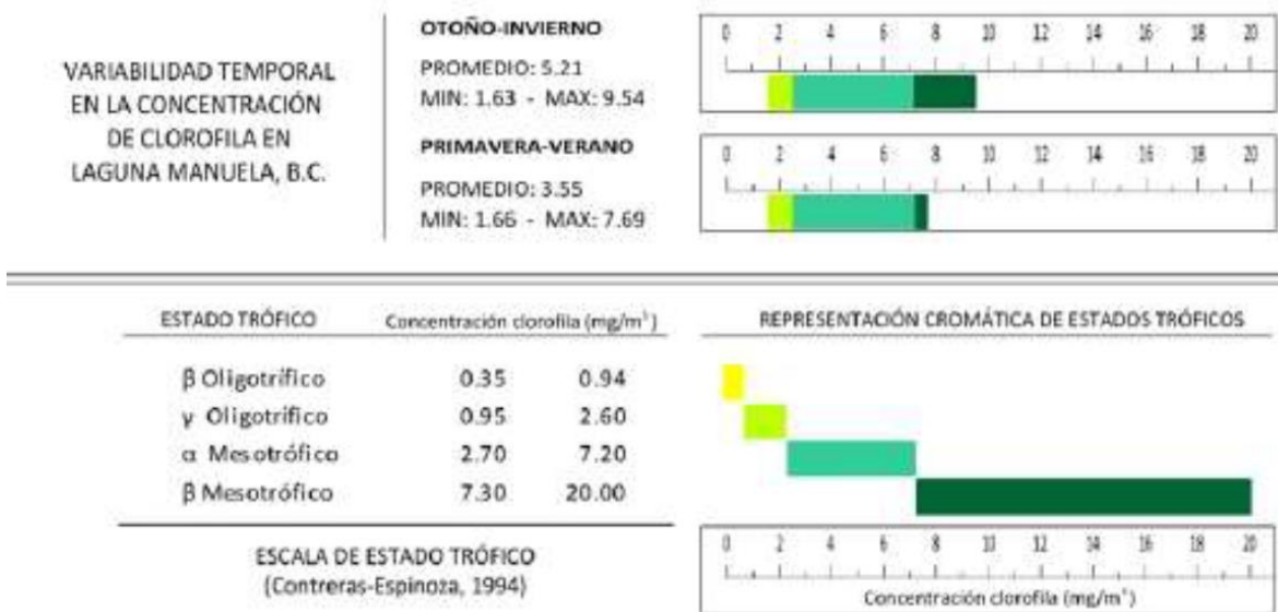
Figura 50. Variabilidad del estado trófico de Laguna Manuela, B.C., con referencia a la clasificación de Contreras-Espinoza, (1994). Fuente: Arano et al., (2011).
