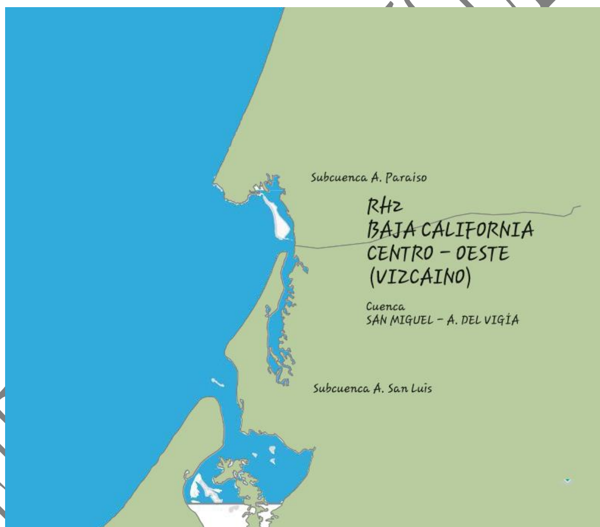
Figura 38. Región Hidrológica, Cuenca y subcuencas que desembocan en el área del proyecto
