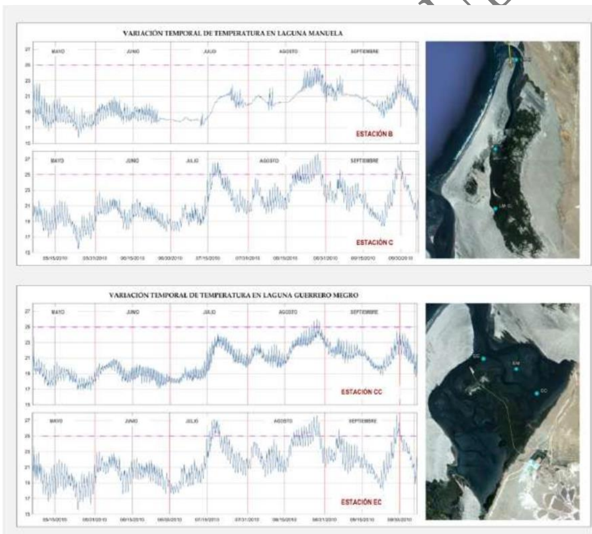
Figura 43. Variaciones de corto y mediano plazo registradas en la temperatura de fondo (°C) para estaciones localizadas en la zonas de las bocas de intercomunicación y cabeceras de las lagunas Manuela (arriba) y Guerrero Negro durante el periodo verano-otoño de 2010. Fuente: Arano, et al., 2010.
