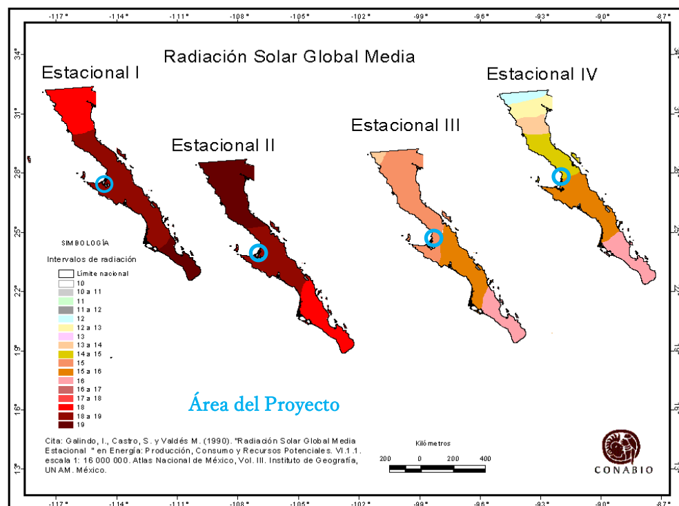
Figura 30. Radiación solar global media estacional I (primavera), II (verano), III (otoño) y IV (invierno)
