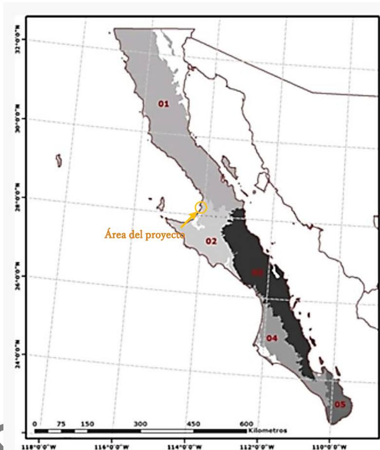
Figura 36. Provincia Península de Baja California. 01: Subprovincia Sierras de Baja California Norte; 02: Discontinuidad Desierto de San Sebastián Vizcaíno; 03: Subprovincia Sierra de La Giganta; 04: Discontinuidad Llanos de Magdalena; 05: Discontinuidad Región del Cabo
