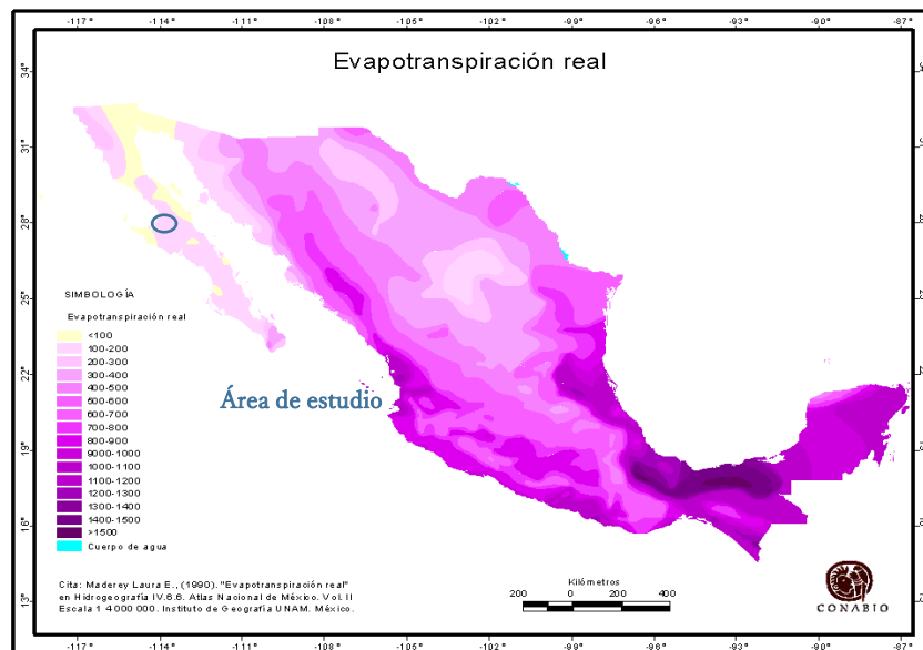
Figura 33. Evapotranspiración real de México (CONABIO, 2006)
