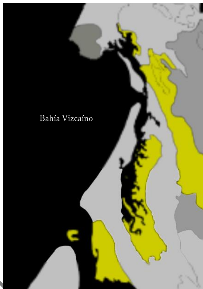
Figura 37. Tipos de suelo en el entorno al área del proyecto. En amarillo Solonchak, Ceniza claro: Arenosol y Ceniza oscuro: regosol. En otros colores, otros suelos
