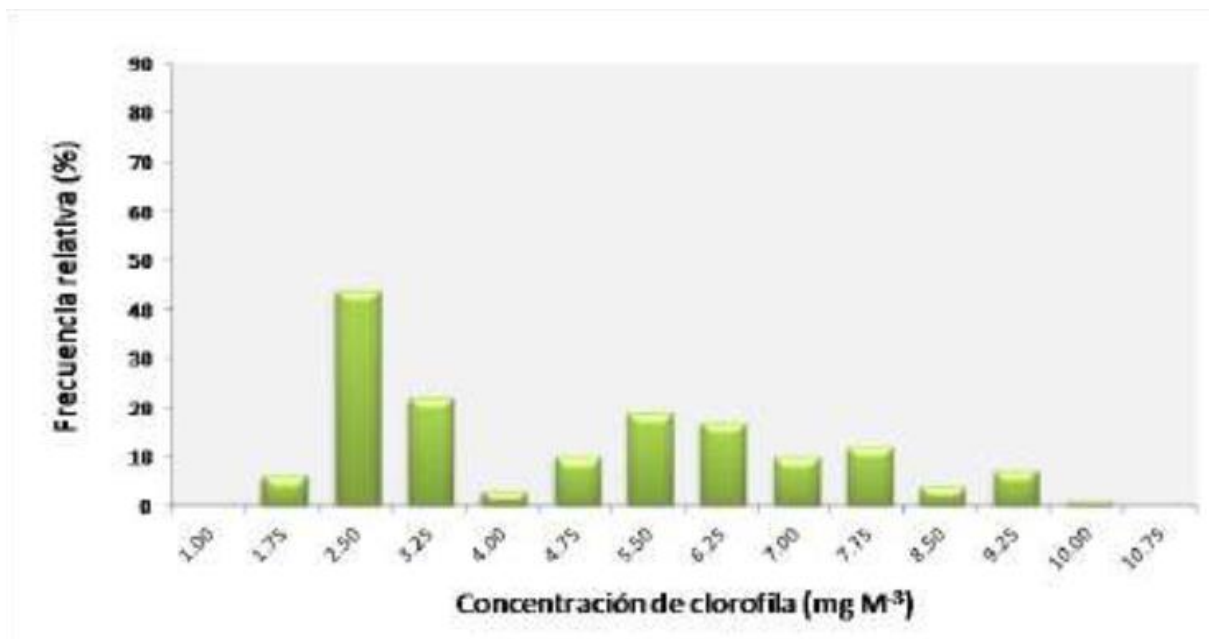
Figura 49. Distribución de frecuencia de las concentraciones de clorofila registradas del análisis del total de las muestras colectadas en Laguna Manuela durante las series de tiempo ( n=155 ).
