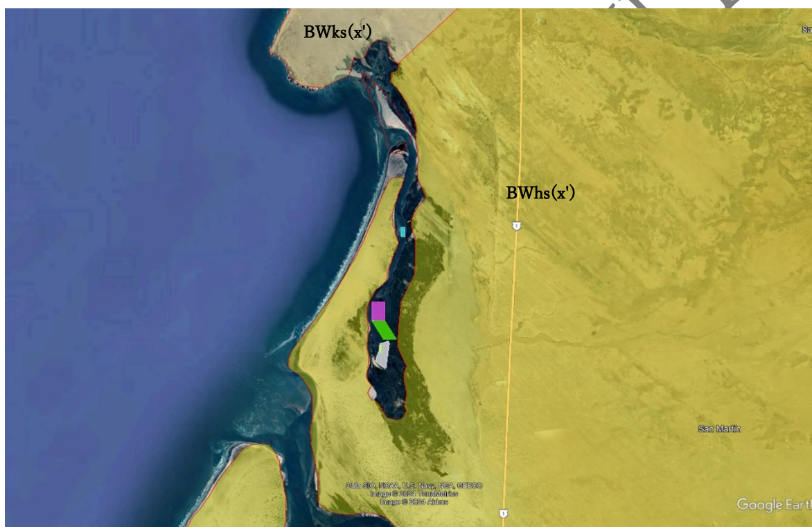
Figura 28. Localización del proyecto según el clima
