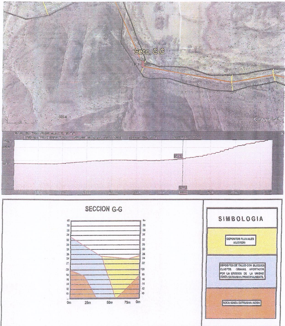
Fig.-14) Terminado el análisis del ambiente geológico, se procedió a realizar las secciones que se indican en Fig.-7, obteniendo como resultado la distribución de las unidades de materiales identificadas en campo, mostrándose en la presente figura, los resultados obtenidos en la sección G-G
