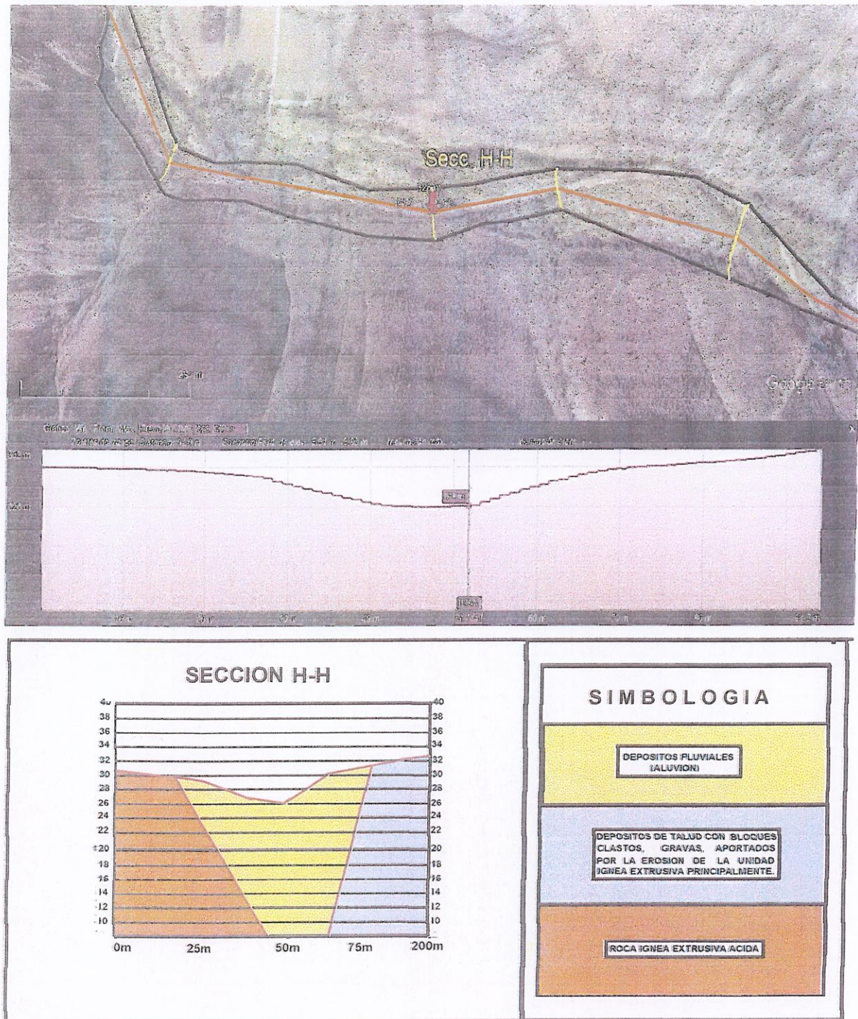
Fig.-15) Terminado el análisis del ambiente geológico, se procedió a realizar las secciones que se indican en Fig.-7, obteniendo como resultado la distribución de las unidades de materiales identificadas en campo, mostrándose en la presente figura, los resultados obtenidos en la sección H-H
