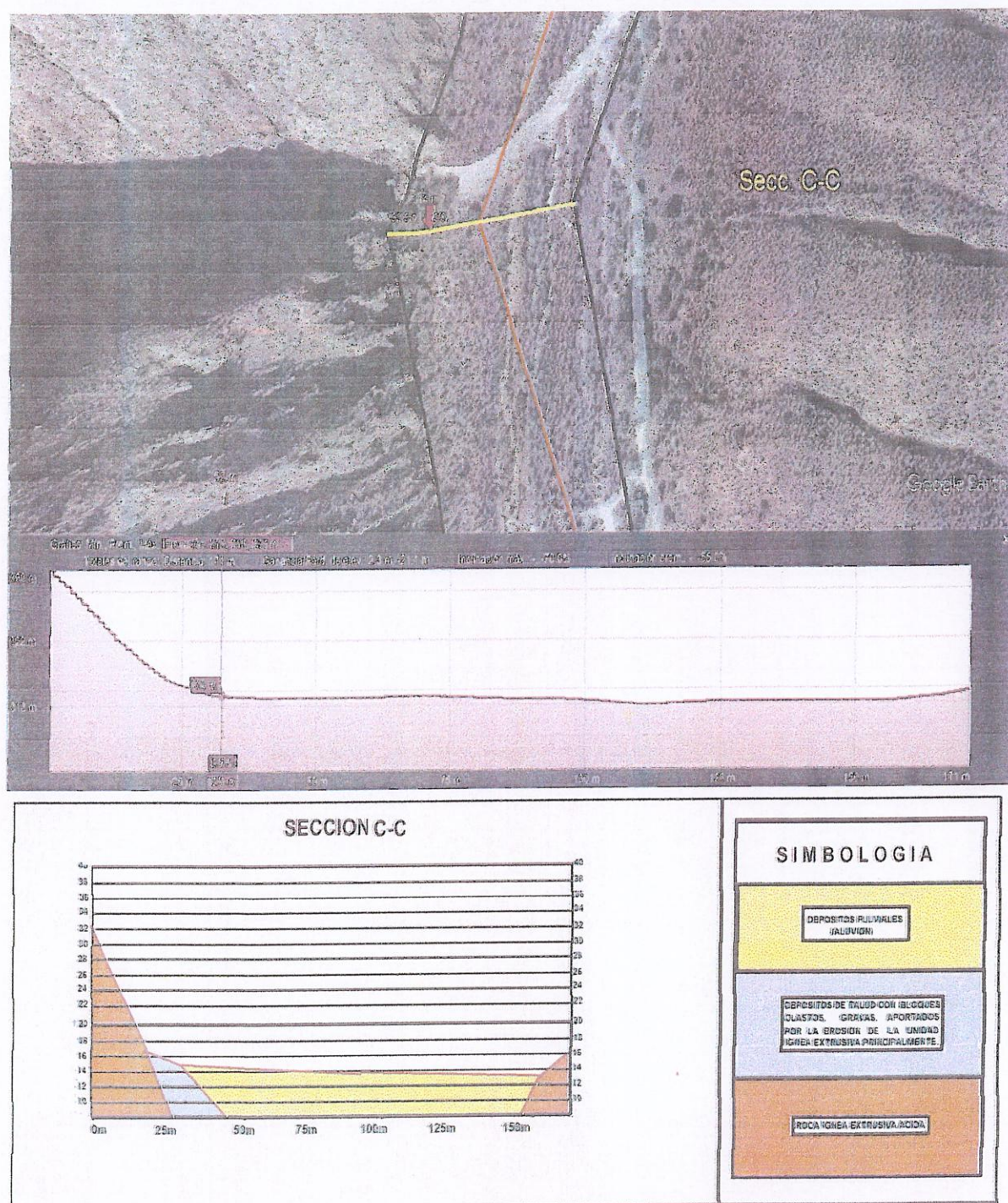
Fig.-10) Terminado el análisis del ambiente geológico, se procedió a realizar las secciones que se indican en Fig.-7, obteniendo como resultado la distribución de las unidades de materiales identificadas en campo, mostrándose en la presente figura, los resultados obtenidos en la sección C-C
