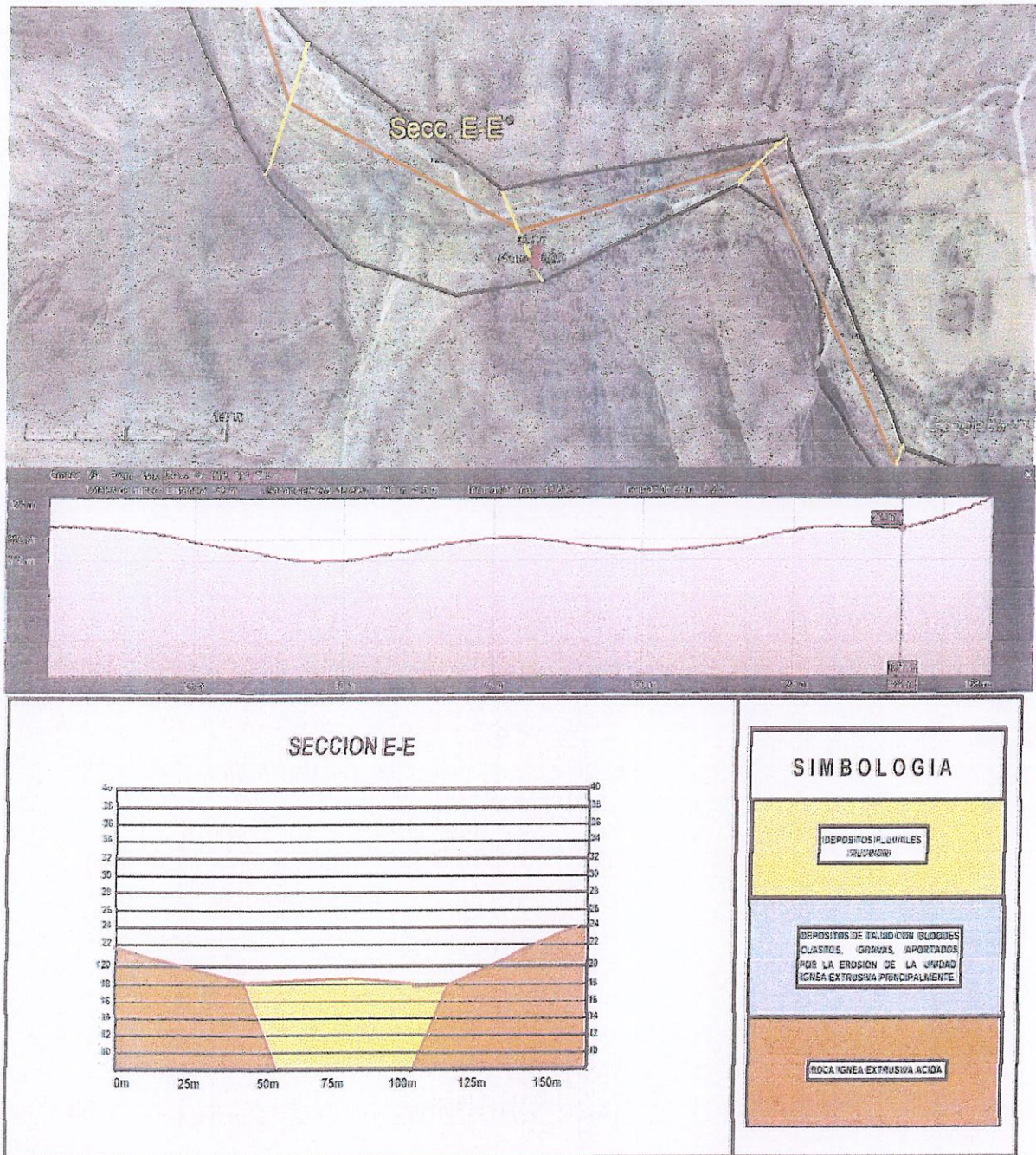
Fig.-12) Terminado el análisis del ambiente geológico, se procedió a realizar las secciones que se indican en Fig.-7, obteniendo como resultado la distribución de las unidades de materiales identificadas en campo, mostrándose en la presente figura, los resultados obtenidos en la sección E-E.
