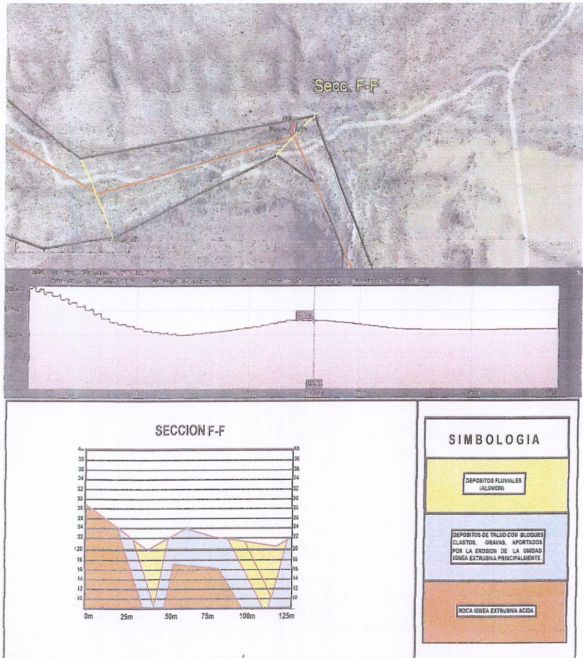
Fig.-13) Terminado el análisis del ambiente geológico, se procedió a realizar las secciones que se indican en Fig.-7, obteniendo como resultado la distribución de las unidades de materiales identificadas en campo, mostrándose en la presente figura, los resultados obtenidos en la sección F-F
