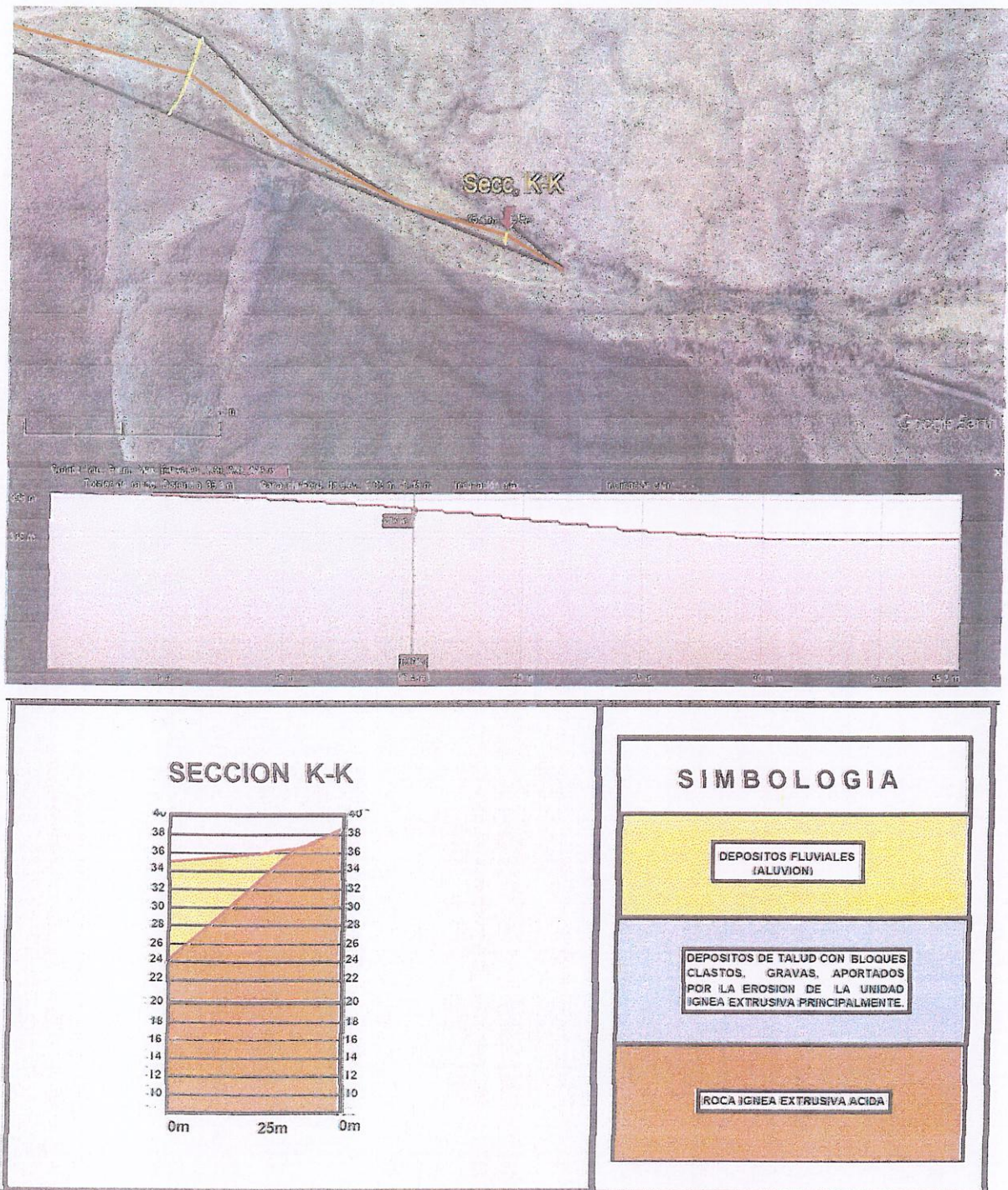
Fig.-18) Terminado el análisis del ambiente geológico, se procedió a realizar las secciones que se indican en Fig.-7, obteniendo como resultado la distribución de las unidades de materiales identificadas en campo, mostrándose en la presente figura, los resultados obtenidos en la sección K-K
