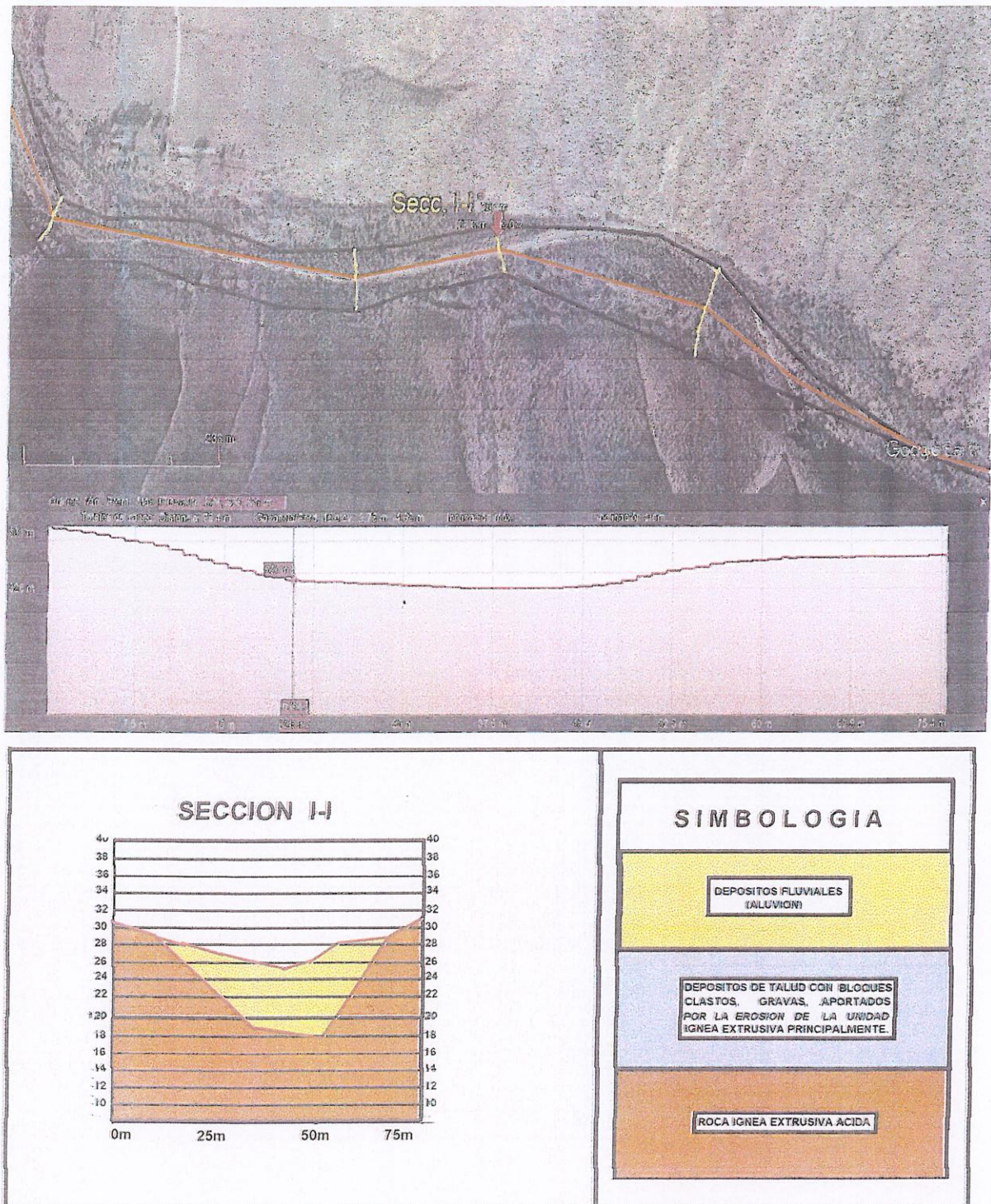
Fig.-16) Terminado el análisis del ambiente geológico, se procedió a realizar las secciones que se indican en Fig.-7, obteniendo como resultado la distribución de las unidades de materiales identificadas en campo, mostrándose en la presente figura, los resultados obtenidos en la sección I-I
