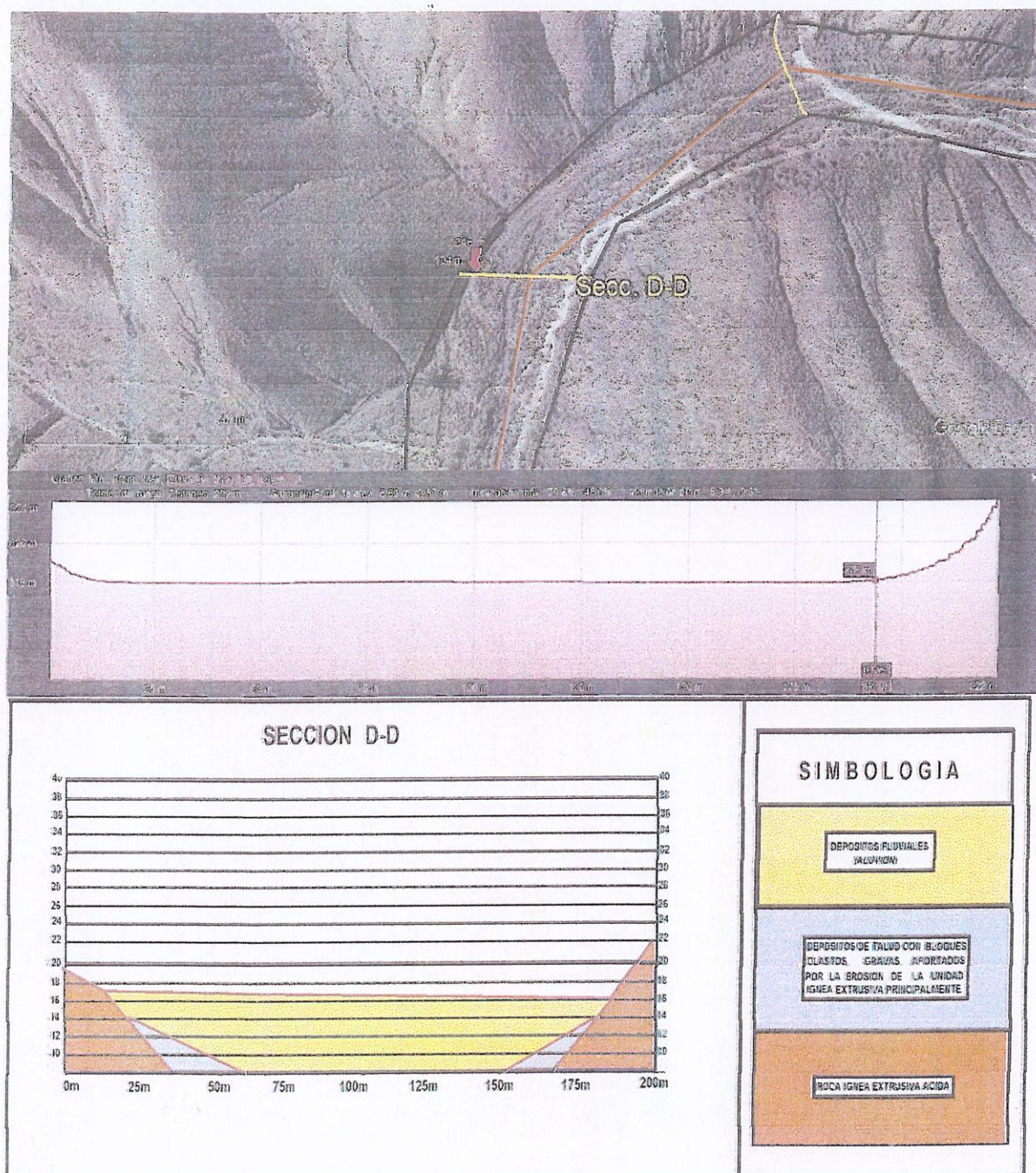
Fig.-11) Terminado el análisis del ambiente geológico, se procedió a realizar las secciones que se indican en Fig.-7, obteniendo como resultado la distribución de las unidades de materiales identificadas en campo, mostrándose en la presente figura, los resultados obtenidos en la sección D-D
