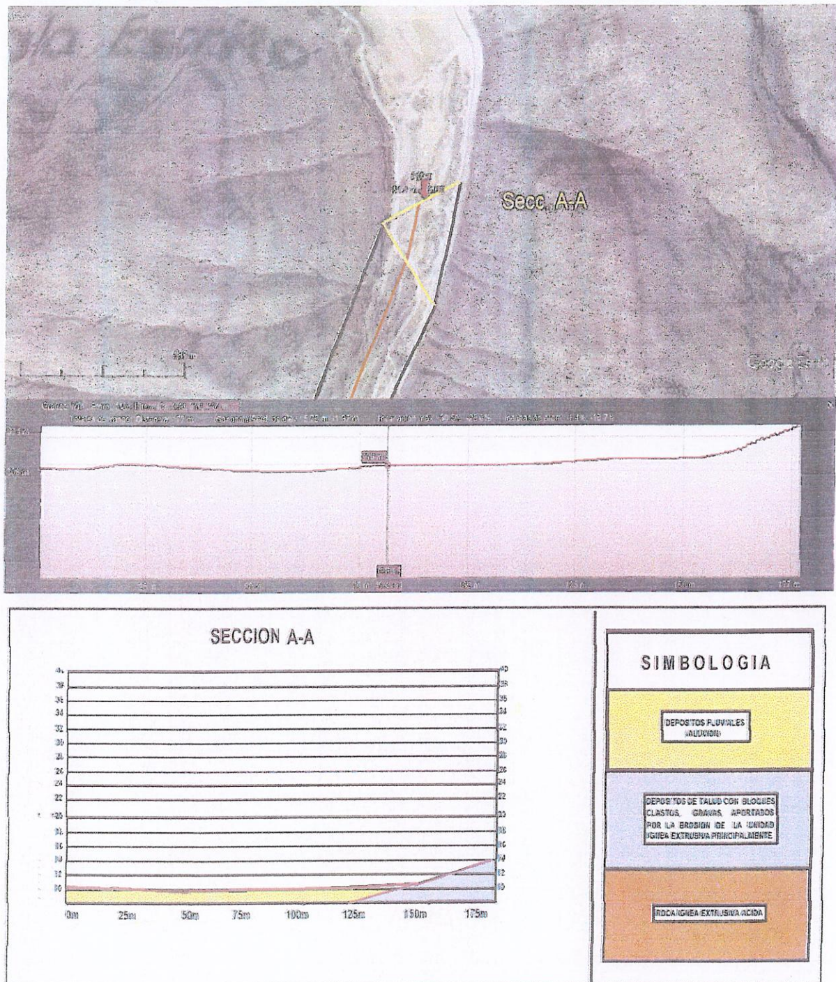
Fig.-8) Terminado el análisis del ambiente geológico, se procedió a realizar las secciones que se indican en Fig.-7, obteniendo como resultado la distribución de las unidades de materiales identificadas en campo, mostrandoce en la presente figura, los resultados obtenidos en la sección A.-A
