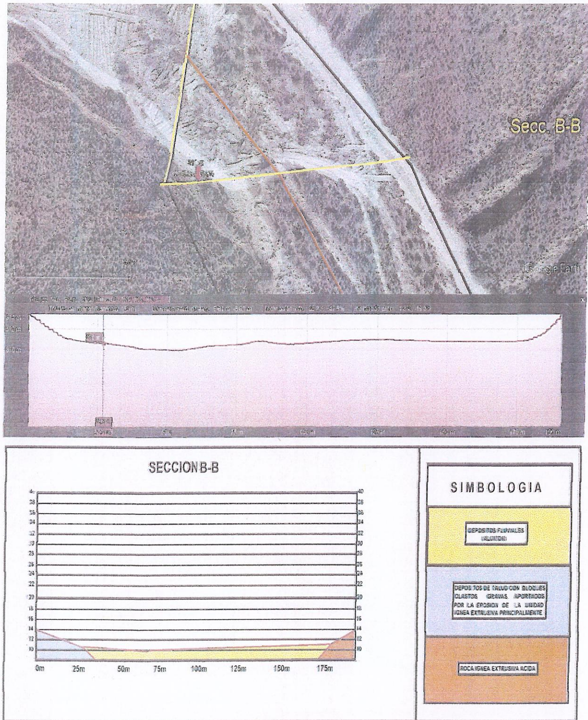
Fig.-9) Terminado el análisis del ambiente geológico, se procedió a realizar las secciones que se indican en Fig.-7, obteniendo como resultado la distribución de las unidades de materiales identificadas en campo, mostrando en la presente figura, los resultados obtenidos en la sección B-B.
