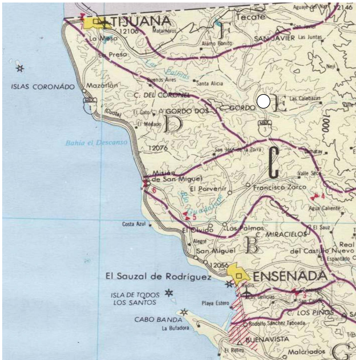
Carta Hidrológica Superficial del Estado INEGI (escala 1:1,000,000). El círculo blanco encierra la zona de estudio.
