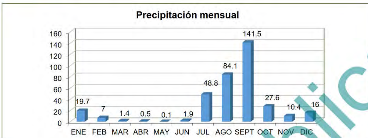
Figura IV-4. Representación gráfica de la precipitación mensual que se registra en la estación más cercana a la superficie requerida para el Proyecto.
