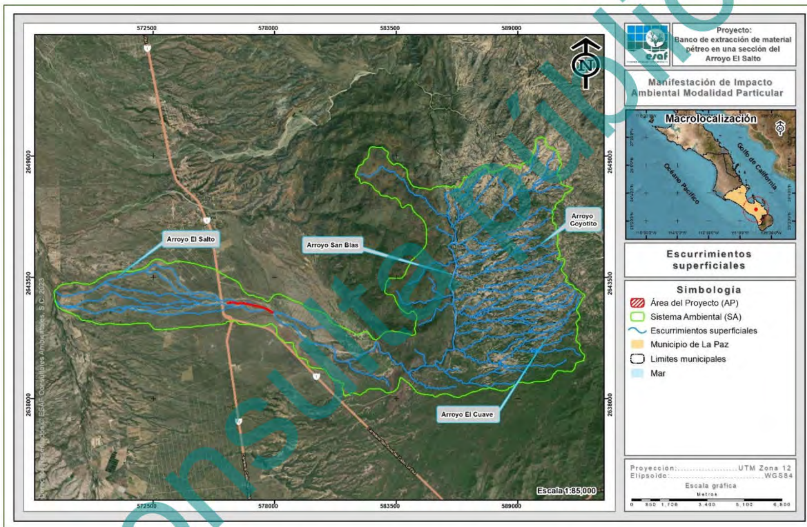
Figura IV-13. Hidrología superficial del SA donde se ubica el Proyecto.
