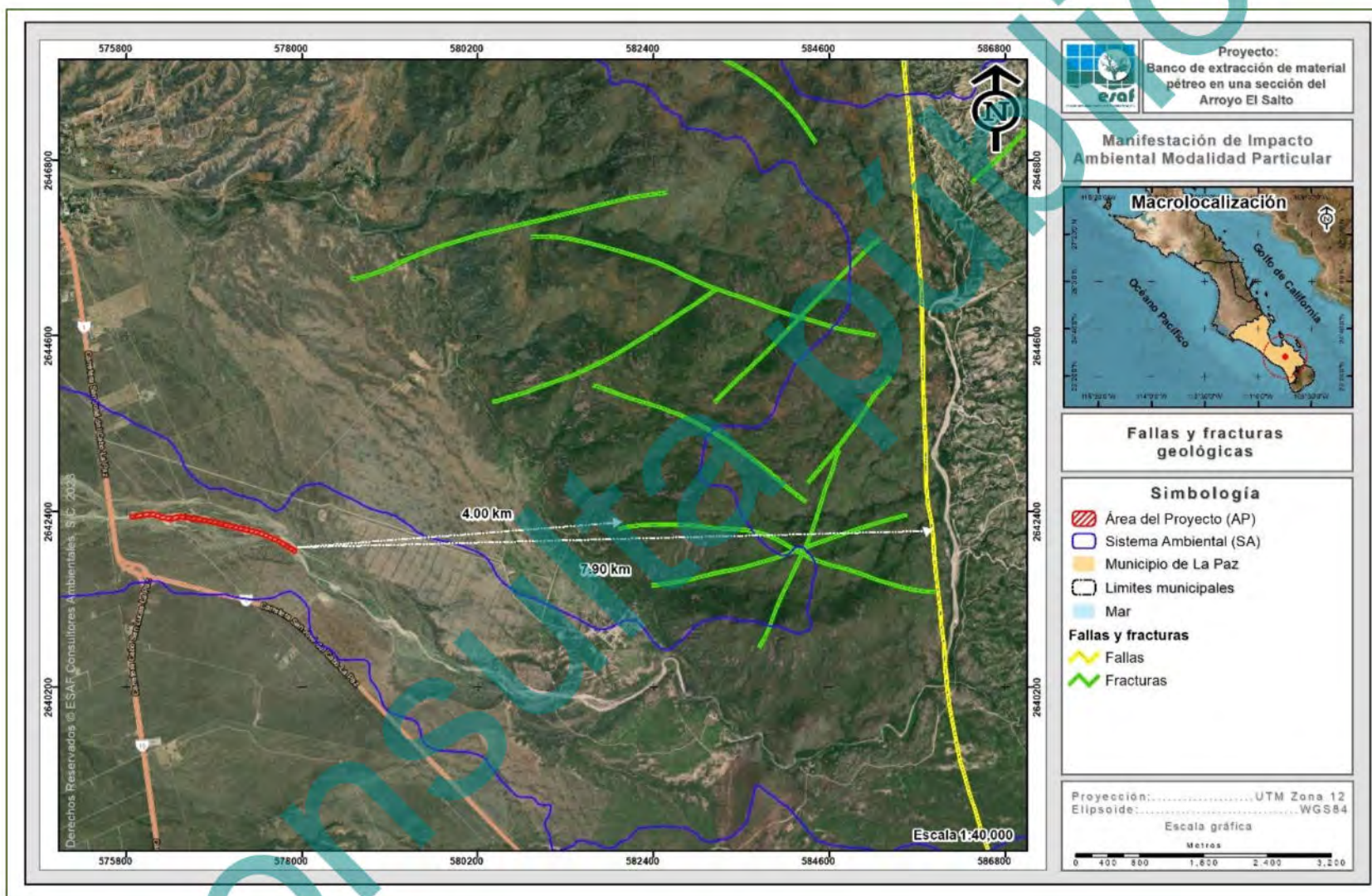
Figura IV-7. Ubicación del AP con respecto al sistema de fallas y zona de fracturación más cercana.
