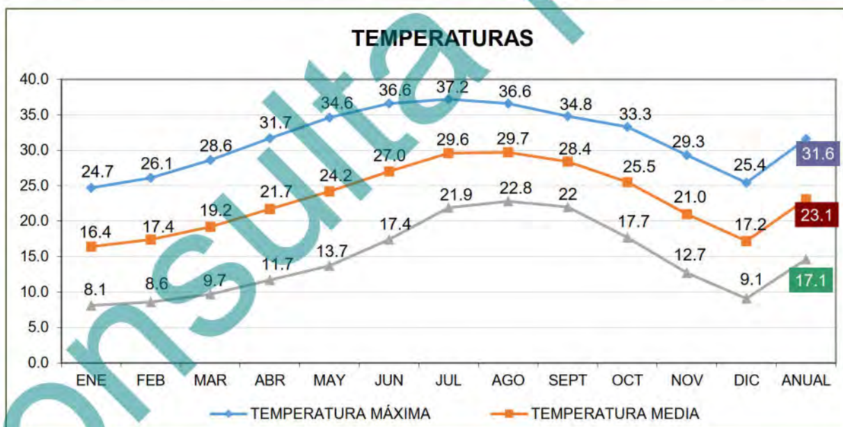
Figura IV-5. Representación gráfica de la temperatura que se registra en la estación más cercana al área del Proyecto.
