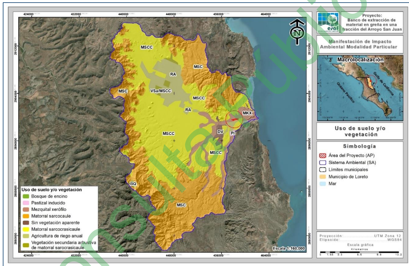
Figura IV-12. Tipos de uso de suelo y vegetación para el SA donde se ubica el proyecto.
