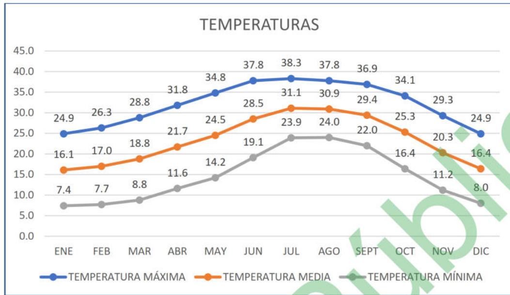
Figura IV-3. Información de la temperatura que se registra dentro del área donde se desarrollará el presente proyecto.
