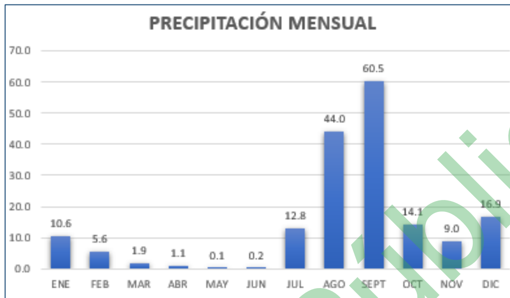
Figura IV-4. Diagrama de precipitación que se registra en la estación climatológica más cercana al AP.
