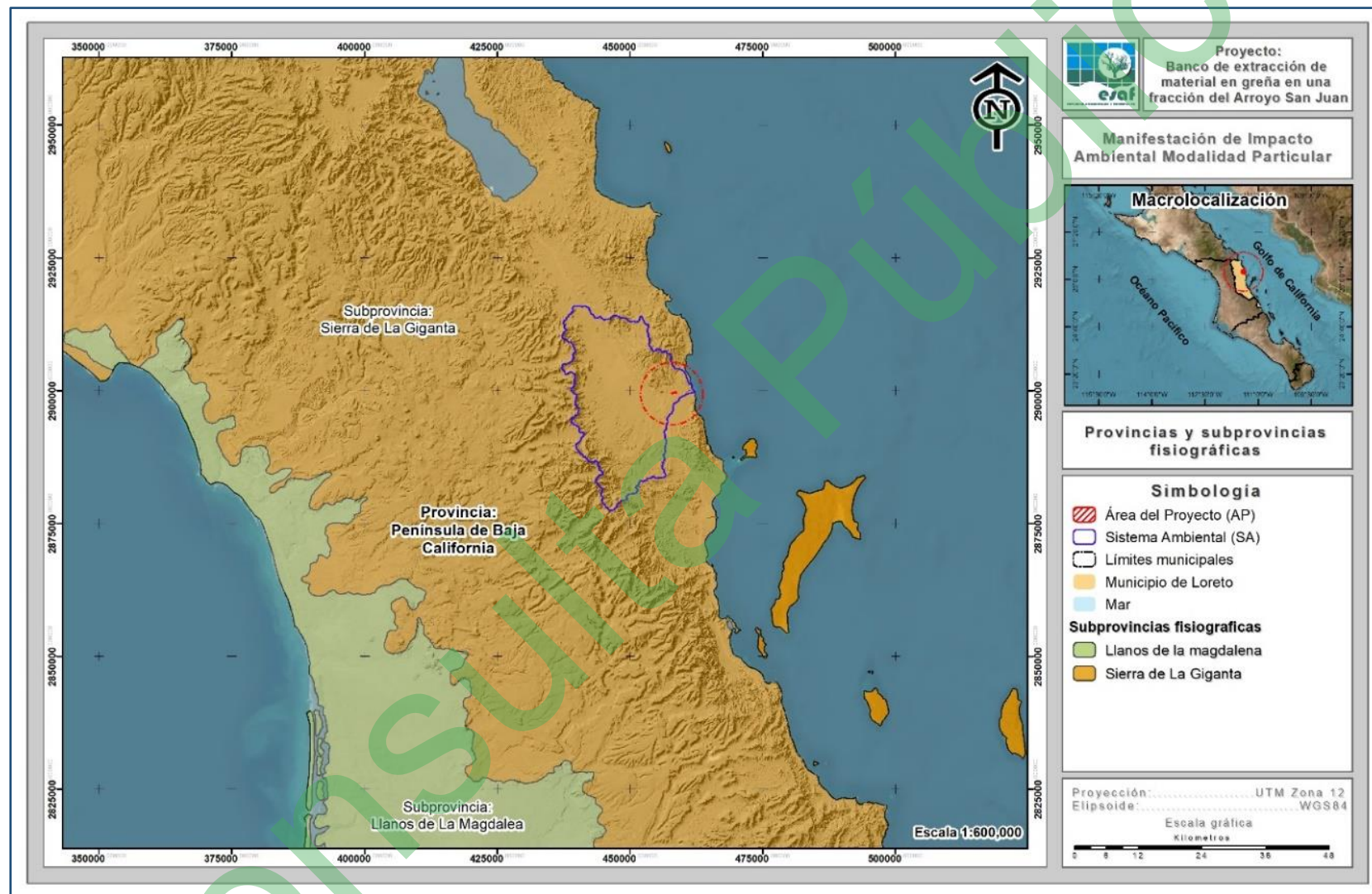
Figura IV-6. Clasificación fisiográfica del SA donde se ubica el proyecto.
