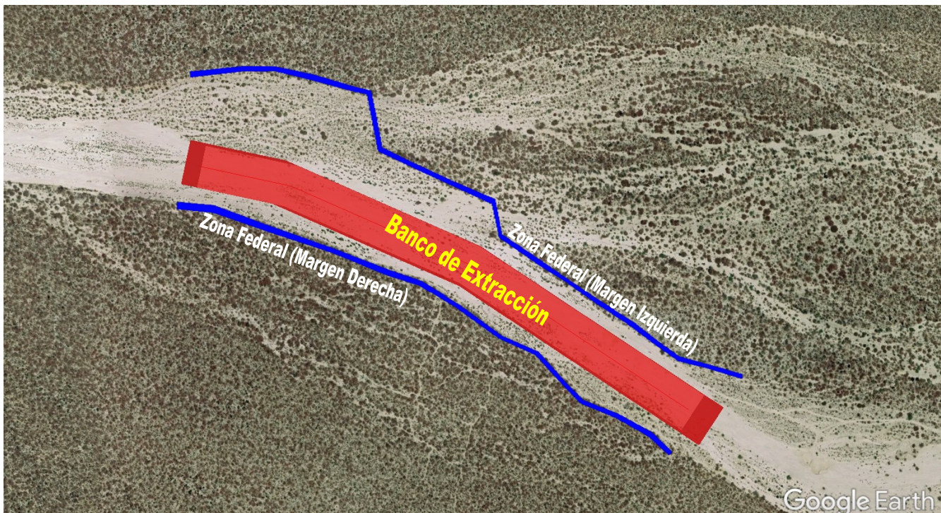
Figura 5.- Planta topográfica mostrando las dimensiones del proyecto pretendido de Banco de Extracción de Materiales en una fracción del cauce federal del Arroyo Agua Fría.
