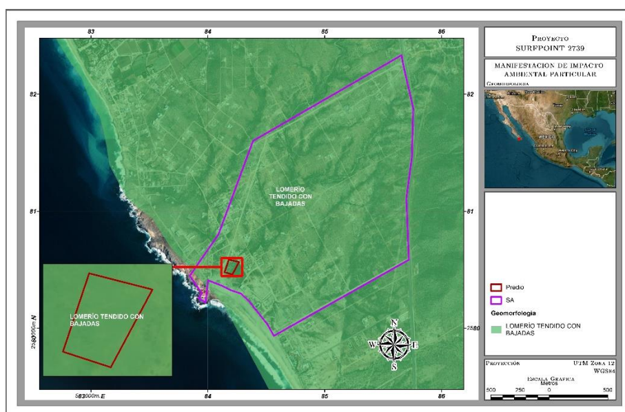
Figura 34.- Geomorfología SA y Proyecto.
