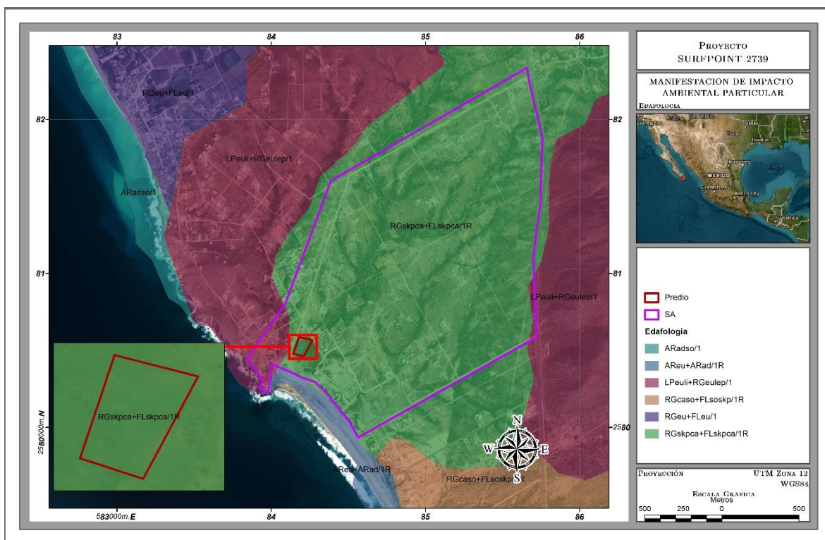
Figura 35.- Suelos en el SA y Proyecto.
