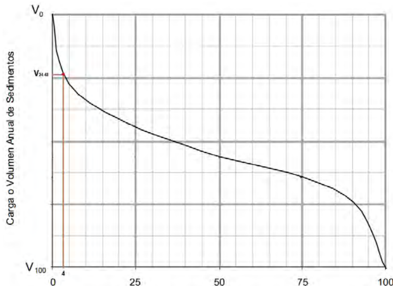
Figura 4. Curva de duración de la carga de fondo anual de un río.
