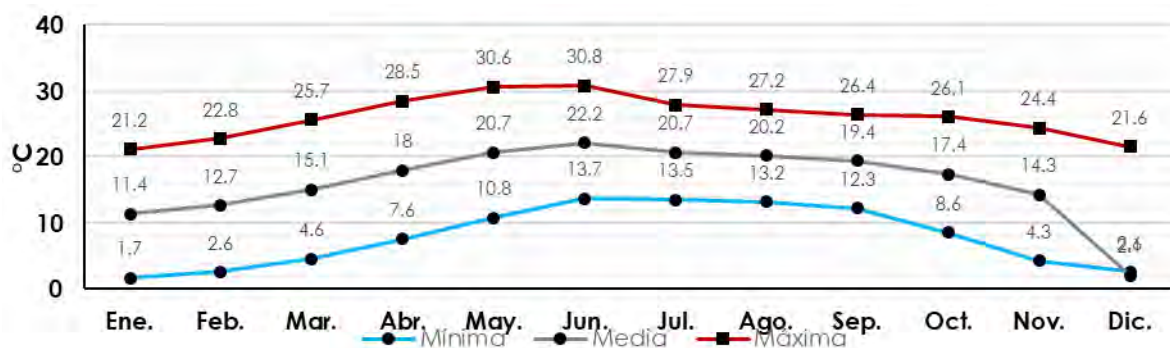
Gráfica 1. Climograma representativo de la estación meteorológica 10047 Narciso Mendoza.
