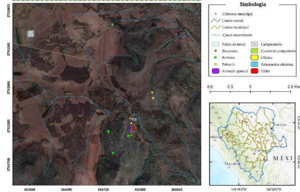
Figura Error: no se encontró el origen de la referencia-2. Localización de la infraestructura
