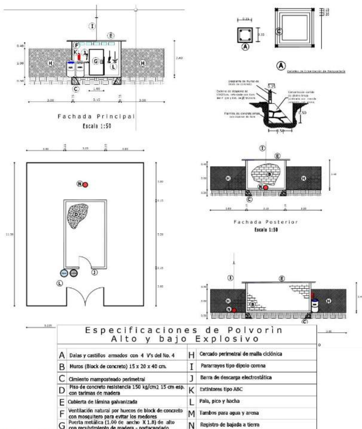
Figura Error: no se encontró el origen de la referencia-5. Detalles de la nave de los polvorines
