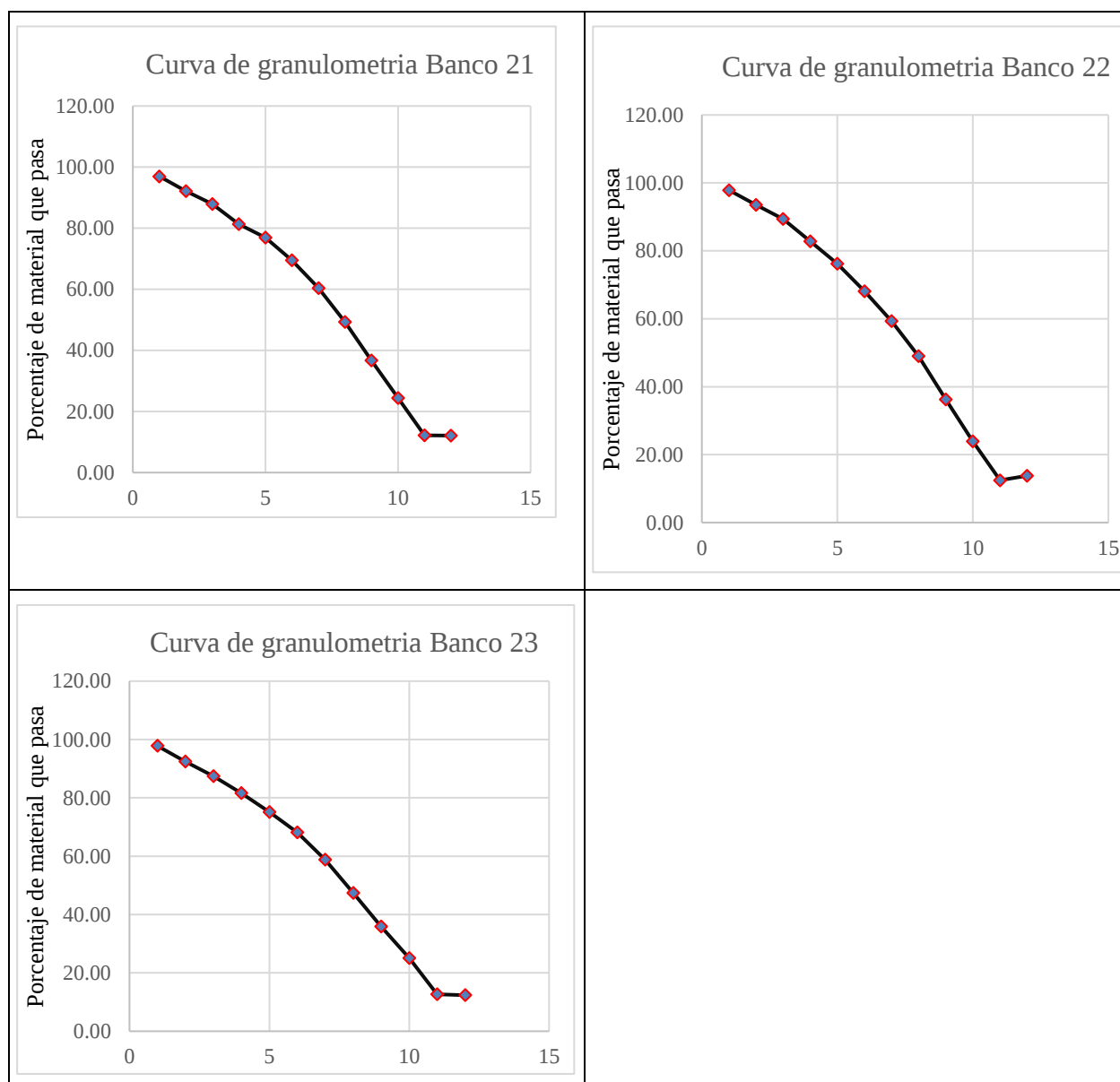
Ilustración VI: Gráficas granulométricas.
