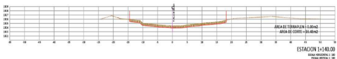
Figura Error: no se encontró el origen de la referencia-37. Sección transversal con levantamiento topográfico
