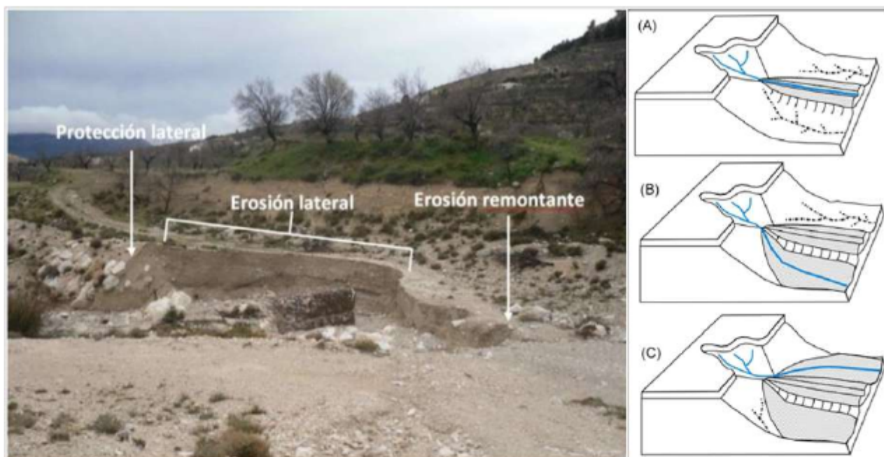
Figura Error: no se encontró el origen de la referencia-55. Fenómeno de erosión remontante y progresiva por extracción de materiales de arrastre en ríos
