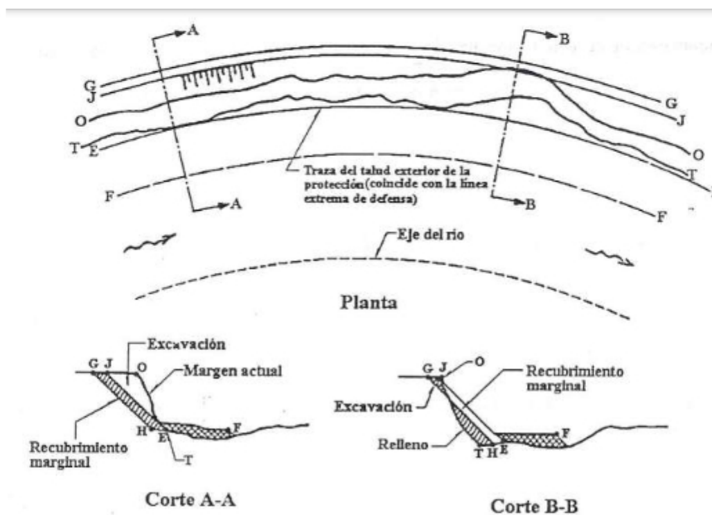
Figura Error: no se encontró el origen de la referencia-56. Trazo de recubrimiento marginal o suavización de taludes
