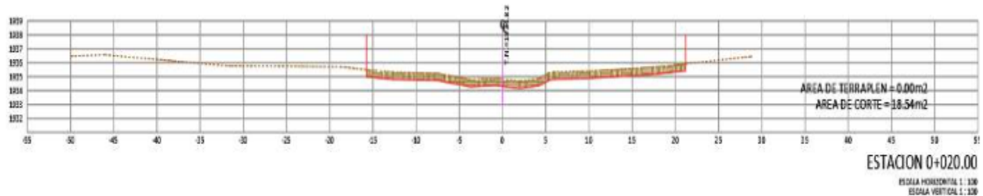
Figura Error: no se encontró el origen de la referencia-6. Sección transversal del cadenamiento 0+020 Banco La Cañadita
