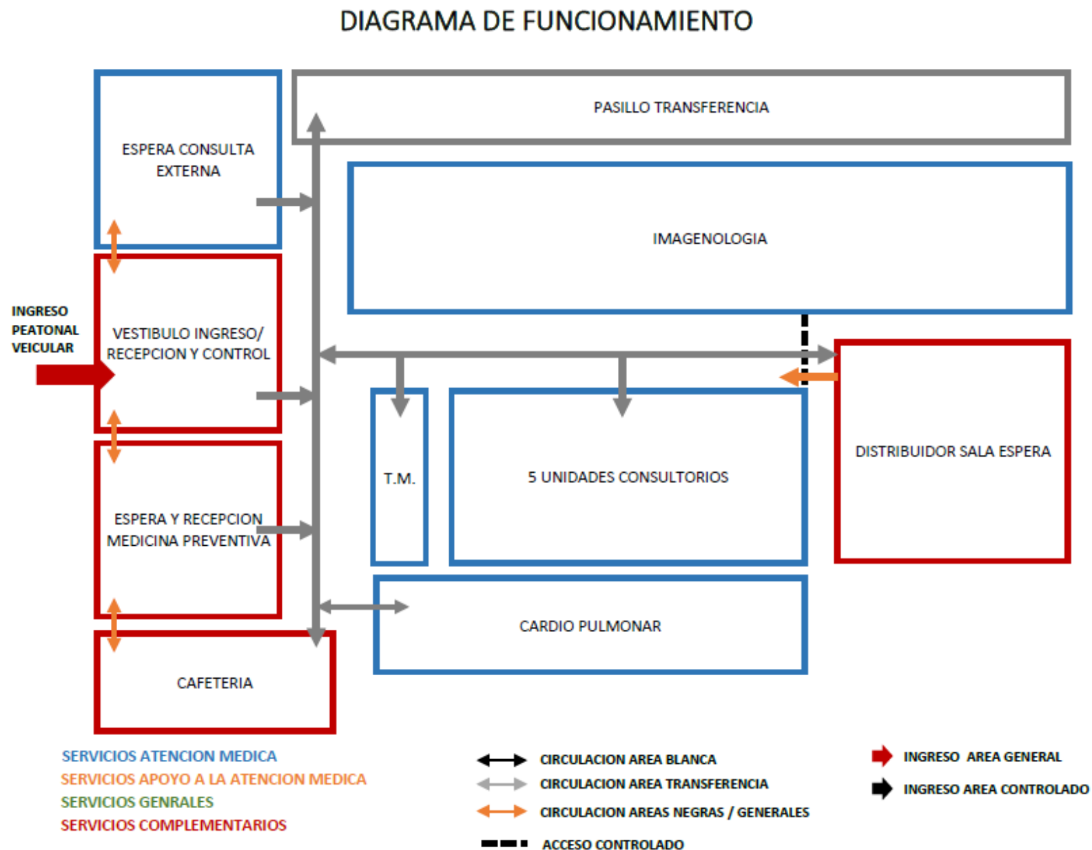
Figura 27.- Diagrama de funcionamiento de consulta externa y chequeos.
