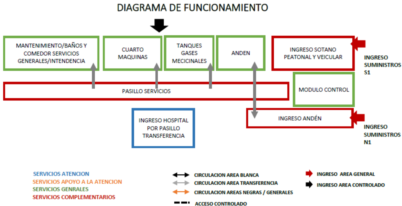
Figura 28.- Diagrama de funcionamiento de Servicios Generales.
