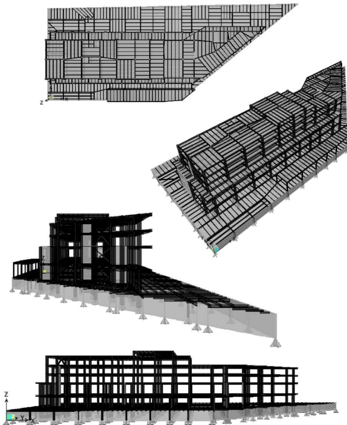
Figura 20.- Modelo matemático de superestructura.
