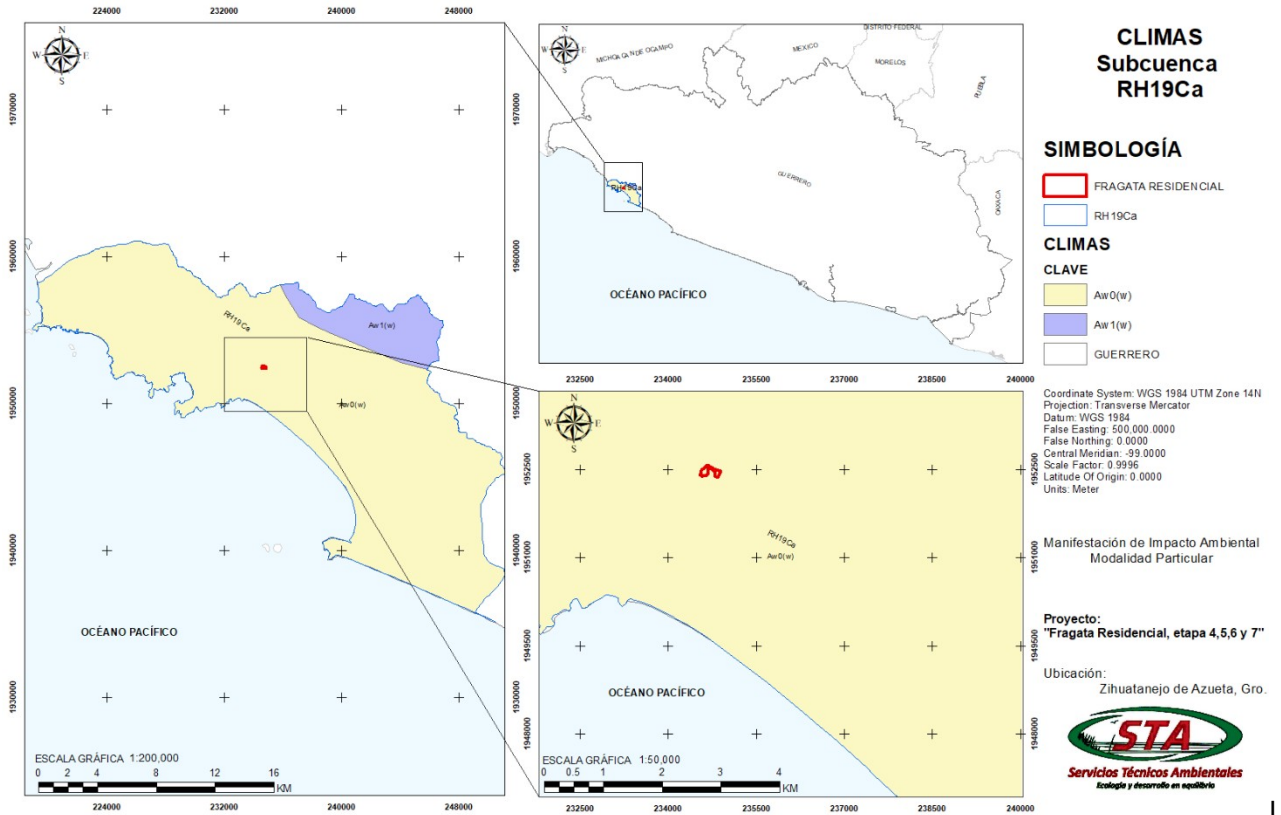
magen 18. Muestra el tipo de clima predominante sobre el área de influencia del proyecto. Fuente: www.inegi.gob.mx
