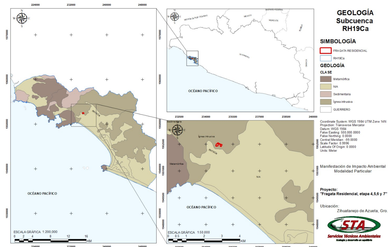
Imagen 19. Muestra el relieve para el área de influencia del proyecto, el cual corresponde a ígnea intrusiva. Fuente: www.inegi.gob.mx
