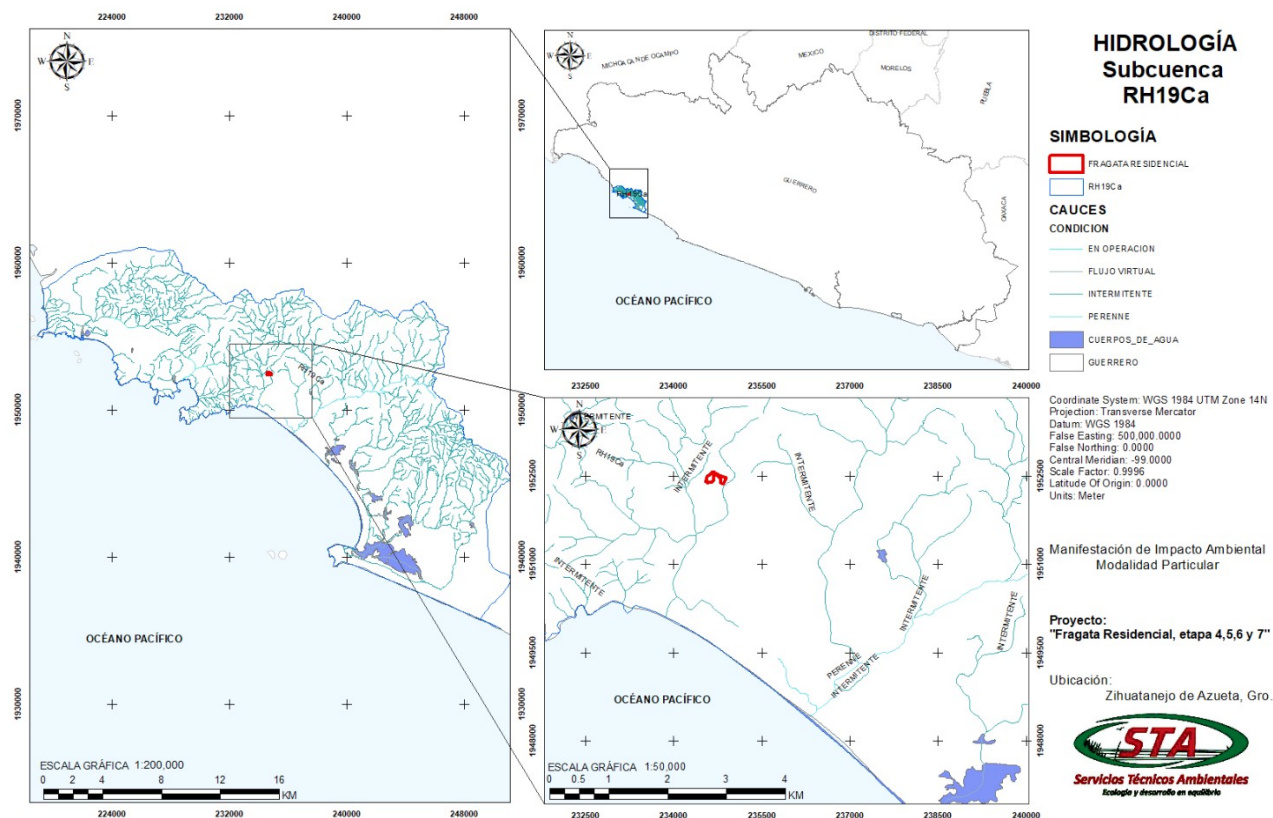
Imagen 21. Ubicación del proyecto en torno a las pendientes de corriente. Fuente: Atlas de riesgo del Municipio de Zihuatanejo.
