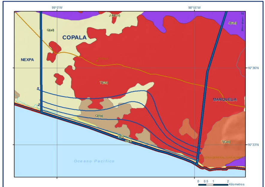
Fig.14. Profundidad al nivel estático en m (2011). Fuente: CONAGUA.
