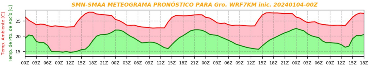
Figura 5. - Meteograma de la variable temperatura del Municipio de Copala.
