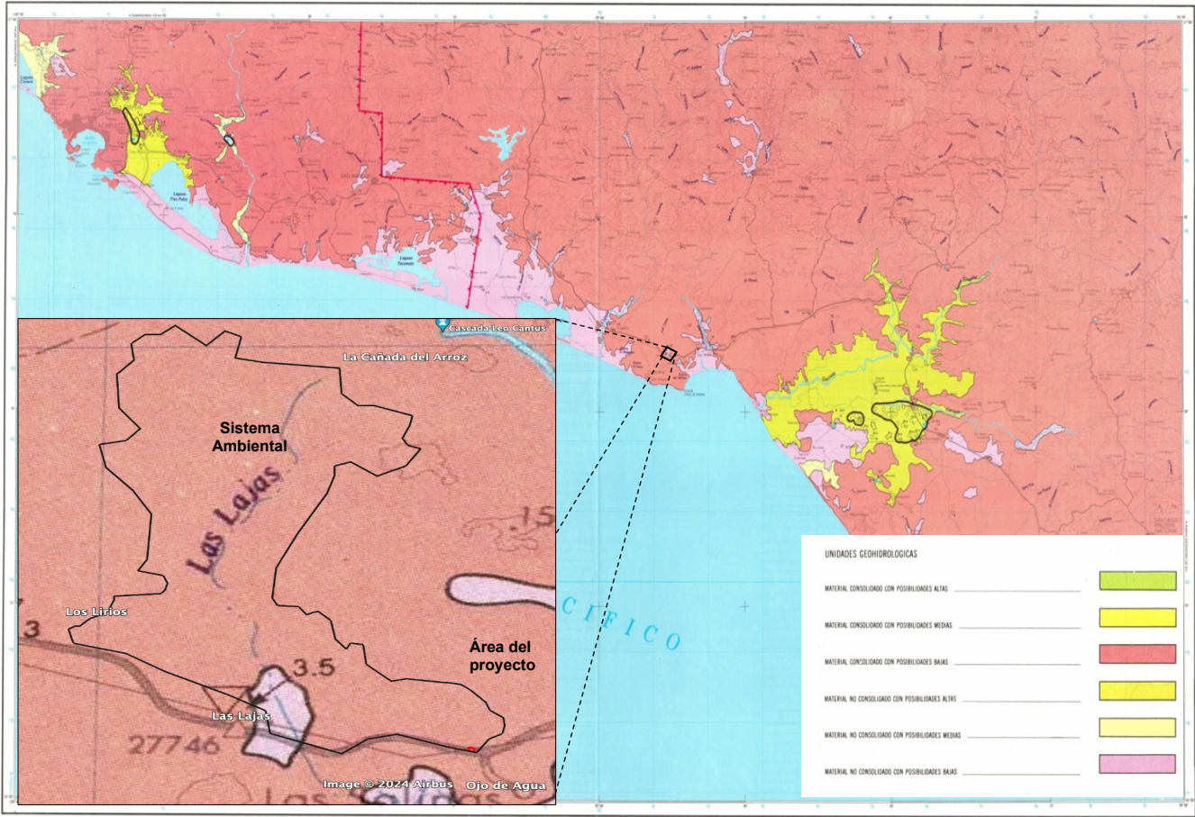
Mapa hidrológico de aguas subterráneas en el Sistema Ambiental y el área del proyecto.
