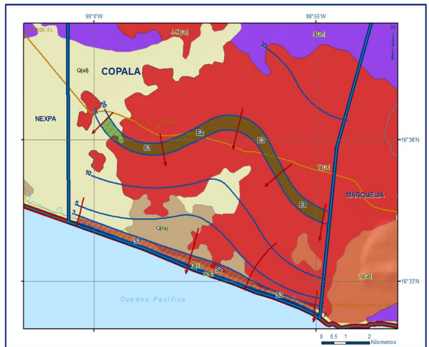
Fig.15. Elevación del nivel estático en msnm (2011) Fuente: CONAGUA.
