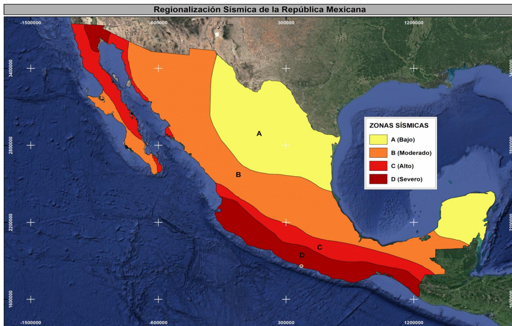
Fig.10. Regionalización Sísmica de la República Mexicana.
