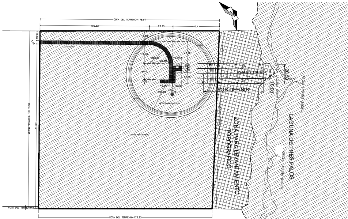
Ilustración 2 PLANTA ARQUITECTONICA Y SECCIONES TIPO DEL MUELLE
