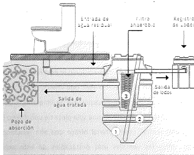
Figura 2. Componentes del Biodigestor
