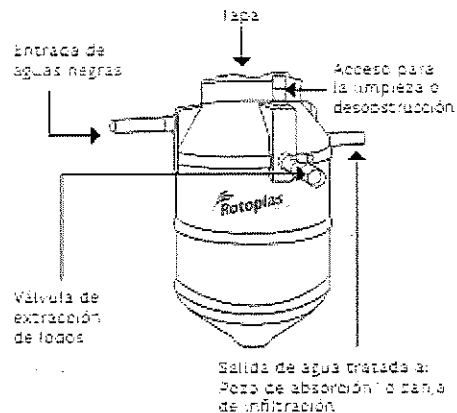
Figura 2. Componentes del Biodigestor
