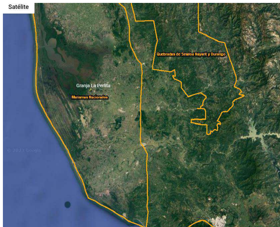
Uso actual de suelo en el sitio del proyecto.
