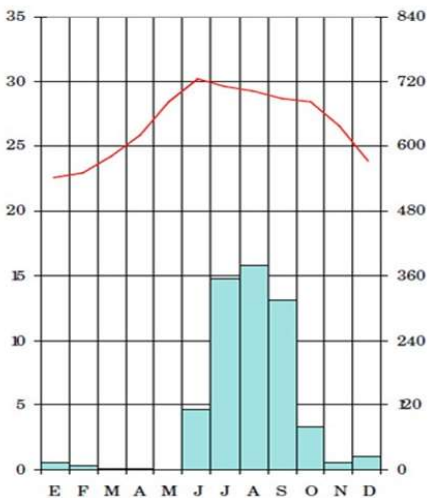
Climograma de la Estación Meteorológica 18-001 Acaponeta, Nayarit
